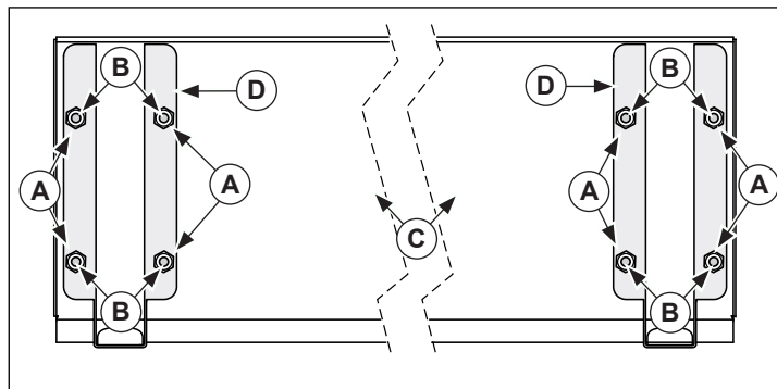
Figura 3. Instalación del posaplatos y los soportes
