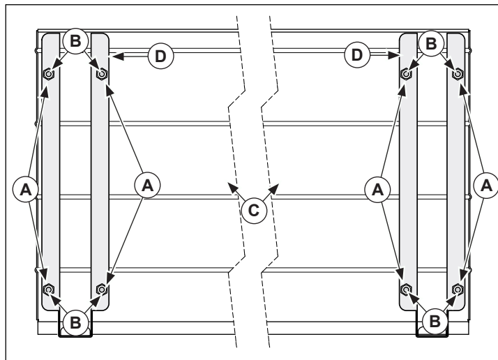
Figure 4. Installation de la glissière à plateaux et des supports
