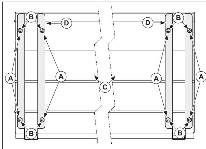
Figura 4. Instalación del deslizador de bandejas y los soportes
