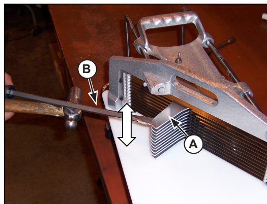
Figure 1. Ajustement de la tête de poussée entre les lames
