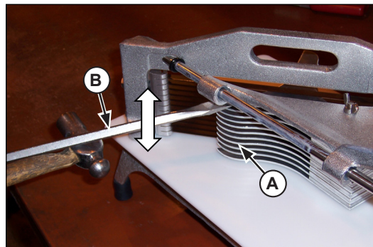
Figure 2. Ajustement de la tête de poussée entre les lames
