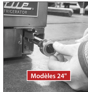
Fig. 1. Les modèles 24 et 27 utilisent différentes charnières inférieures.
