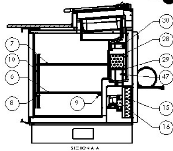
SECCION A-A
