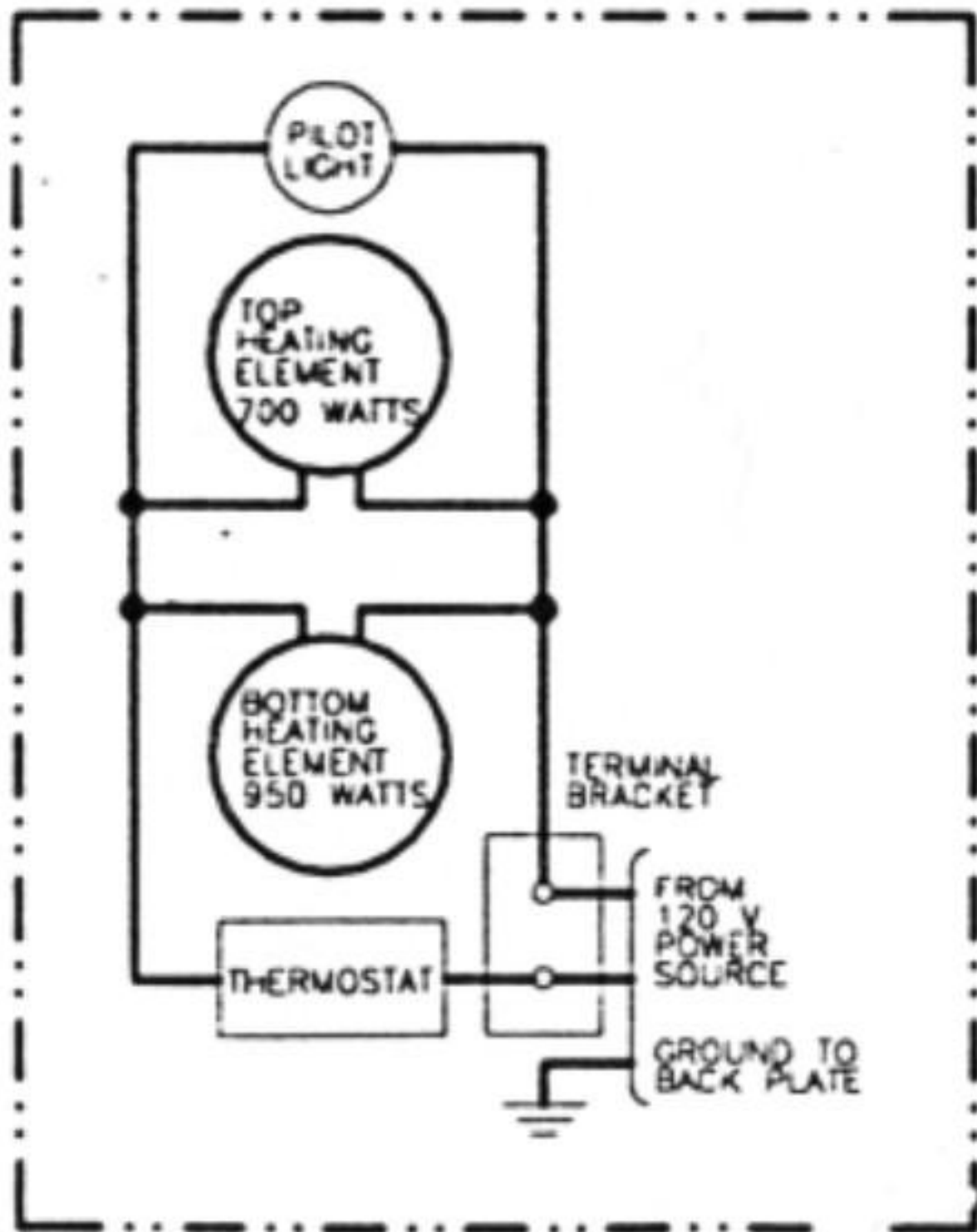
WIRING DIAGRAMS
