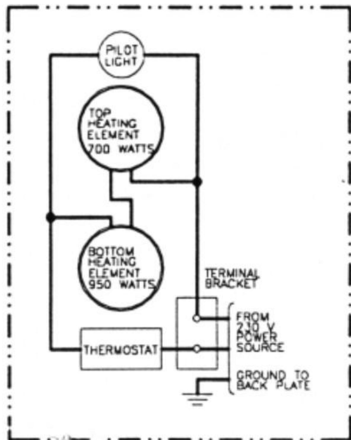
WIRING DIAGRAMS
