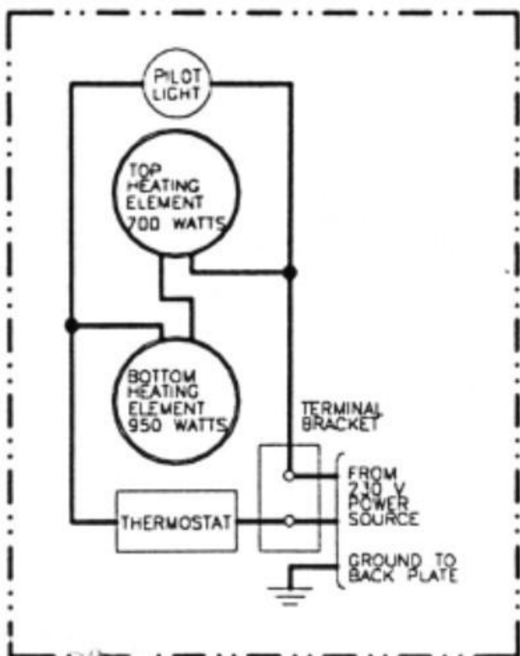
WIRING DIAGRAMS
