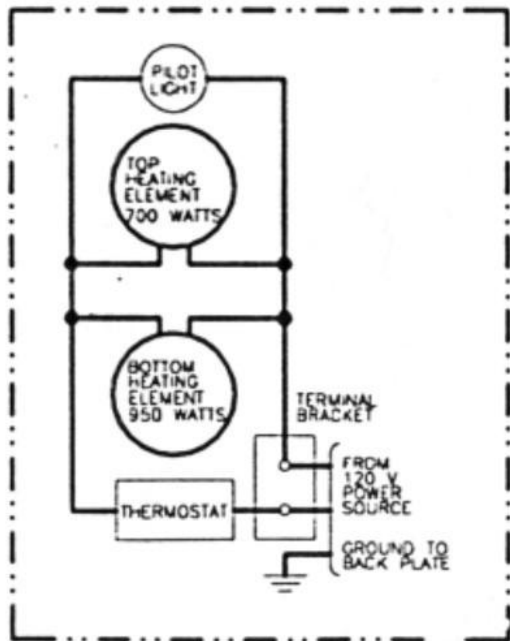
WIRING DIAGRAMS
