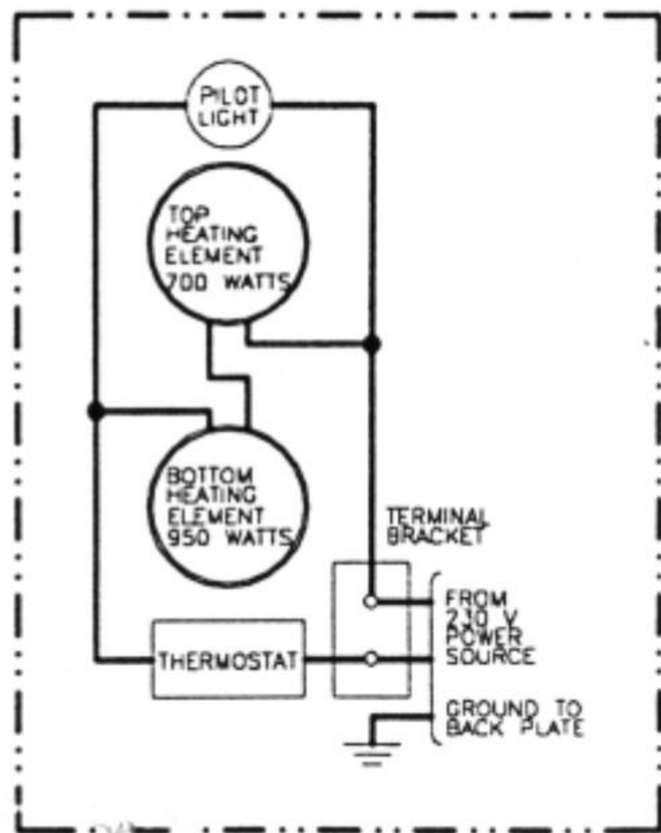
WIRING DIAGRAMS
