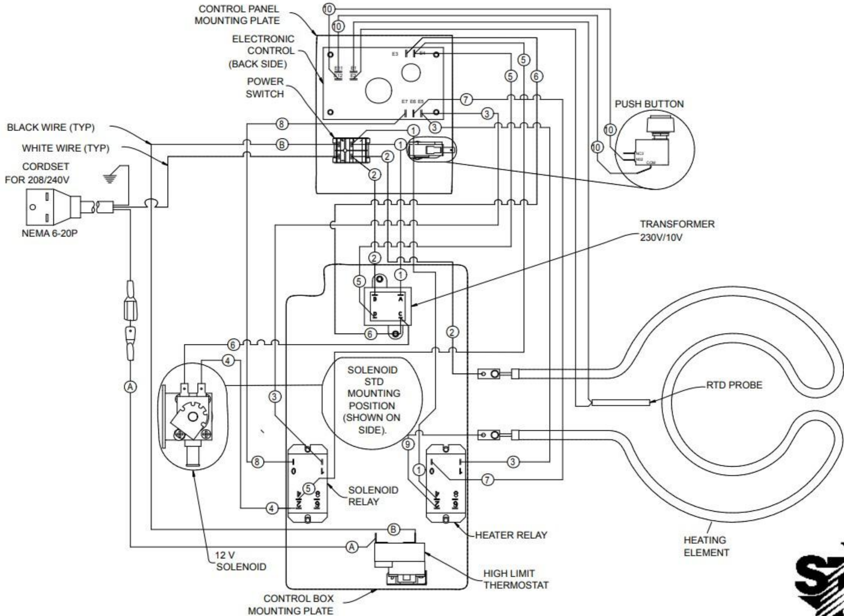
WIRING DIAGRAM FSFDT
