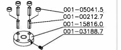
Acoplamiento Completo 001-15815.1
