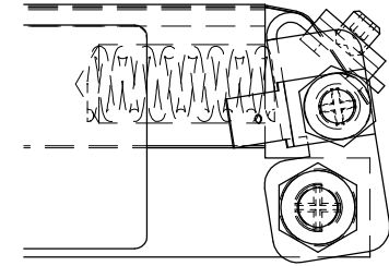
-DÉTAIL A-
