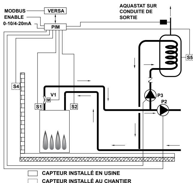
Figure 30. Mode 2 - Chaudière unique avec chauffe-eau indirect - boucle primaire
