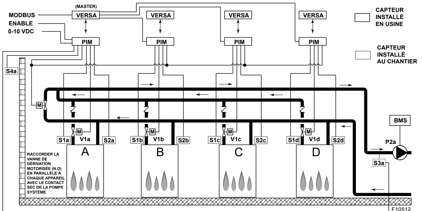
Figure 28. Cascade de chaudières avec vanne de dérivation motorisée
