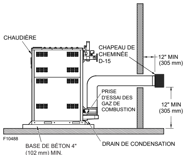
Figure 48. Acier inoxydable et polypropylène - Ventilation directe murale à l'horizontale
