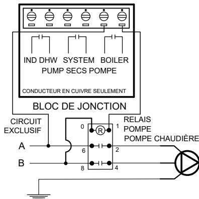
Figure 44. Câblage de la pompe de chaudière
