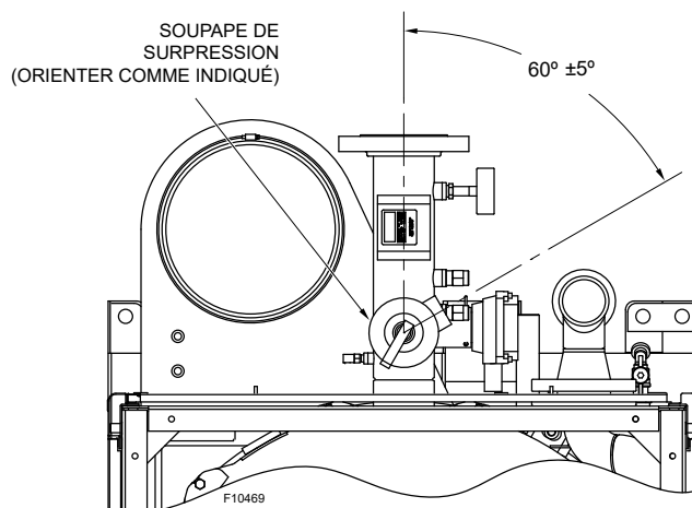
Figure 17. Orientation recommandée de la soupape
