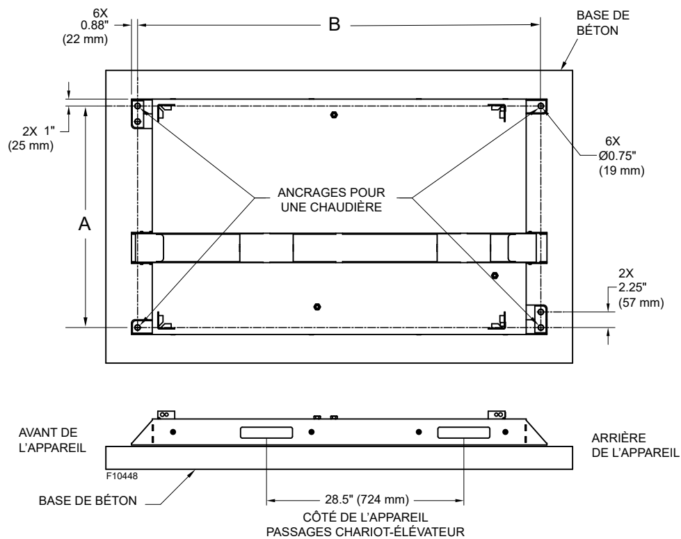
Figure 5. Ancrage pour un appareil
