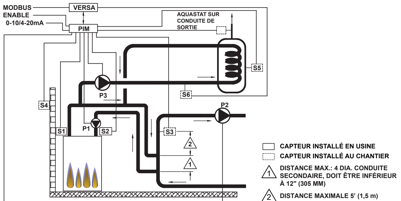
Figure 24. Mode 3 - Chaudière unique avec chauffe-eau indirect sur boucle primaire - boucles prim./sec.
