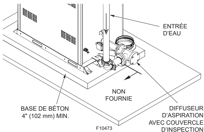
Figure 15. Diffuseur d'aspiration (débit laminaire)
