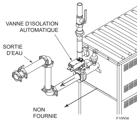
Figure 60. Installation de la vanne d'isolement automatique
