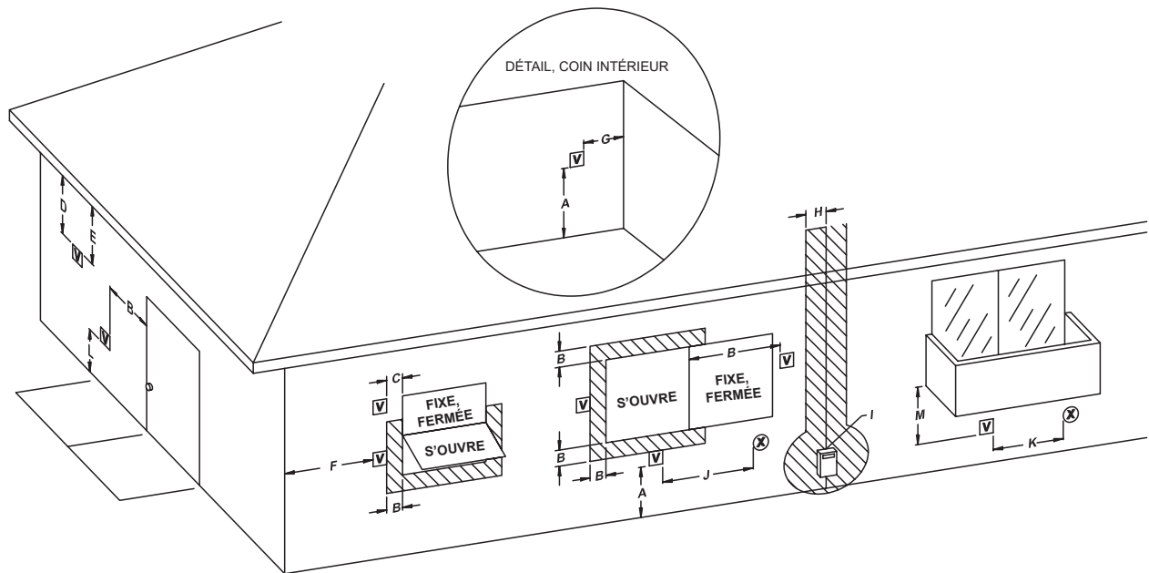
Figure 11. Dégagements minimum aux matières combustibles, terminaisons d'apport d'air et d'évacuation – Installation intérieure ou extérieure
