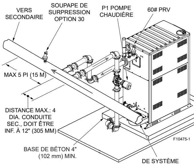
Figure 20. Boucles primaire/secondaire hydriques
