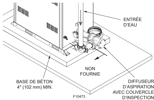
Figure 58. Diffuseur d'aspiration (débit laminaire)
