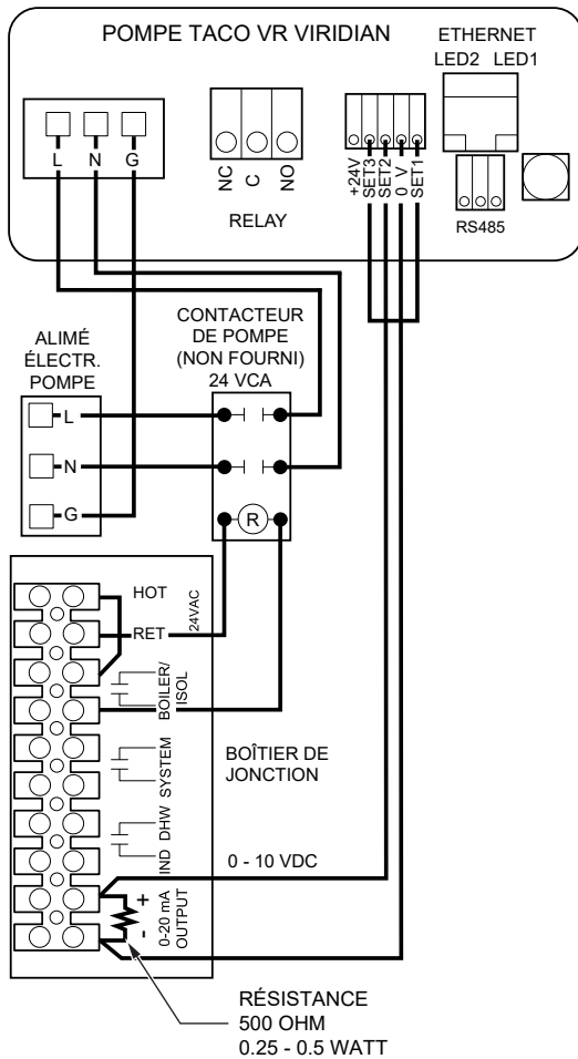
Figure 43. Schéma de câblage, pompe VS
