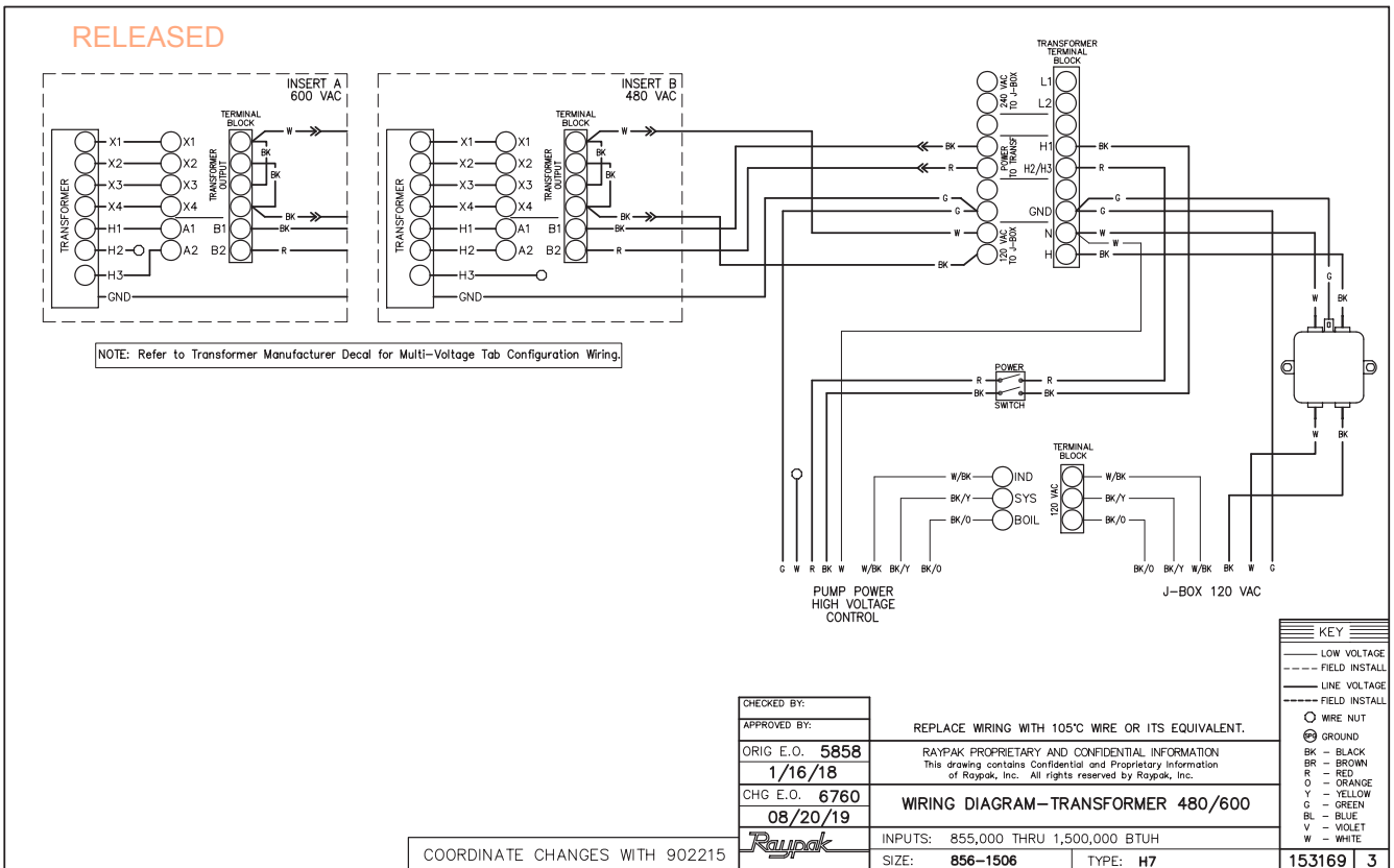
Figure 38. Schéma de câblage transformateur 480/600 VAC pour modèles 0856-1506
