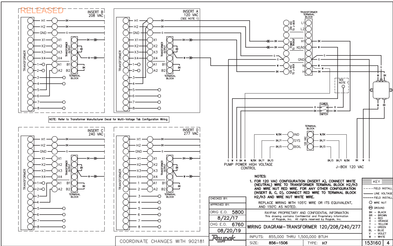
Figure 37. Schéma de câblage transformateur 120/208/240/277 VAC for Models 0856-1506
