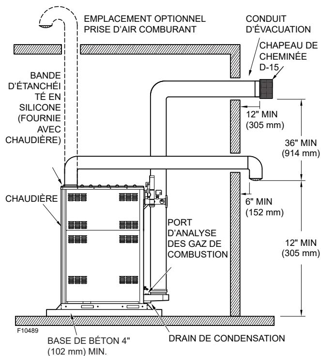
Figure 49. Acier inoxydable et polypropylène - Ventilation directe à l'horizontale
