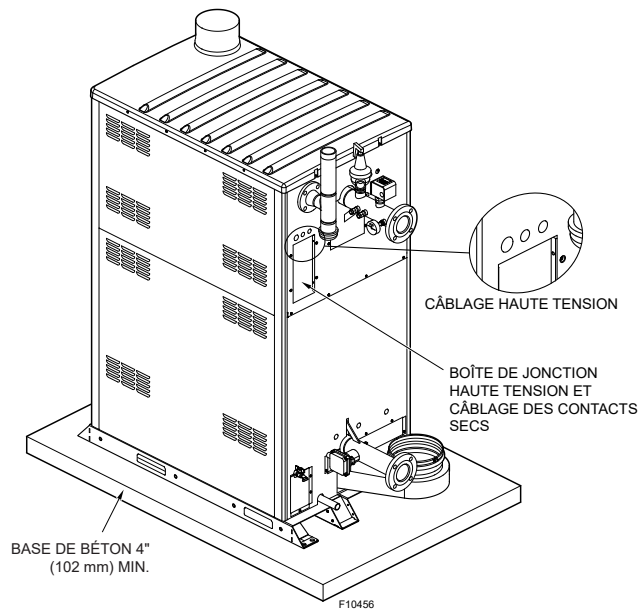
Figure 32. Emplacement boîte de jonction arrière
