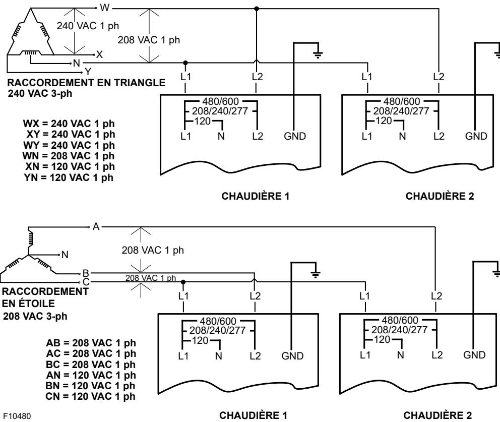
Figure 34. Raccordements électriques en triangle et en étoile 120/208/240 VCA
