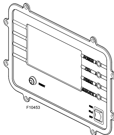
Figure 71. Interface-utilisateur
