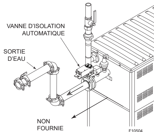
Figure 16. Installation de la vanne d'isolation motorisée
