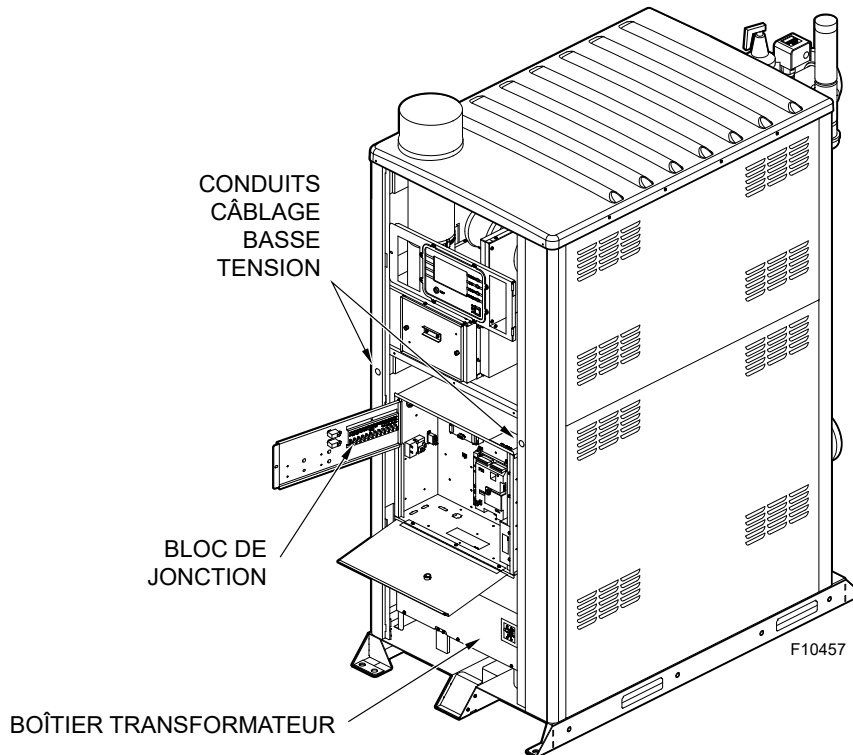
Figure 42. Boîtier de jonction basse tension
