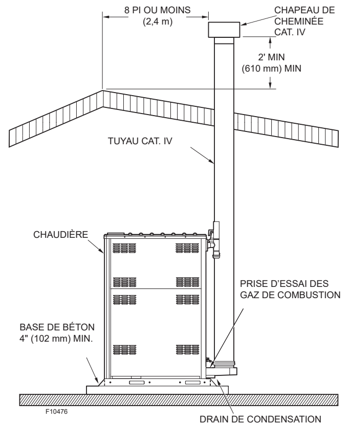
Figure 46. Acier inoxydable et polypropylène - Ventilation verticale
