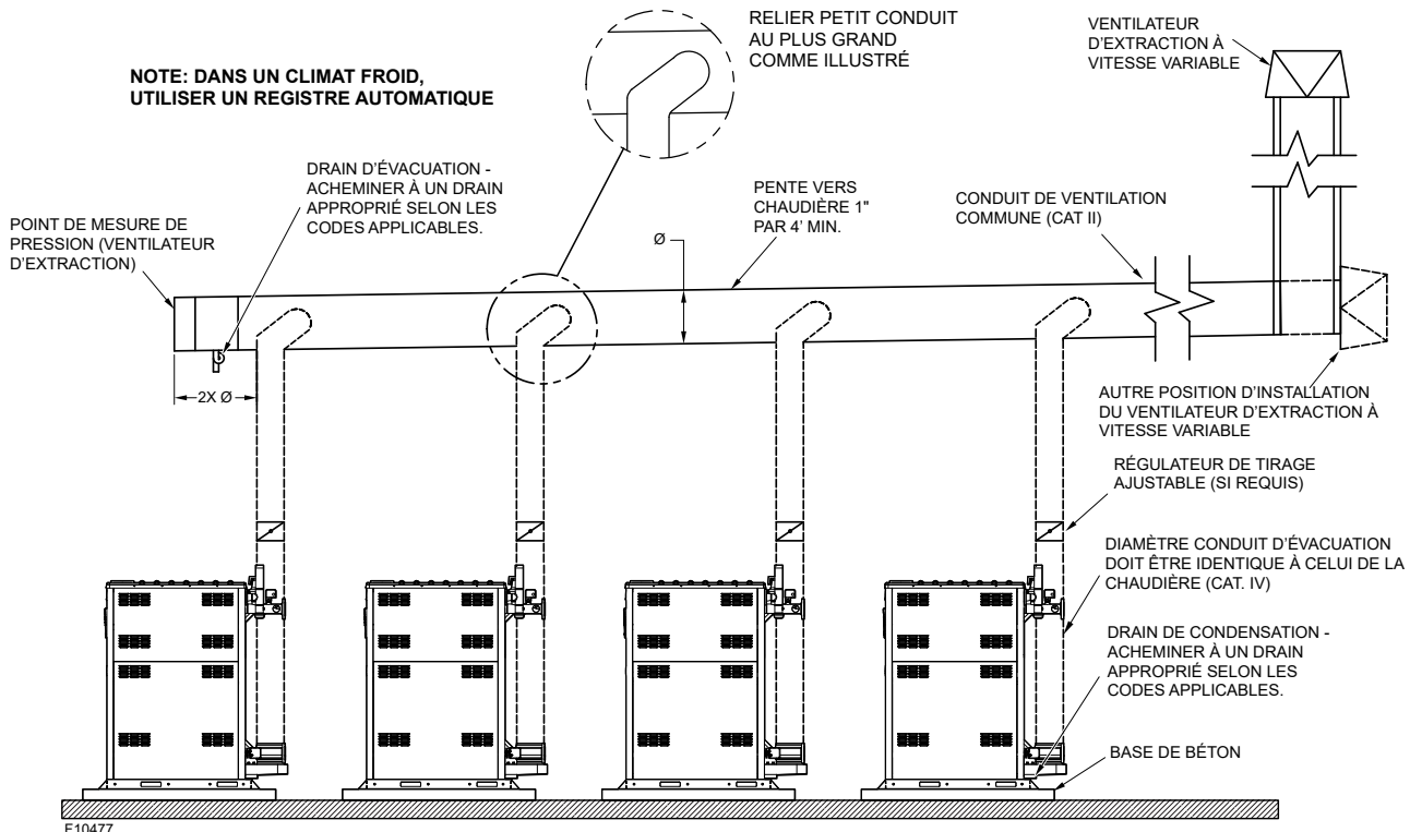
Figure 56. Ventilation commune typique
