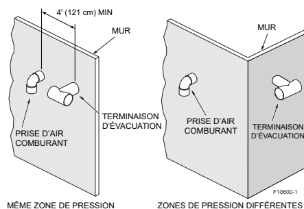
Figure 50. Emplacement apport d'air
