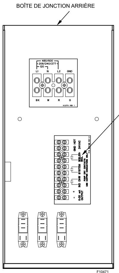
Figure 33. Raccordements électriques
