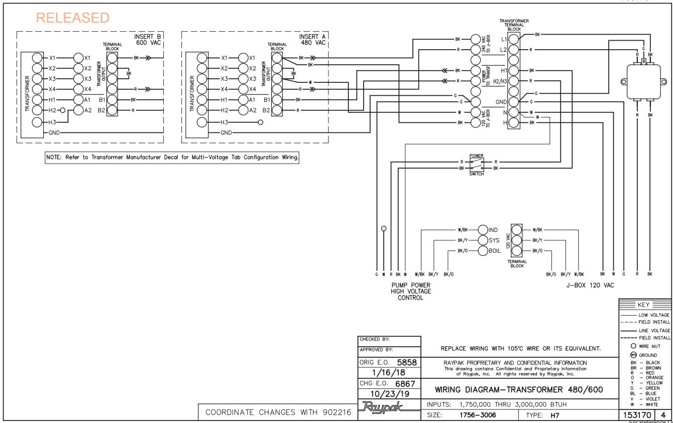
Figure 40. Schéma de câblage transformateur 480/600 VAC pour modèles 1756-3006
