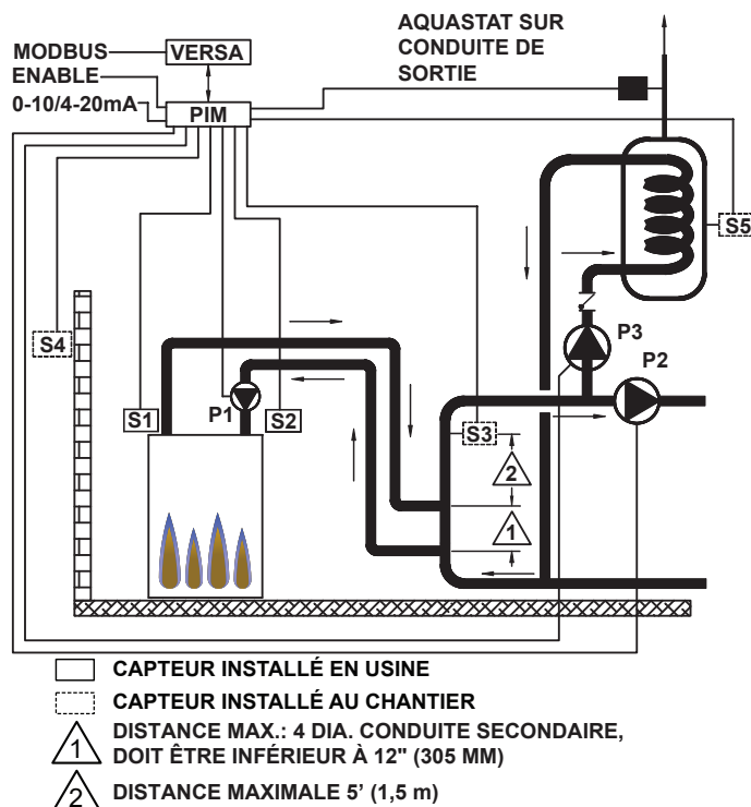
Figure 23. Mode 2 - Chaudière unique avec chauffe-eau indirect sur boucle secondaire - boucles prim./sec.
