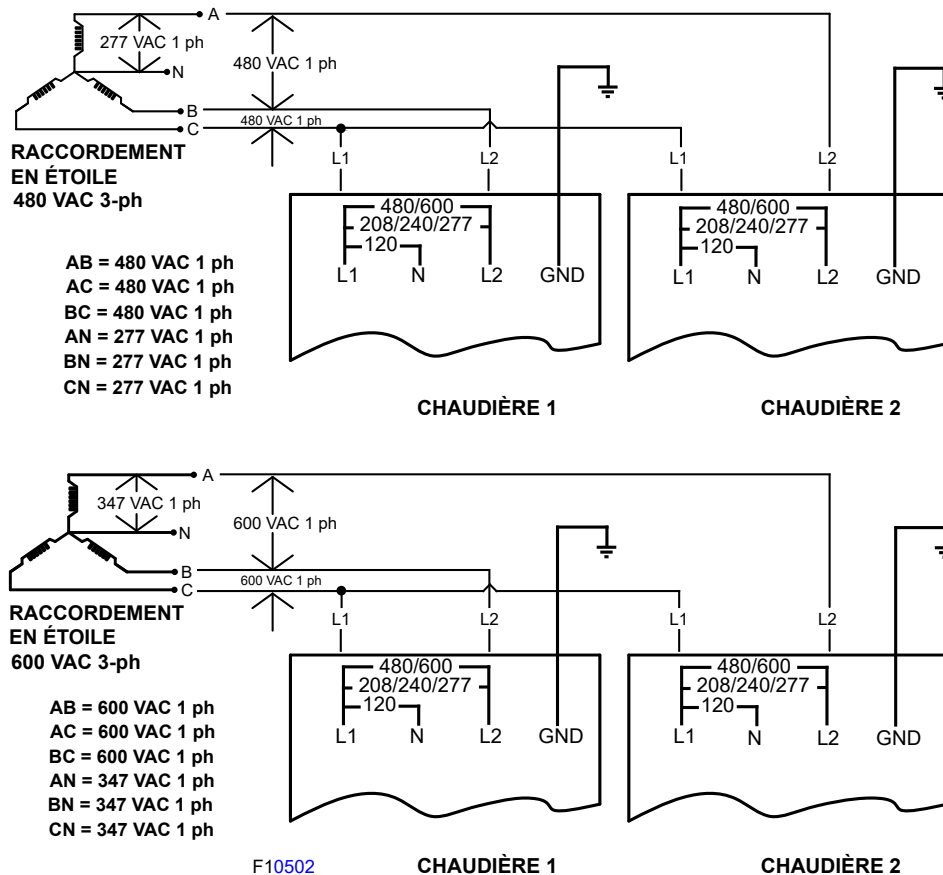
Figure 35. Raccordements électriques en étoile 277/480/600 VAC
