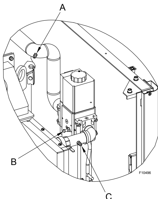
Figure 73. Emplacements de mesure de pression de gaz
