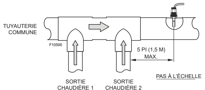
Figure 19. Installation de la sonde système, primaire système en cascade
