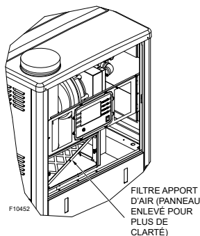
Figure 13. Position du filtre à air
