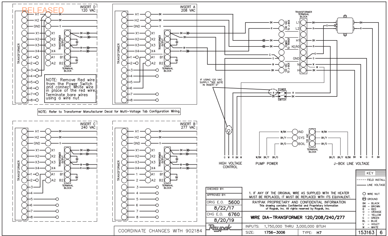
Figure 39. Schéma de câblage transformateur 208/240/277 VAC pour modèles 1756-3006
