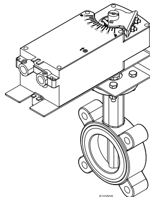
Figure 61. Vanne d'isolement automatique
