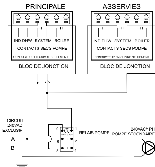
Figure 45. Pompes système en cascade XVers (240 VCA illustré)
