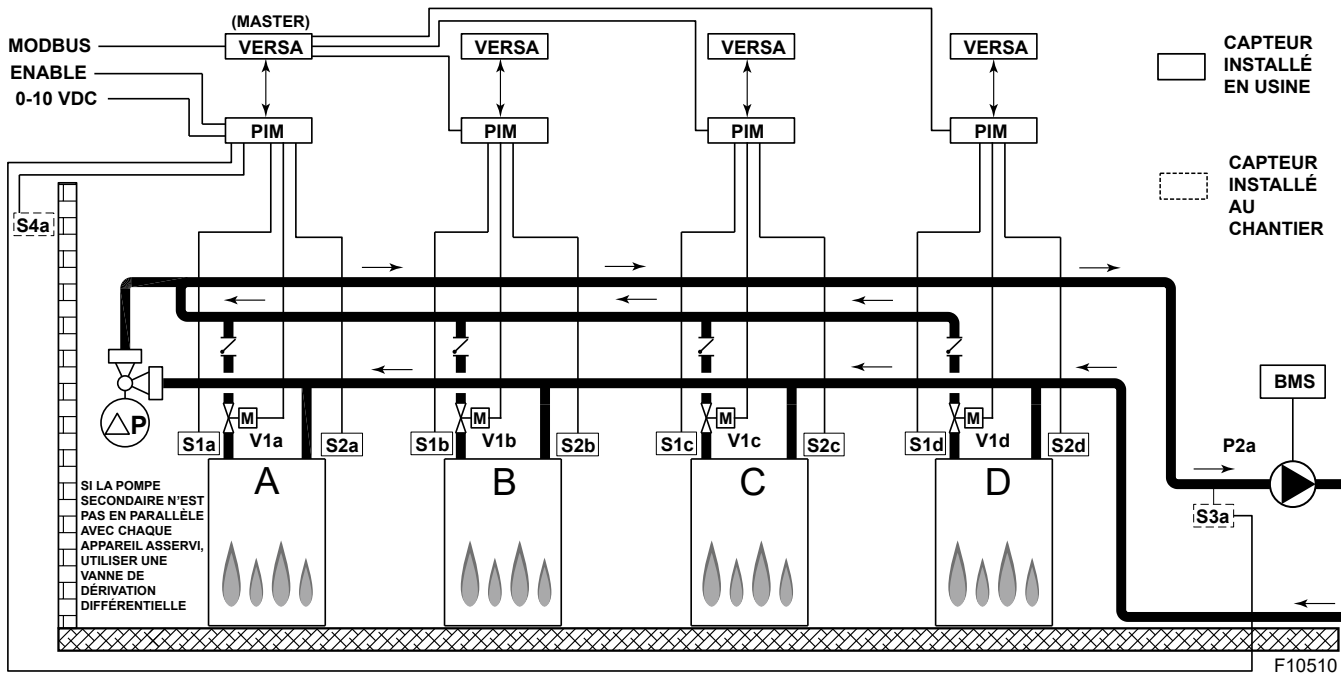
Figure 29. Cascade de chaudières avec vanne de dérivation à pression différentielle - boucle primaire
