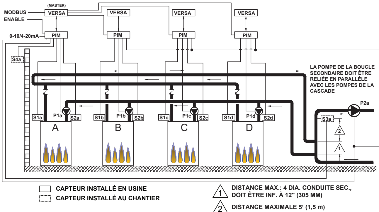
Figure 22. Mode 1 - Chaudières en cascade avec boucles primaire/secondaire
