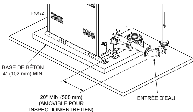
Figure 14. Exigence de tuyauterie
