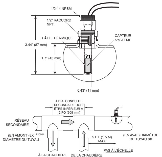
Figure 18. Installation de la sonde système, primaire/secondaire
