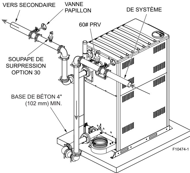
Figure 25. Tuyauterie primaire hydronique
