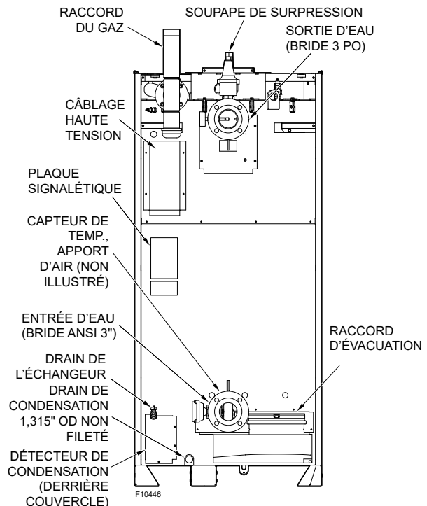
Figure 3. Position des pièces – Vue arrière
