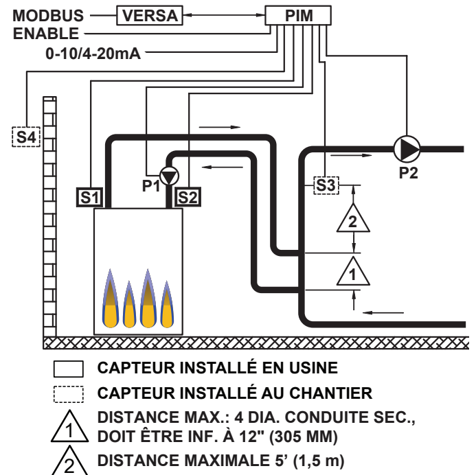
Figure 21. Mode 1 - Chaudière unique avec boucles primaire/secondaire
