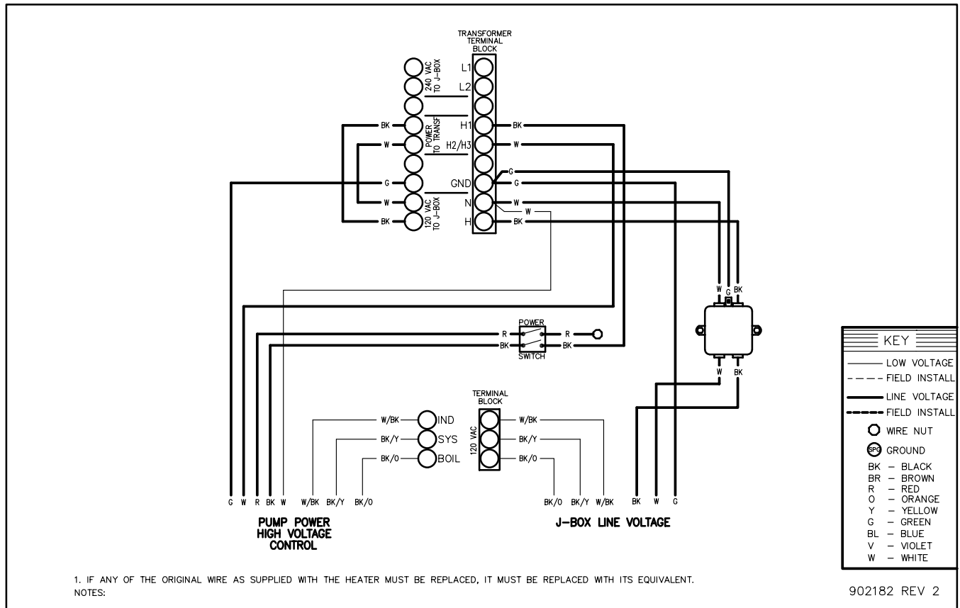
Figure 36. Schéma de câblage transformateur 120 VCA, de série sur 856-1506, en option sur 1756-3006
