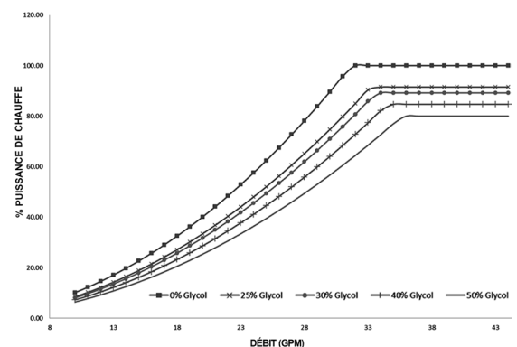
Figure 59. Graphique de fonctionnement au glycol
