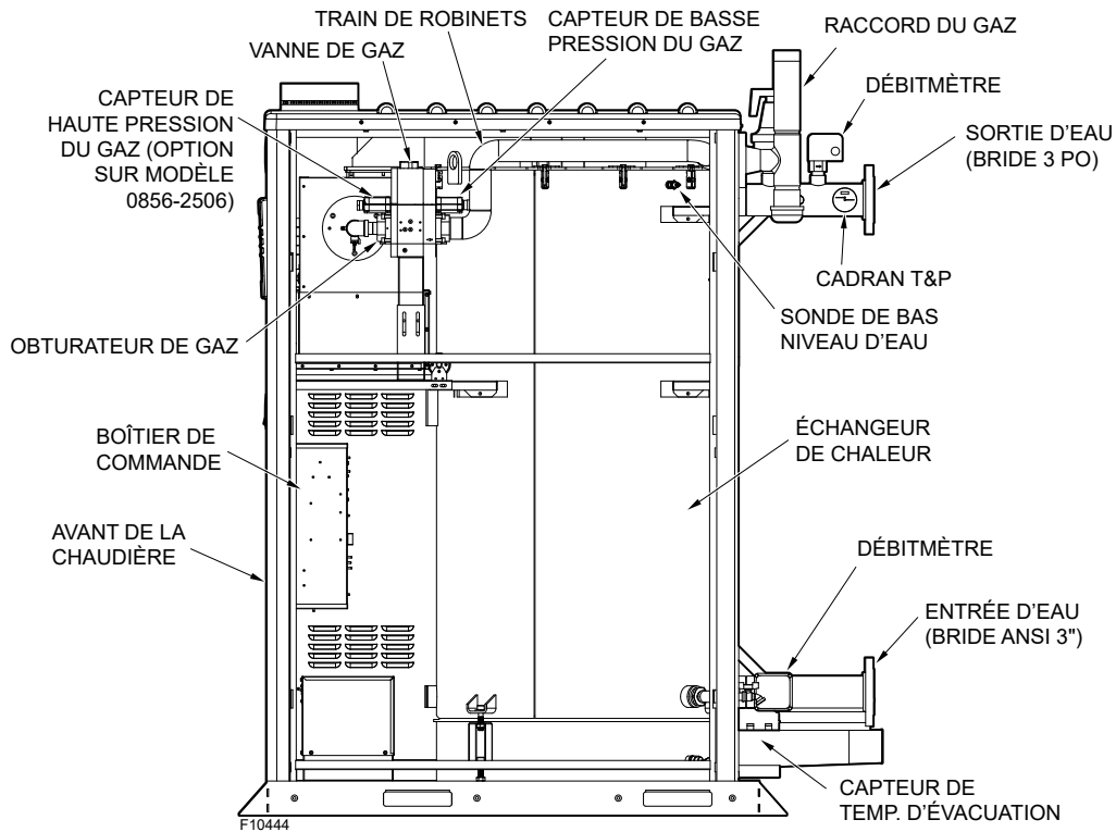
Figure 1. Position des pièces – Vue de droite
