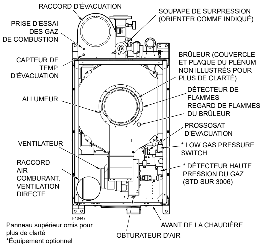
Figure 4. Position des pièces – Vue du dessus
