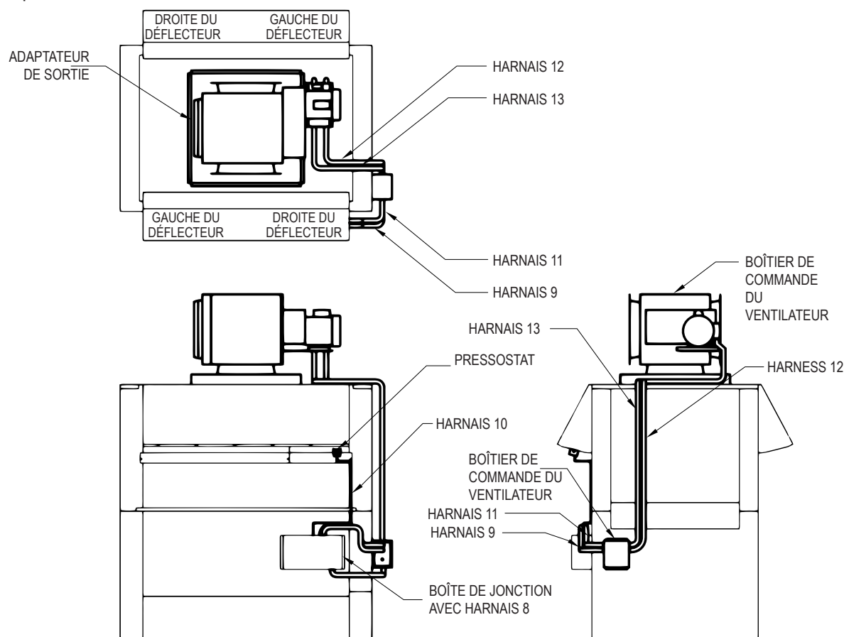
Figure 14. Raccordements, modèles 2100 à 4001
