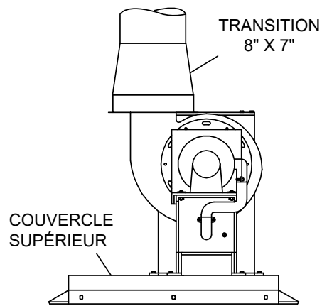
Figure 26. Transition d'évacuation, modèles 0514 à 1223
