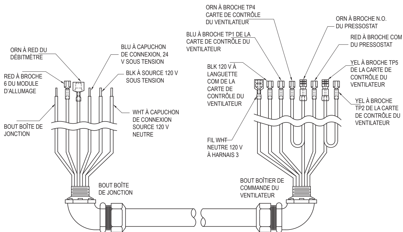
Figure 6. Harnais 2, modèles 0514 à 0824
