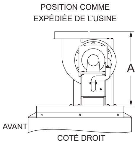
Figure 30. Ventilateur, position 1
