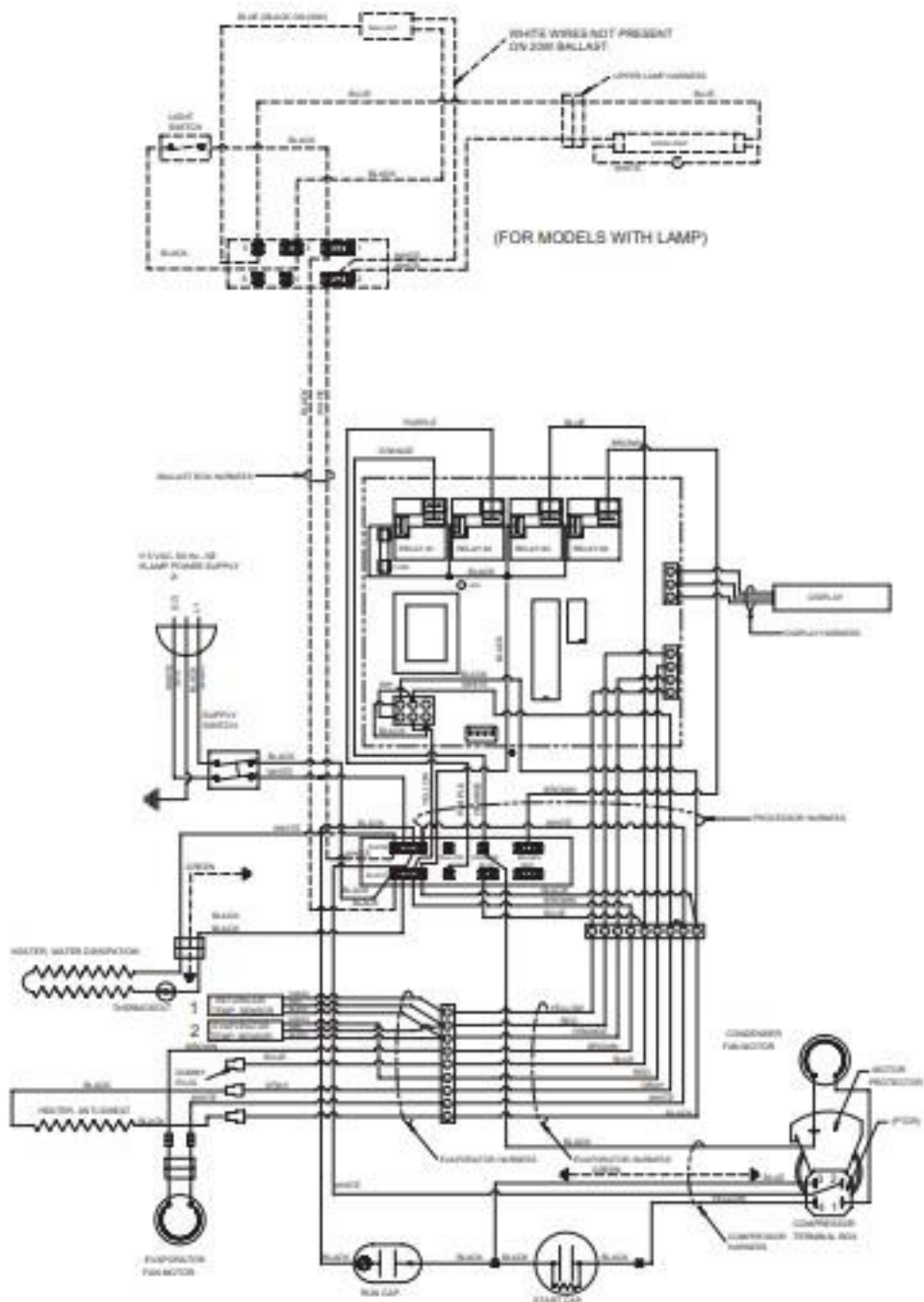
WIRING DIAGRAM-OPEN, MED-TEMP. 00-0219-00
