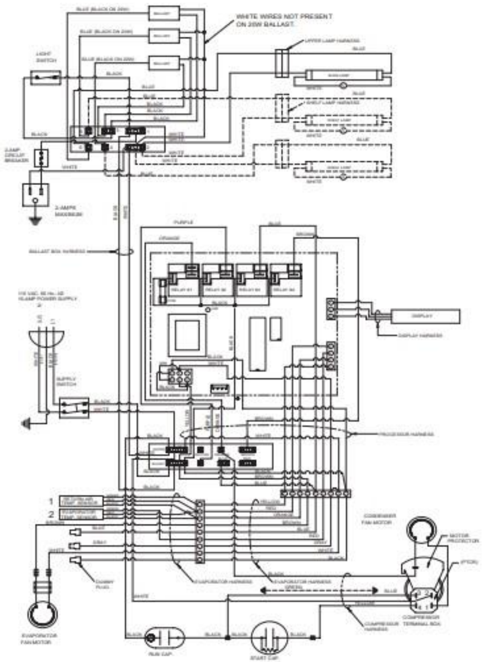
WIRING DIAGRAM-DISPLAY, MED-TEMP. 00-0217-00
