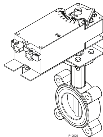
Figure 68. Vanne d'isolation automatique
