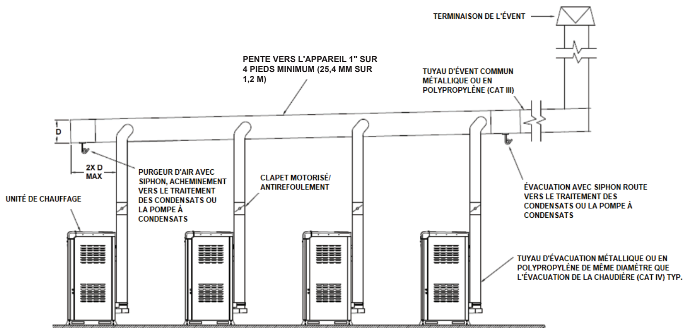
Figure 53. Événement commun à pression positive typique
