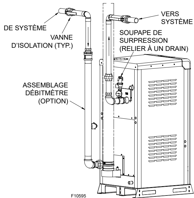
Figure 24. Tuyauterie primaire hydraulique
