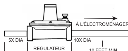
Figure 31. Distances de régulateur de gaz
