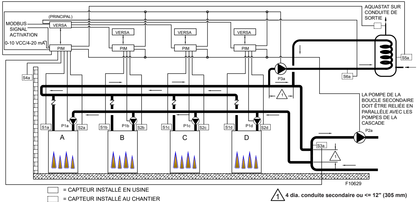
Figure 23. Mode 3 - Chaudières en cascade avec chauffe-eau indirect, boucle primaire/secondaire
