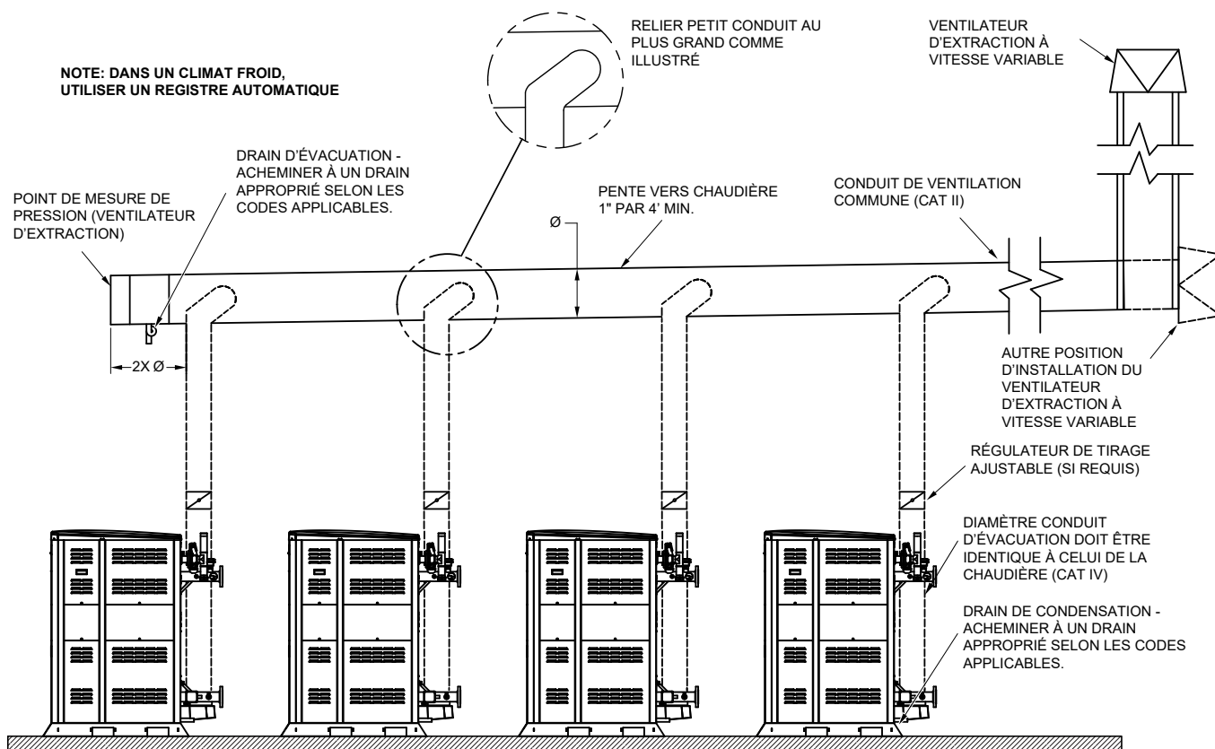
Figure 52. Événement commun à pression négative typique
