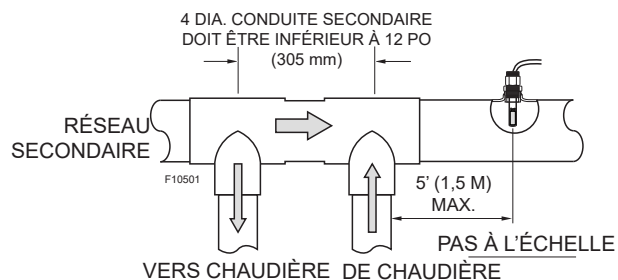
Figure 15. Installation de la sonde système, primaire/secondaire
