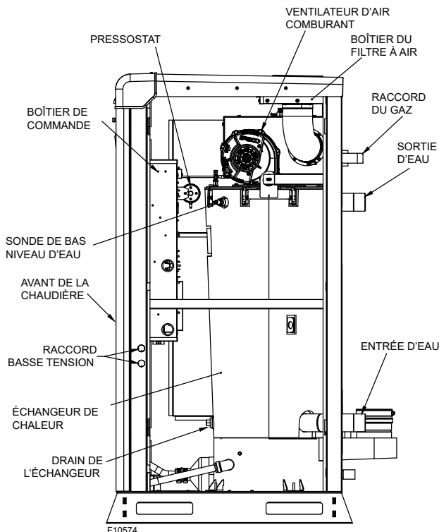
Figure 2. Position des pièces – Vue de côté
