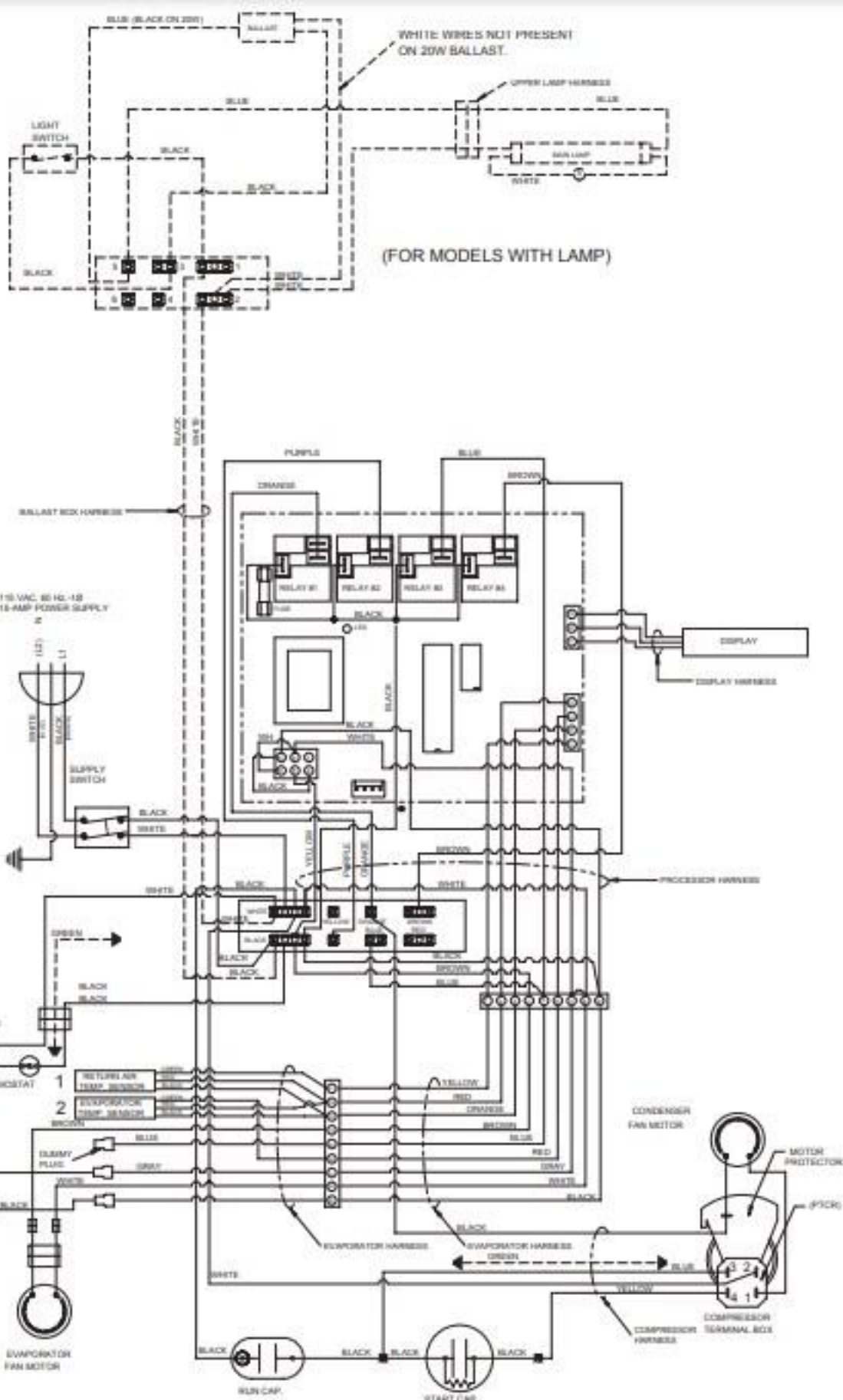
WIRING DIAGRAM-OPEN, MED-TEMP.
