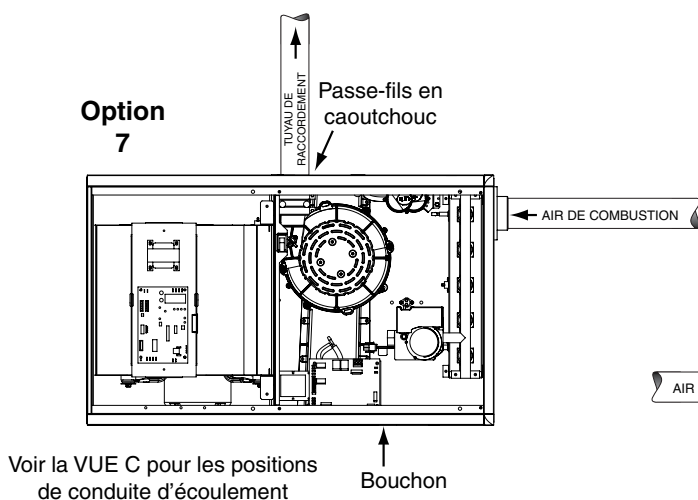
Figure 27. Options de conduit d'évent et de condensat – Générateurs d'air chaud horizontaux
