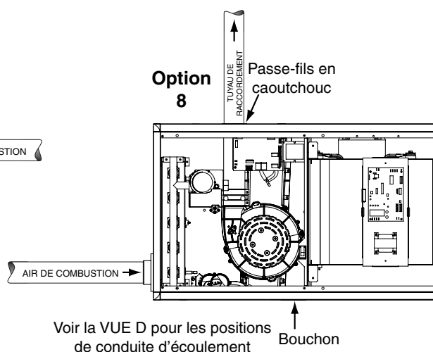
Figure 27. Options de conduit d'évent et de condensat – Générateurs d'air chaud horizontaux
