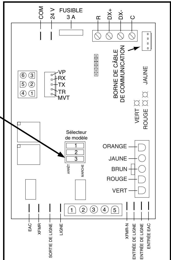
Figure 24. Tableau de commande de générateur d'air chaud à modulation
