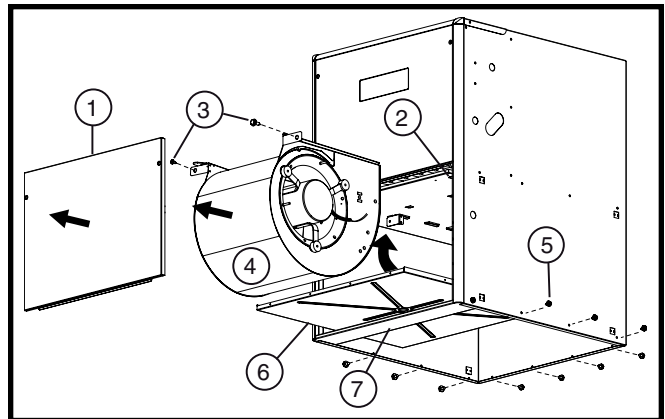
Figure 13. Désassemblage du panneau inférieur
