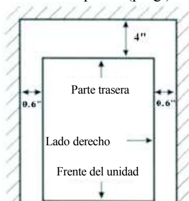
Distancias de Instalación: Vista superior (pulg.)
