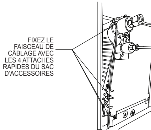
DÉTAIL A
