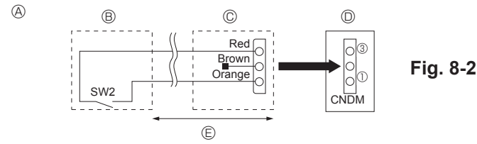
Fig. 8-2 Ⓐ Ejemplo de diagrama de circuito (Función de demanda) Ⓑ Disposición sur site Ⓒ Adaptador de contacto externo (PAC-SC36NA-E) Ⓓ Cuadro de control de la unidad exterior Ⓔ Máx. 10 m, 33 ft
