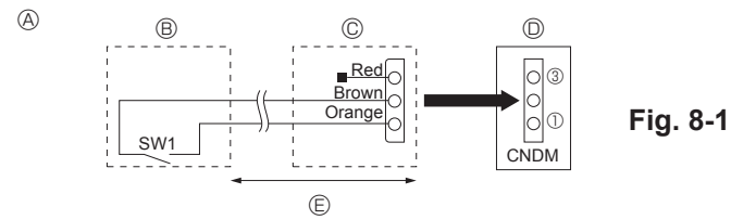
Fig. 8-1 Ⓐ Ejemplo de diagrama de circuito (modo de reducción del ruido) Ⓑ Arreglo in situ Ⓒ Adaptador de contacto externo (PACS-C36NA-E) Ⓓ Cuadro de control de la unidad exterior Ⓔ Máx. 10 m, 33 ft
