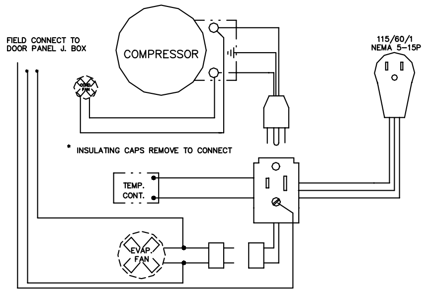
WIRING DIAGRAM CM-156-50
