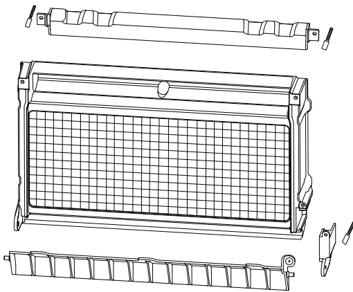
Retire el tornillo de apriete manual de la cubierta del interruptor del recipiente, afirme la compuerta, y retire
