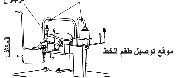
توصيل طقم عداد متشعب أو خرطوم مزود بضغطات لقلب الصمام عند طرفيه
