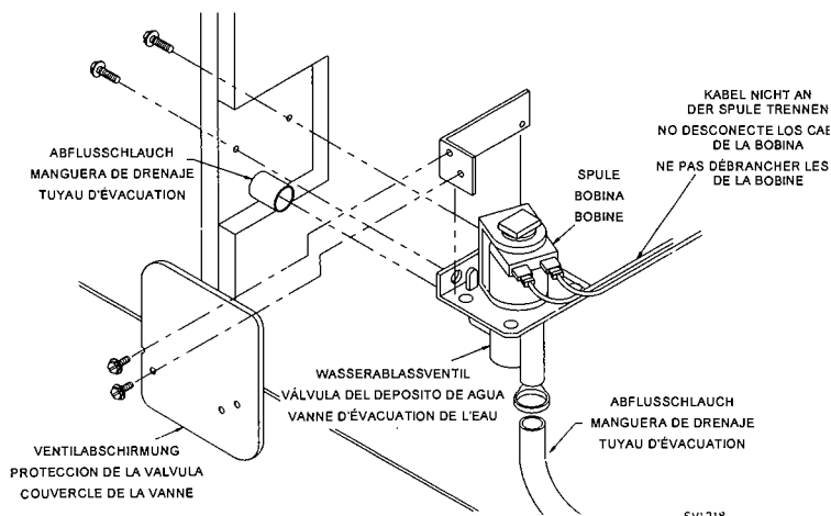
Abbildung 11. ENTFERNUNG DES ABLASSVENTILS
