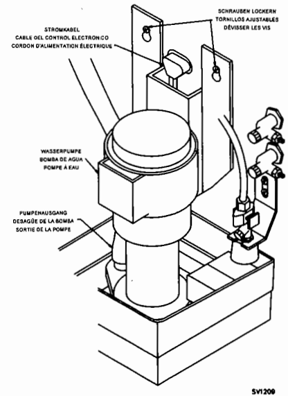
Abbildung 12. ENTFERNUNG DER WASSERPUMPE
