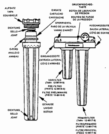
Abbildung 19. WASSERFILTRATION
