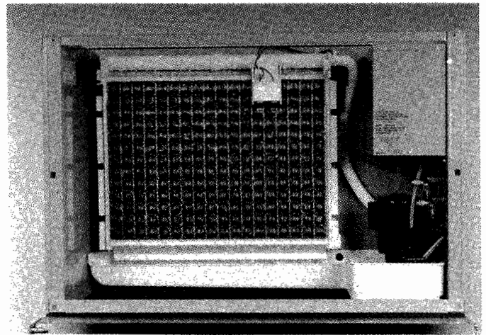
Abbildung 3. GEFRIERSEQUENZ
