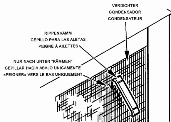
Abbildung 9. VERBOGENE VERDICHTERRIPPEN GERADE BIEGEN
