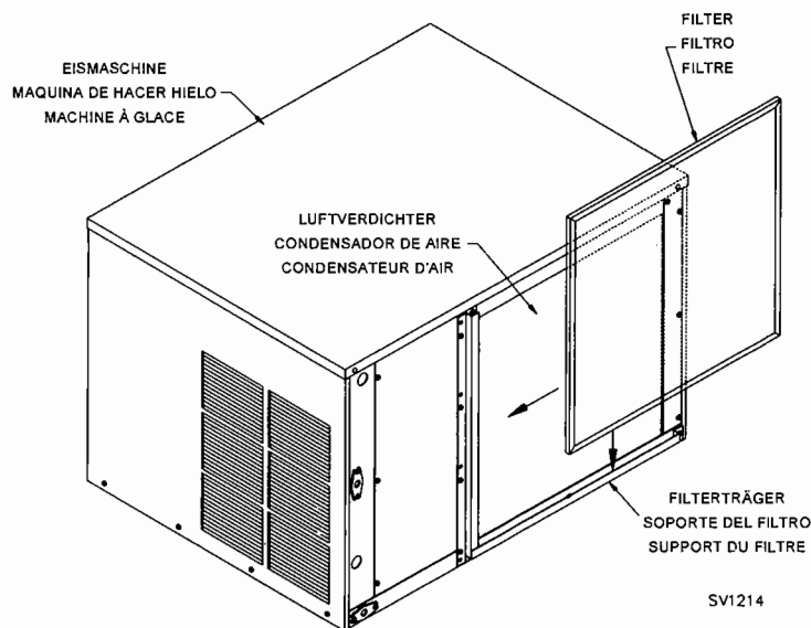
Abbildung 8. AUTONOMER, LUFTGEKÜHLTER FILTER
