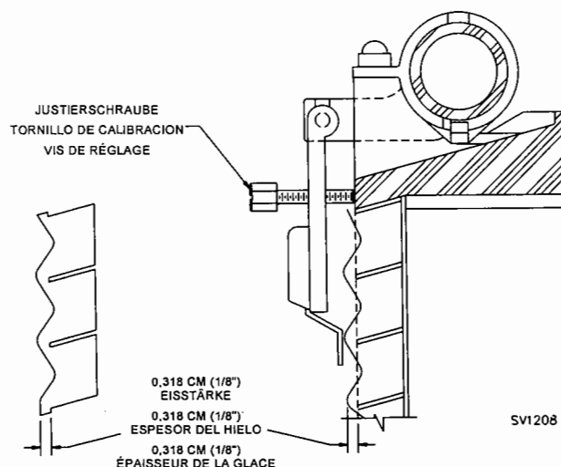
Abbildung 7. ÜBERPRÜFUNG DER EISSTÄRKE
