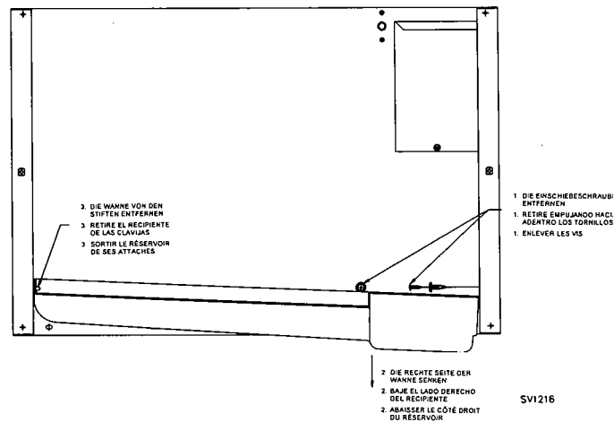
Abbildung 14. ENTFERNUNG DER WASSERWANNE
