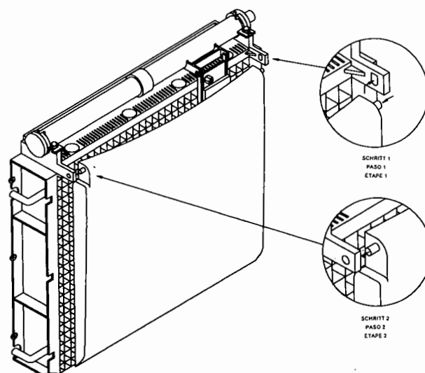
Abbildung 18. ENTFERNUNG DES WASSERVORHANGES
