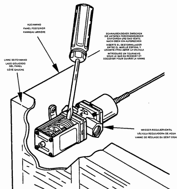
Abbildung 20. MANUELLES ÖFFNEN DES WASSER-REGULIERVENTILES
