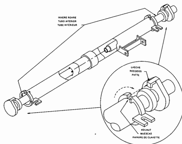
Abbildung 17. ZERLEGUNG DER WASSERVERTEILERRÖHRE
