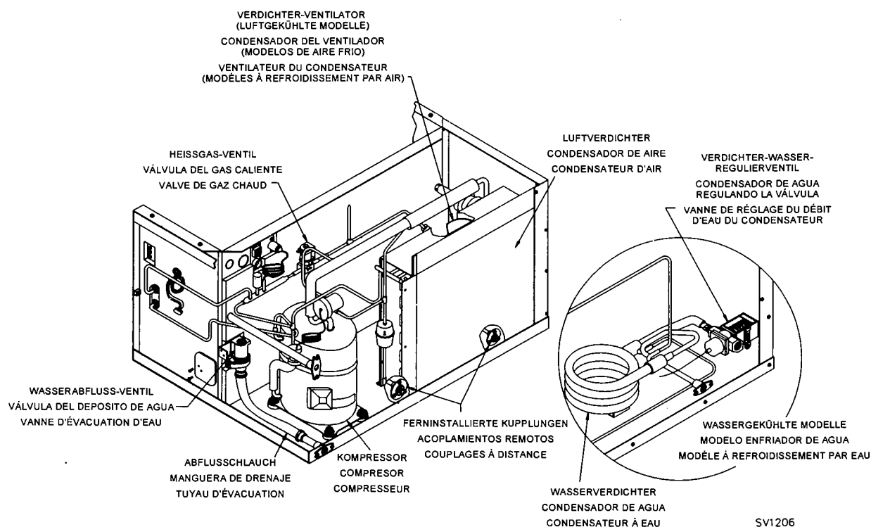
Abbildung 2. POSITION DER KOMPONENTEN/IDENTIFIZIERUNG Figura 2. LOCALIZACION E IDENTIFICACION DE LOS COMPONENTES Figure 2. EMBLACEMENT/IDENTIFICATION DES COMPOSANTS
