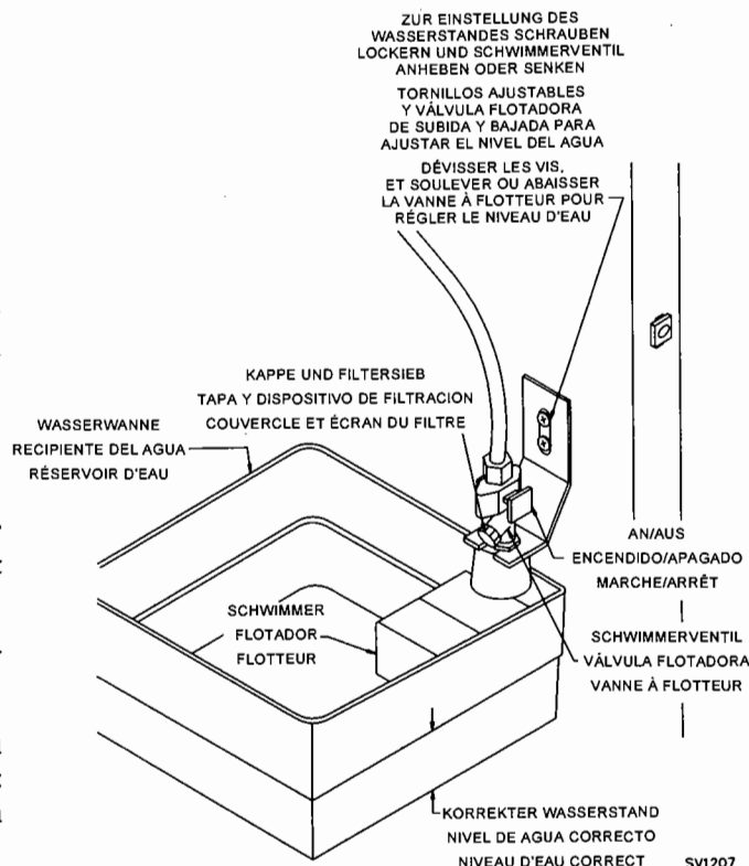
Abbildung 6. ÜBERPRÜFUNG DES WASSERSTANDES
