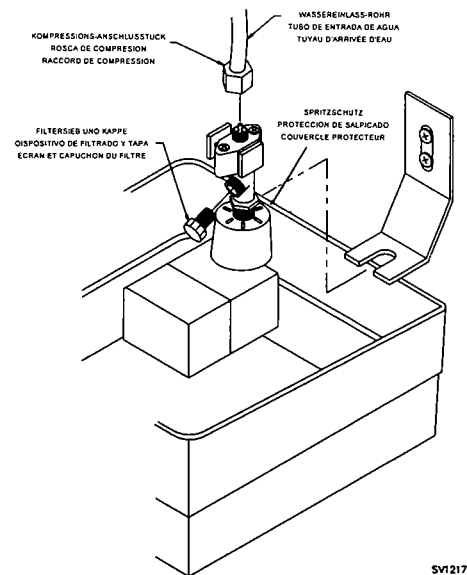
Abbildung 15. ENTFERNUNG DES SCHWIMMERVENTILS
