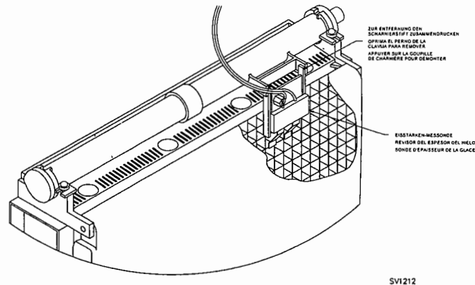
Abbildung 13. ENTFERNUNG DER EISSTÄRKEN-MESSSONDE
