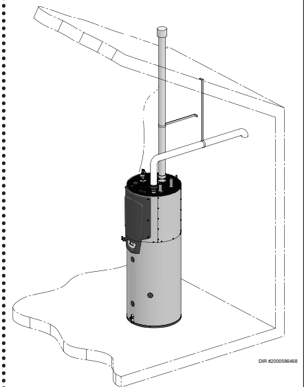
Figure 2-5 Évacuation verticale, apport d'air mural
