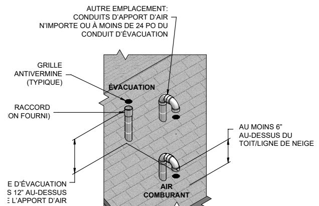
Figure 4-1B Terminaisons verticales d'apport d'air et d'évacuation en acier inoxydable
