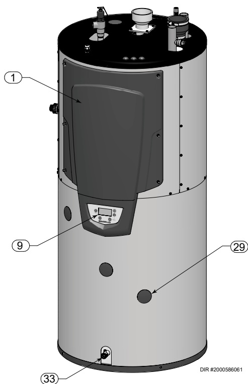
Vue avant - Modèles SWR125 à 200
