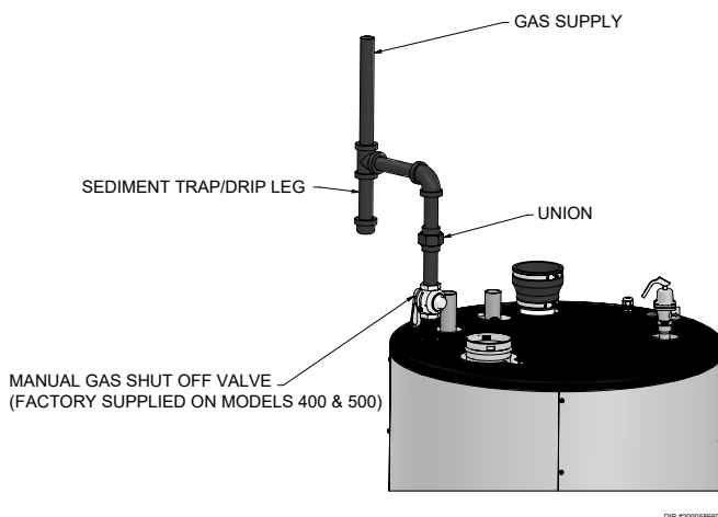
Figure 6-2 Conduites d'alimentation en gaz - Modèles 400 à 500
