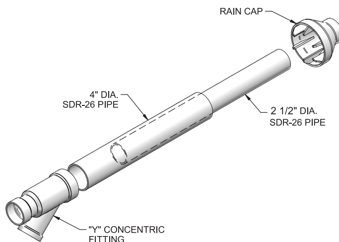
Figure 3-8 Contenu du kit 100140484 - 285 à 500
