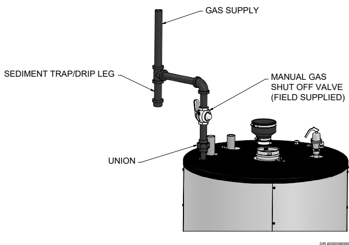
Figure 6-2 Conduites d'alimentation en gaz - Modèles 400 à 500
