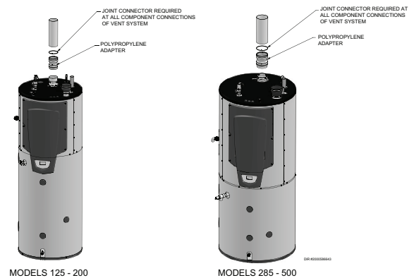
Figure 2-9 Conduit d'évacuation en polypropylène à proximité d'un chauffe-eau
