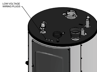
Figure 7-1 Câblage réalisé au chantier
