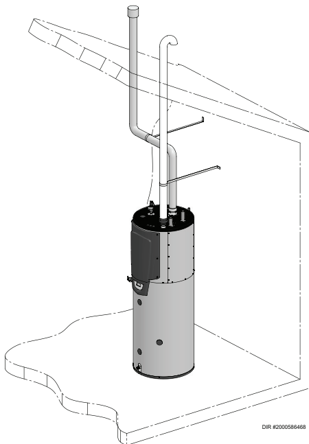
Figure 2-3 Deux conduits, vertical à travers le toit
