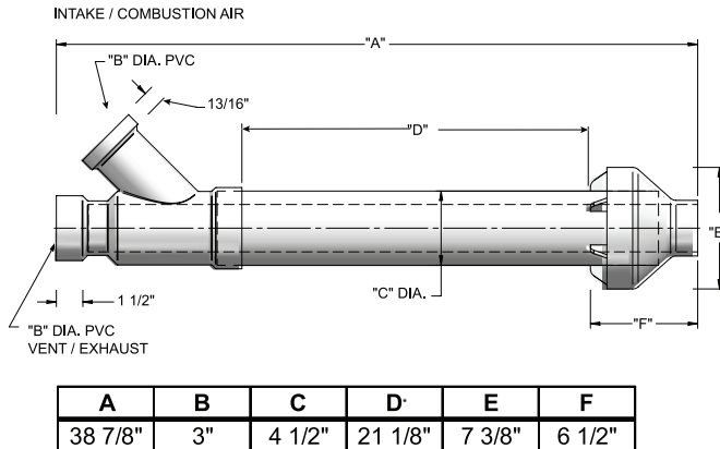
Figure 3-9 Dim. terminaison concentrique - Modèles 125 à 200 / 100140480
