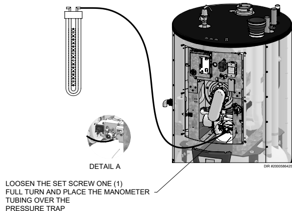
Figure 6-4 Vérification de la pression d'entrée - Modèles 125 à 285
