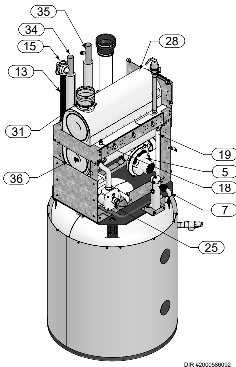
Vue arrière – Modèles SWA400 et 500
