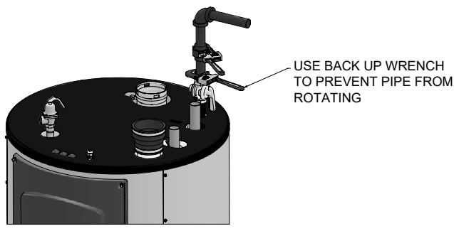
Figure 6-3 Raccord d'entrée de gaz retenu par une clé
