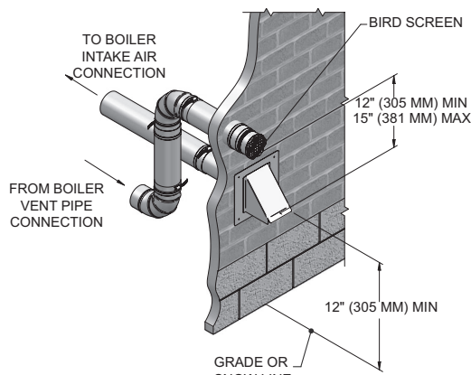
Figure 3-1D Figure 3-1D Ventilation optionnelle en acier inoxydable - Positionnement typique des terminaisons d'apport d'air et d'évacuation en acier inoxydable (à pied-d'oeuvre)
