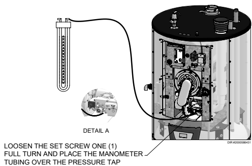
Figure 6-5 Vérification de la pression d'entrée - Modèle 400
