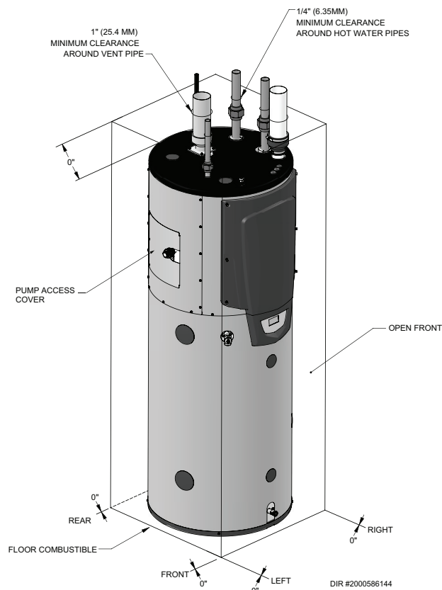
Figure 1-2 Installation dans une alcôve - Distances de dégagement minimales
