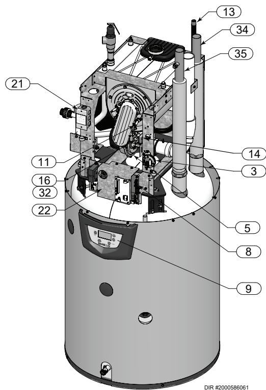
Côté gauche (intérieur de l'appareil) - Modèles SWR125 à 200
