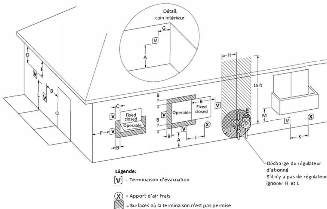
Figure 3-3A Dégagements de la terminaison, ventilation directe
