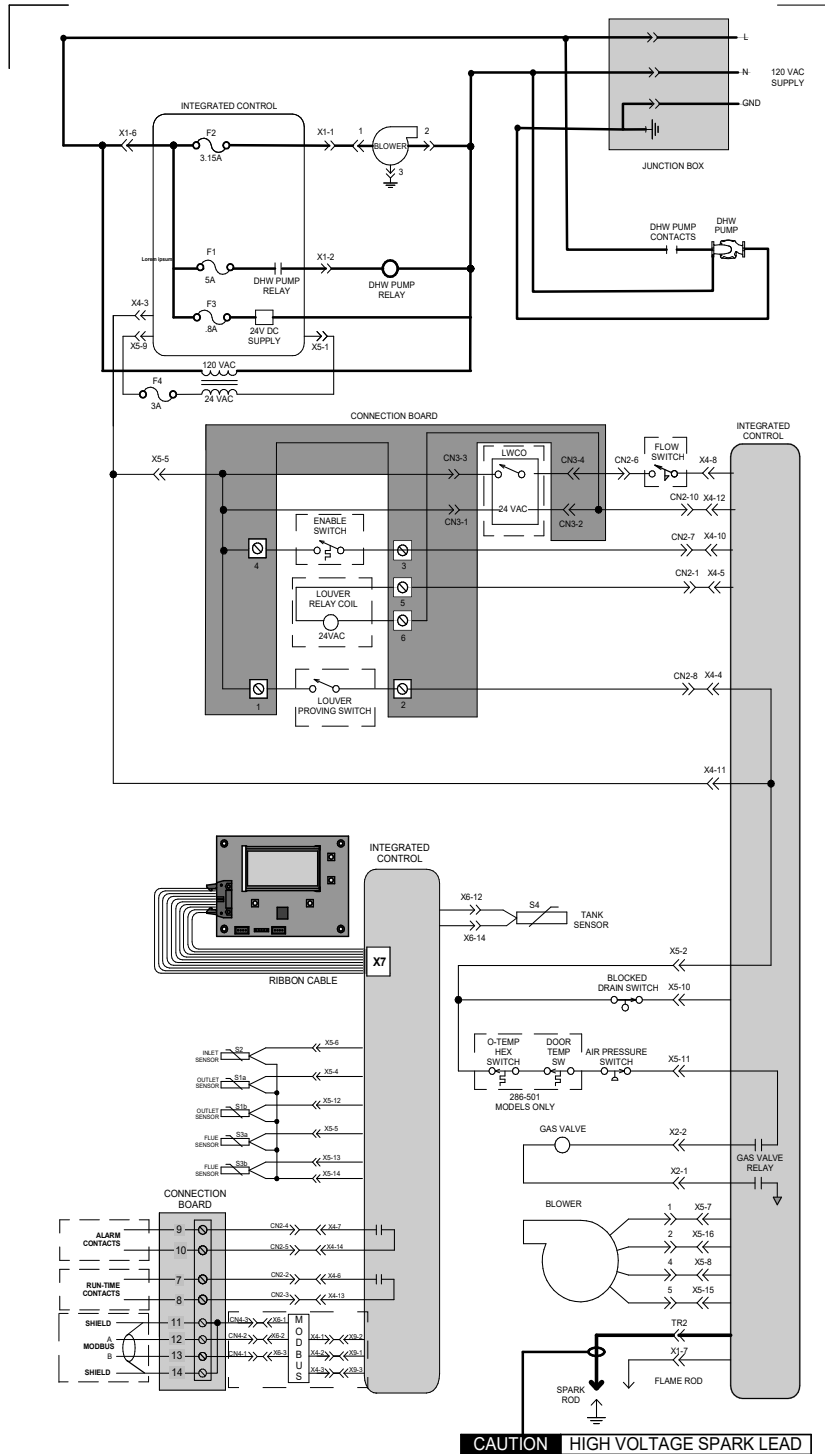
Figure 13-1 Schéma électrique
