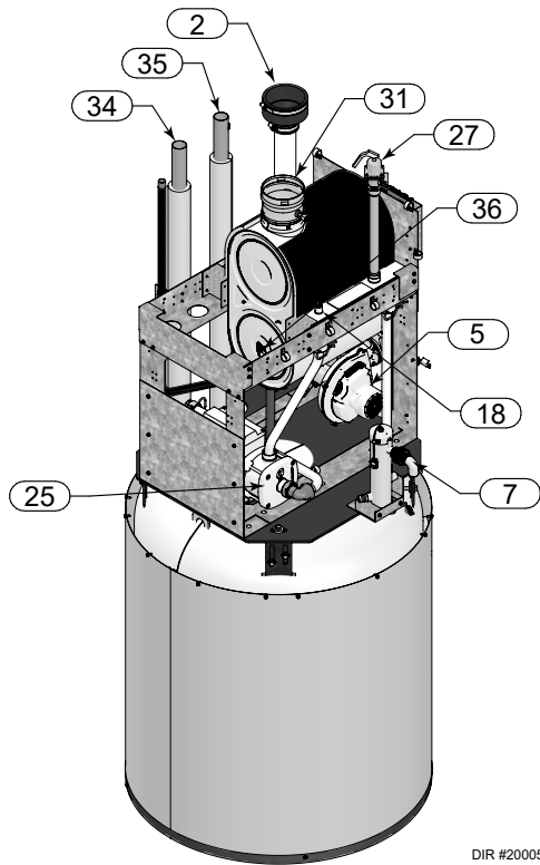
Vue arrière – Modèle SWA285
