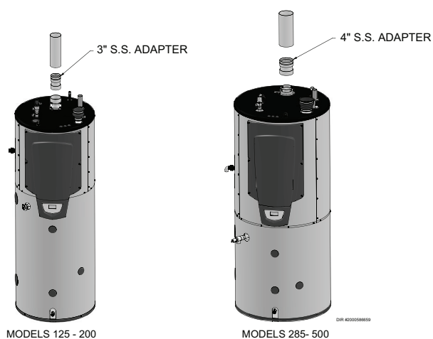
Figure 2-10 Conduit d'évacuation en inox à proximité d'un chauffe-eau
