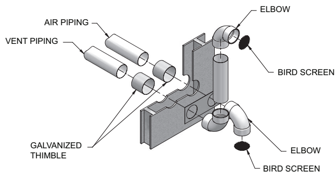
Figure 3-5B Plusieurs terminaisons d'évacuation optionnelles (à pied-d'oeuvre, doit aussi être conforme à Figure 3-1B)
