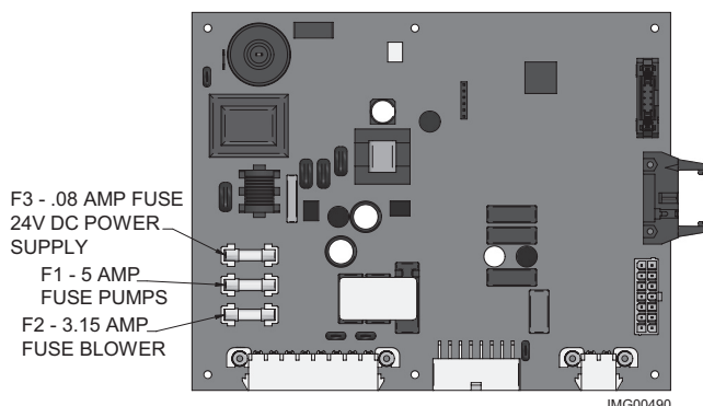
Figure 12-1 Fusibles du contrôleur électronique
