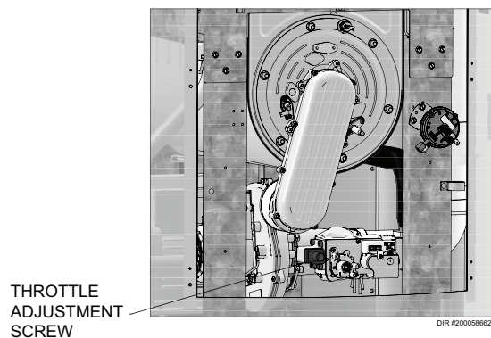
Figure 12-3 Réglage de la vanne du gaz: modèles 400 et 500
