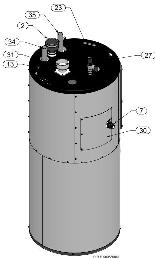
Vue arrière - Modèles SWR125 à 200
