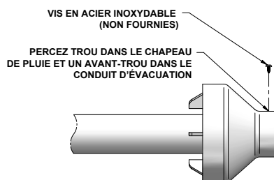
Figure 3-11 Assemblage optionnel, chapeau de pluie au conduit d'évacuation
