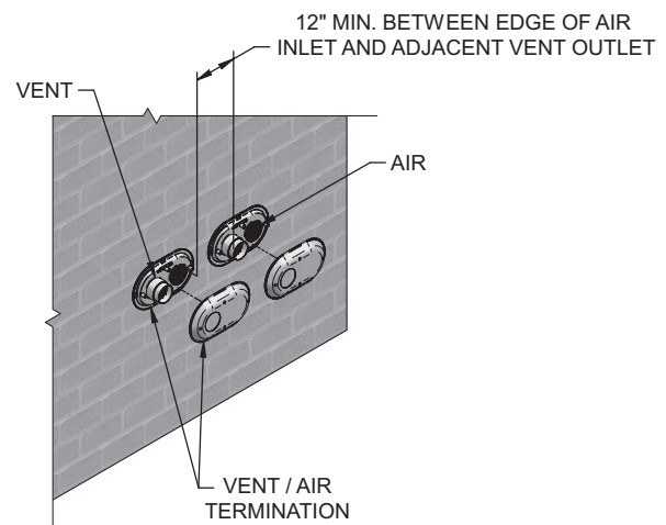
Figure 3-5A Plusieurs terminaisons d'évacuation (doit aussi être conforme à Figure 3-1A)
