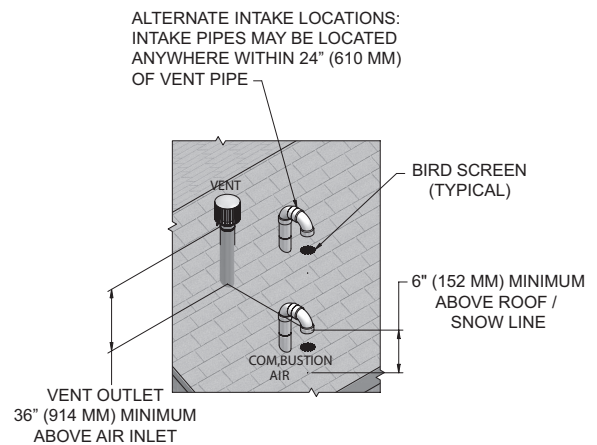
Figure 4-1B Terminaisons verticales d'apport d'air et d'évacuation en acier inoxydable
