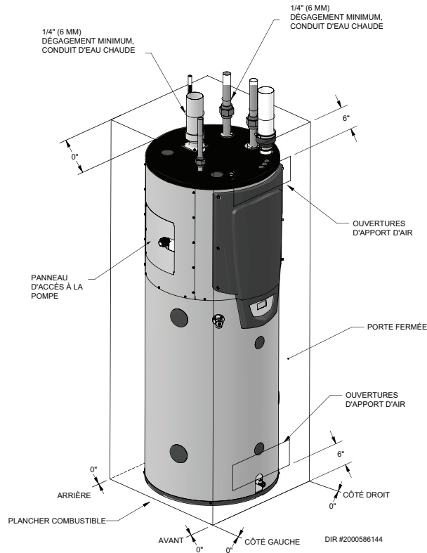
Figure 1-2 Installation dans une alcôve - Distances de dégagement minimales
