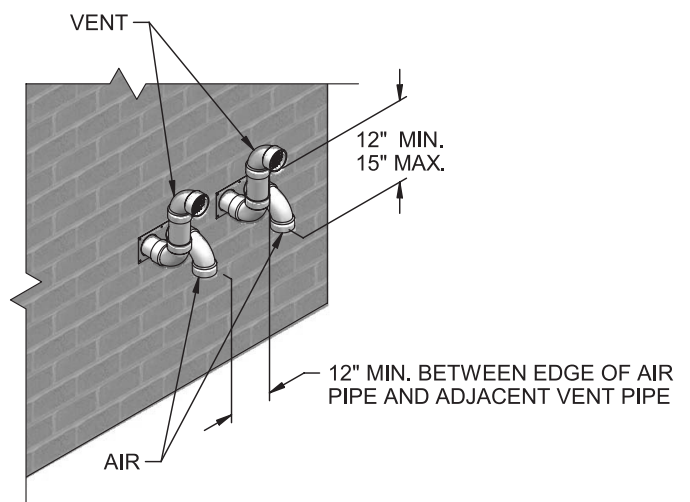
Figure 3-5B Plusieurs terminaisons d'évacuation optionnelles (à pied-d'oeuvre, doit aussi être conforme à Figure 3-1B)
