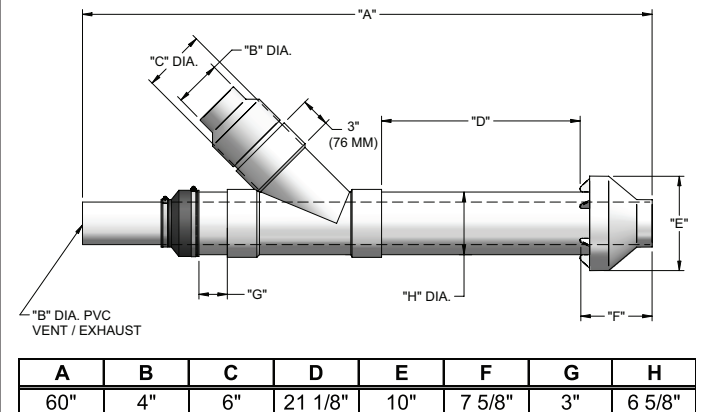
Figure 3-10 Dim. terminaison concentrique - Modèles 285 à 500 / 100140484
