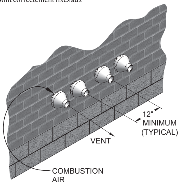
Figure 3-13 Terminaison concentrique, apport d'air et évacuation
