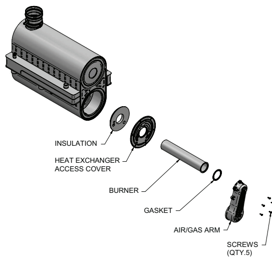
Figure 11-2 Assemblage du brûleur
