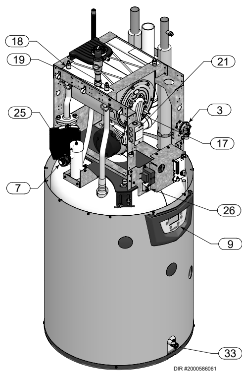
Côté droit (intérieur de l'appareil) - Modèles SWR125 à 200
