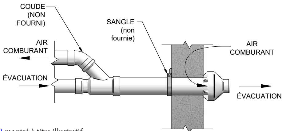
Figure 3-12 Fixation murale d'une terminaison concentrique
