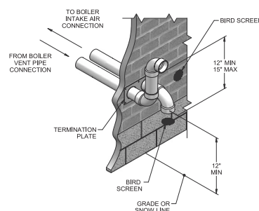
Figure 3-1B Terminaison murale optionnelle en PVC/CPVC/polypropylène (à pied-d'oeuvre)
