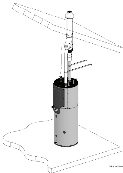
Figure 2-4 Terminaison concentrique verticale en PVC/CPVC
