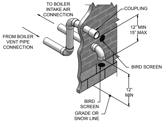
Figure 3-1D Figure 3-1D Ventilation optionnelle en acier inoxydable - Positionnement typique des terminaisons d'apport d'air et d'évacuation en acier inoxydable (à pied-d'oeuvre)
