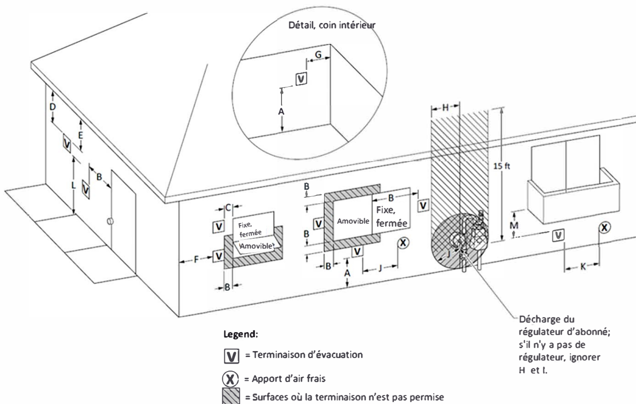
Figure 3-3B Dégagements de la terminaison, autre que ventilation directe (DV)
