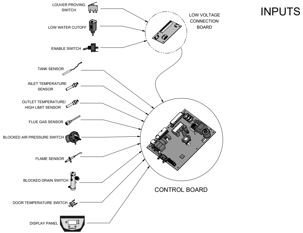
Figure 7-4 Entrées et sorties de contrôle
