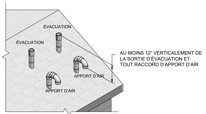
Figure 4-3 Terminaisons verticales optionnelles, plusieurs chauffe-eau
