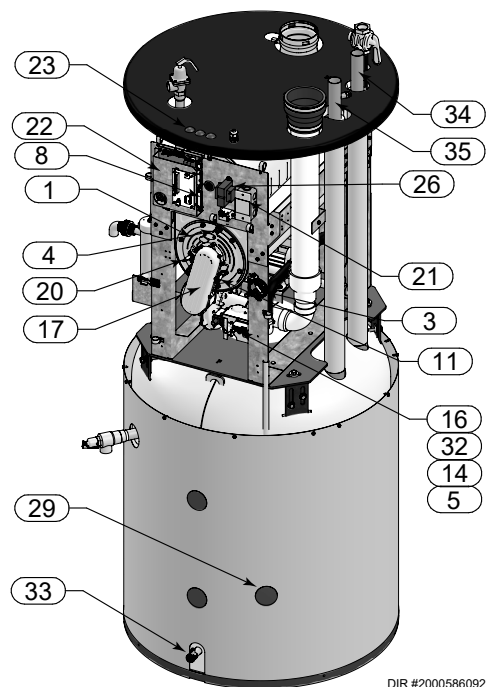
Côté droit (intérieur de l'appareil) – Modèles SWA400 et 500
