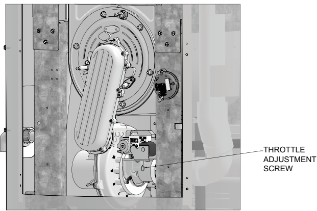
Figure 12-2 Réglage de la vanne du gaz: modèles 125 à 285
