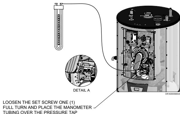
Figure 6-6 Vérification de la pression d'entrée - Modèle 500
