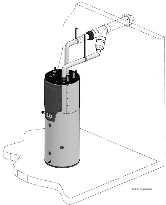
Figure 2-2 Terminaison concentrique murale en PVC/CPVC
