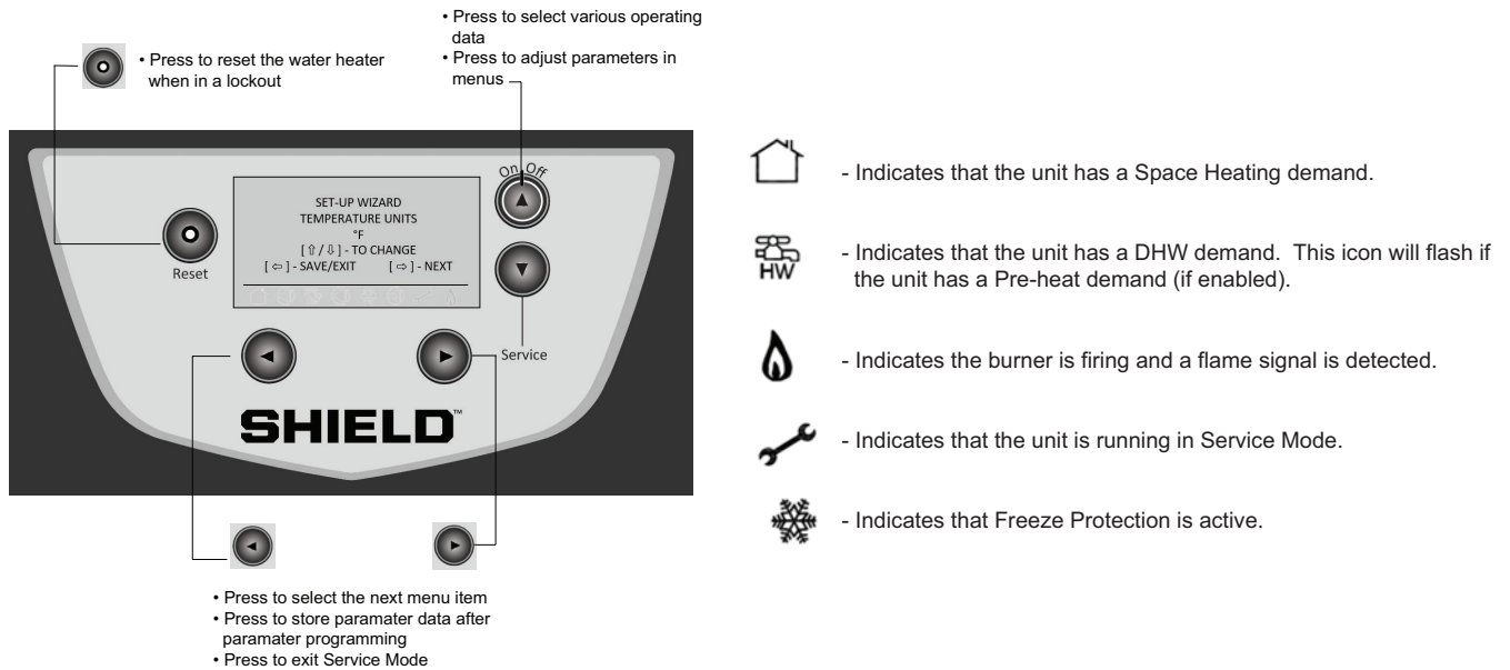
Figure 9-4 Panneau de commande
