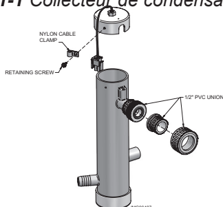
Figure 11-1 Collecteur de condensation
