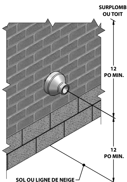
Figure 3-6 Terminaison concentrique murale
