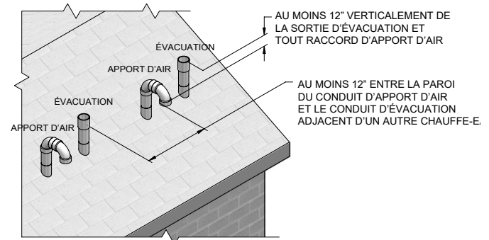
Figure 4-3 Terminaisons verticales optionnelles, plusieurs chauffe-eau
