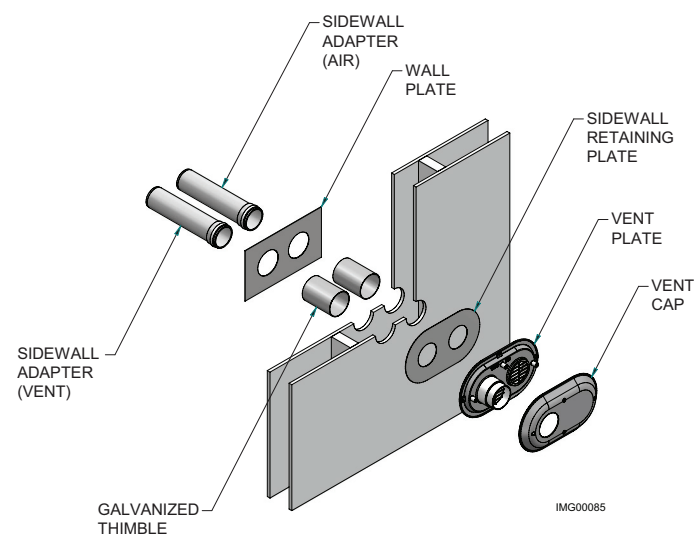
Figure 3-4B Terminaison murale en polypropylène
