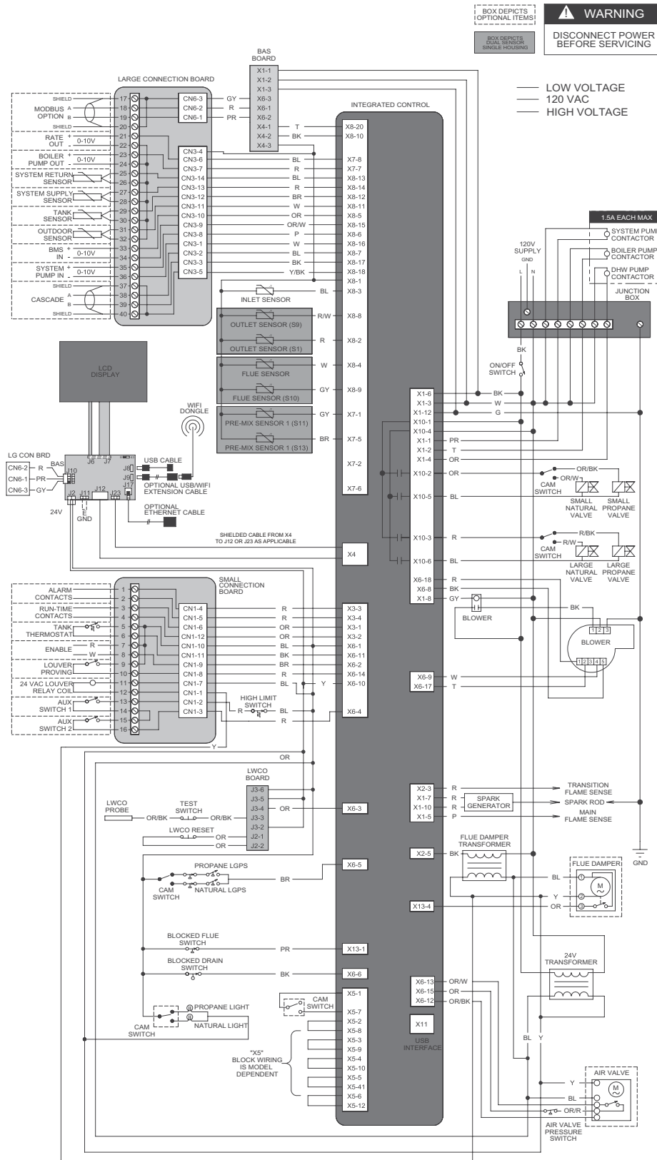
Figure 3-2 Schéma de câblage - Modèles 751 - 2001
