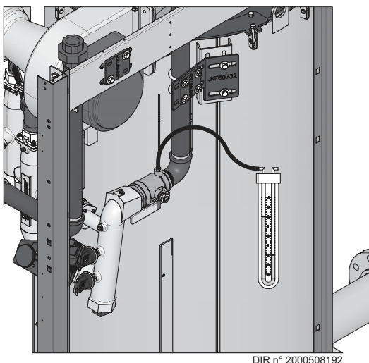
Figure 1-1 Vérification de l'arrivée d'alimentation en gaz_Naturel
