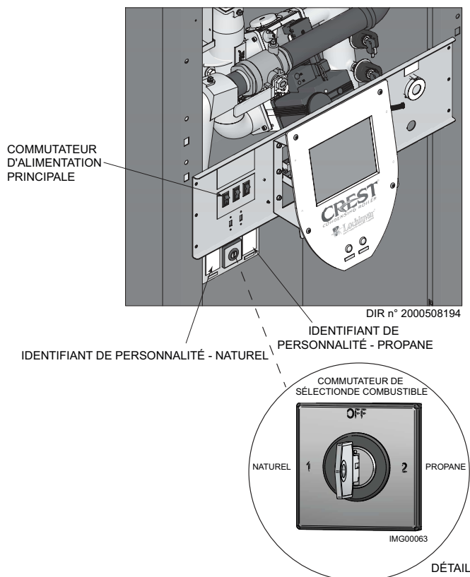
Figure 2-2 Commutateur de sélection de combustible
