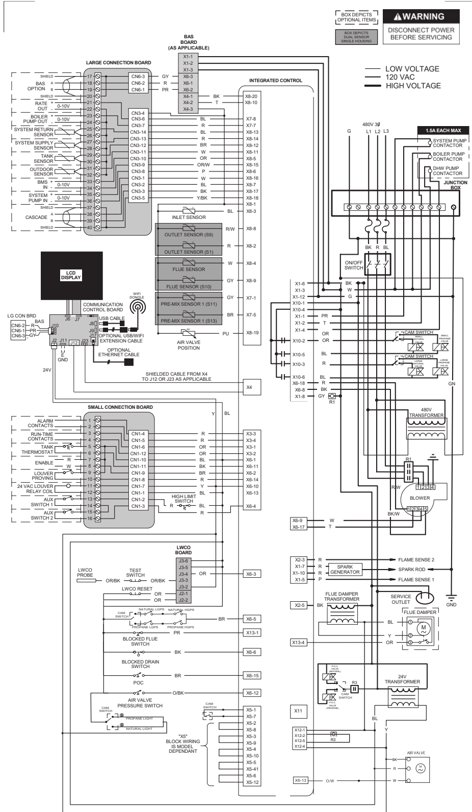
Figure 3-8 Schéma de câblage - Modèle 6001
