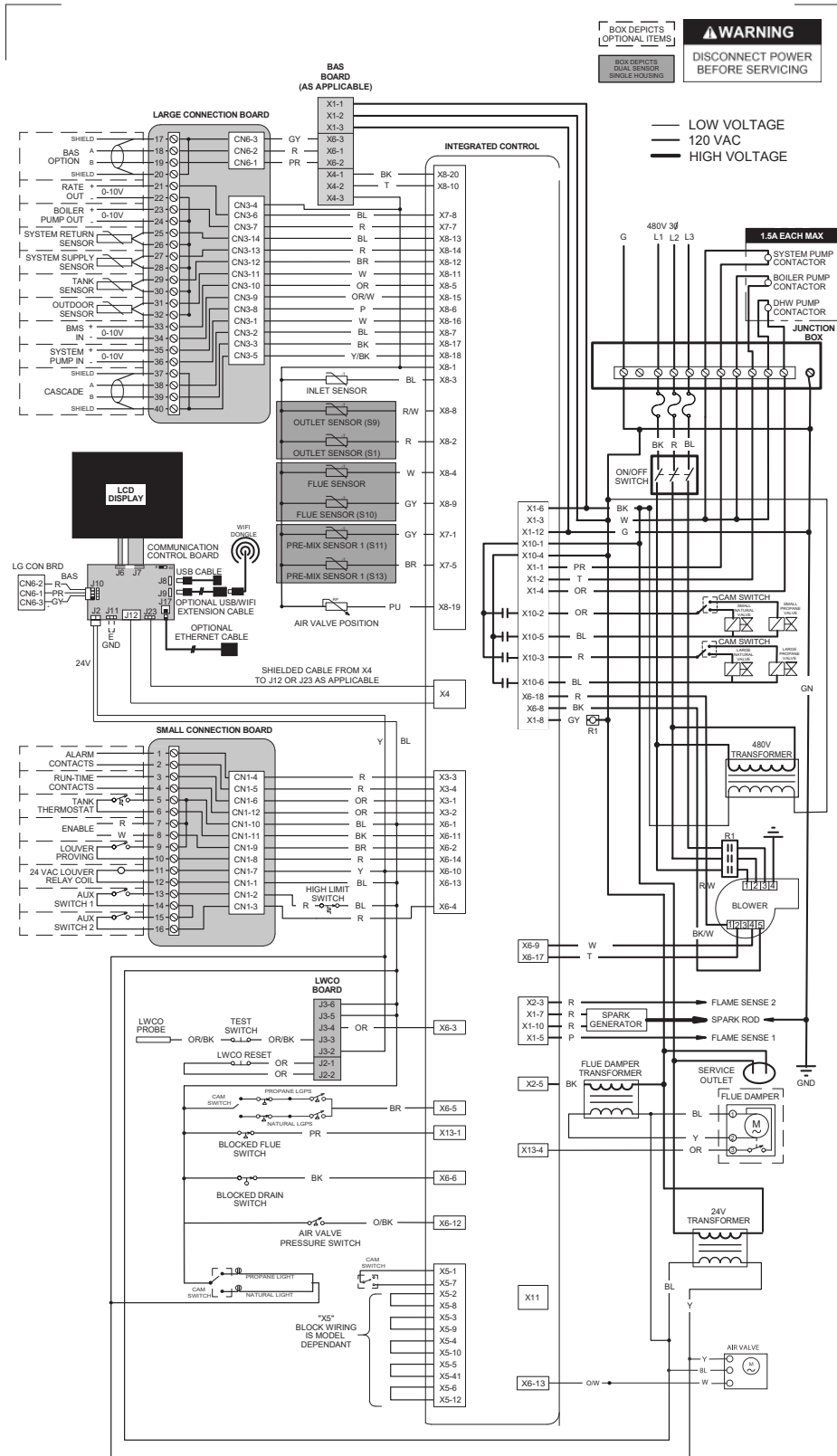
Figure 3-6 Schéma de câblage - Modèles 4001 - 5001
