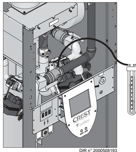
Figure 1-2 Vérification de l'arrivée d'alimentation en gaz_Propane
