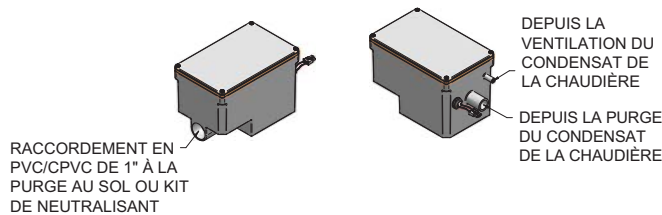
Figure 2-1 Piège à condensat
