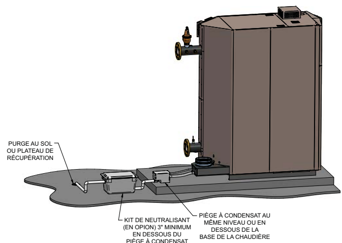
Figure 2-2 Élimination du condensat
