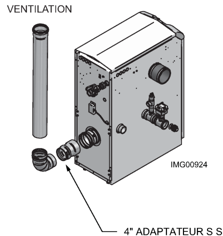
Figure 3-11 Près de la ventilation en acier inoxydable du chauffe-eau Modèle 286
