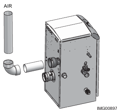
Figure 3-7 À côté de la tuyauterie d'air du chauffe-eau Modèle 286
