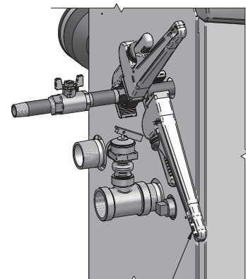
Figure 7-3 Tuyau d'entrée avec clé de retenue
