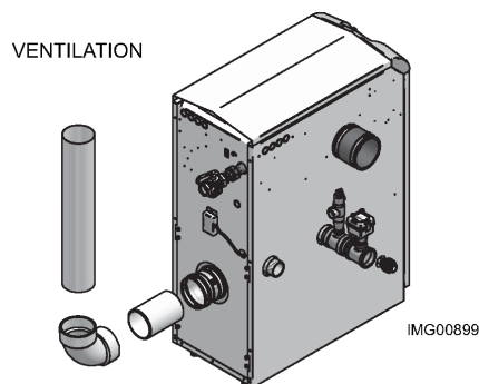
Figure 3-8 Près de la ventilation en PVC/CPVC du chauffe-eau
