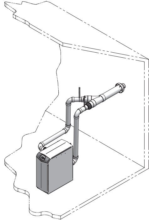
Figure 3-2 Terminaison murale concentrique en PVC/CPVC - Voir page 31 pour d'autres détails
