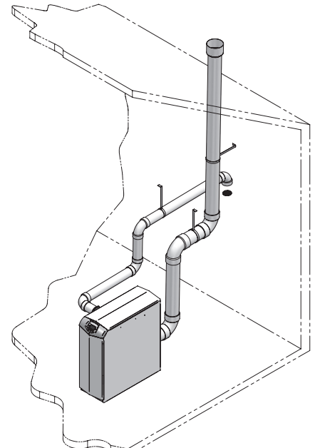
Figure 3-5 Ventilation verticale en Air latéral
