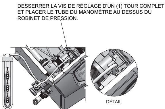
Figure 7-4 Vérification de l'alimentation en gaz d'entrée
