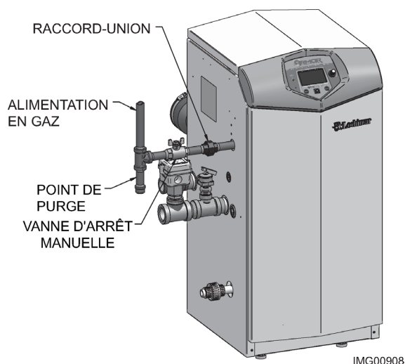
Figure 7-2 Tuyauterie d'alimentation en gaz - Modèle 286
