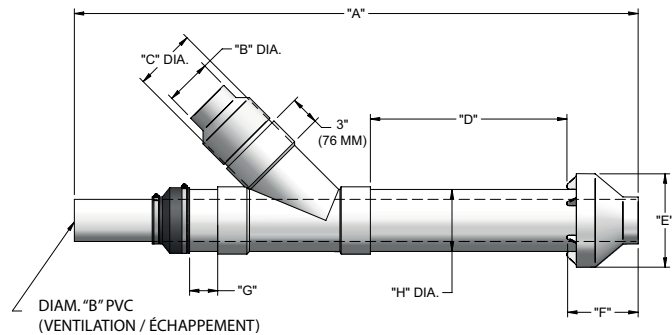
Figure 4-11 Schéma des dimensions de ventilation concentrique - Modèles 286
