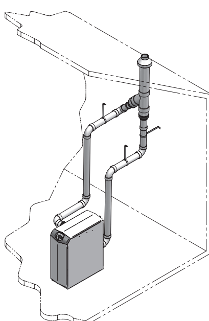
Figure 3-4 Terminaison verticale concentrique en PVC/CPVC - Voir page 36 pour d'autres détails
