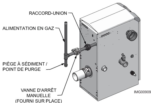
Figure 7-2 Tuyauterie d'alimentation en gaz - Modèle 286
