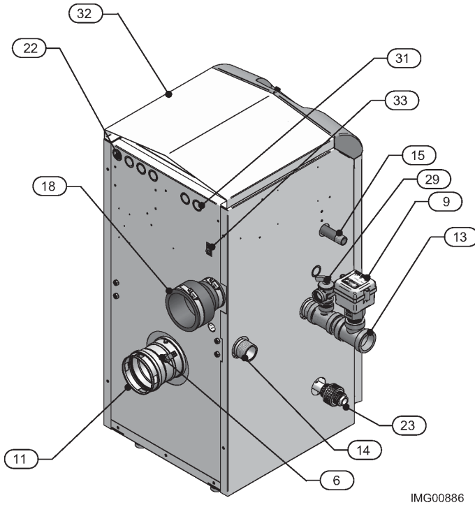
Vue arrière - Modèles 151 - 201
