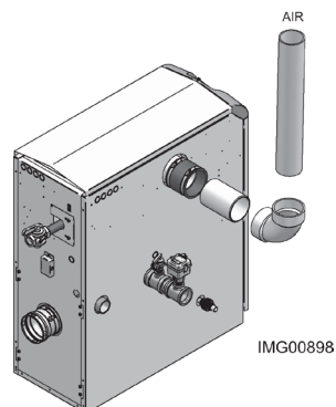
Figure 3-7 À côté de la tuyauterie d'air du chauffe-eau Modèle 286
