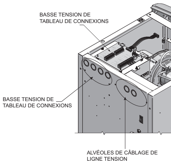
Figure 8-2 Passage des câbles
