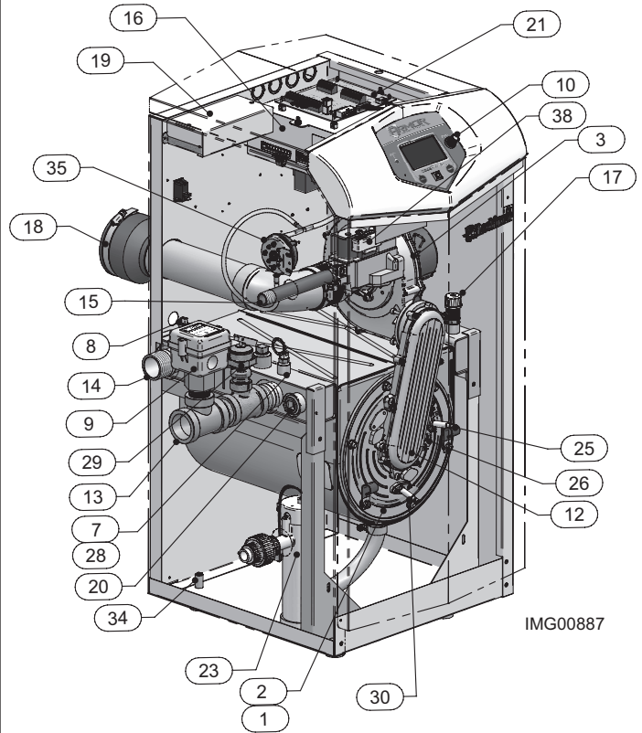
Côté gauche (intérieur de l'appareil) - Modèles 151 - 201
