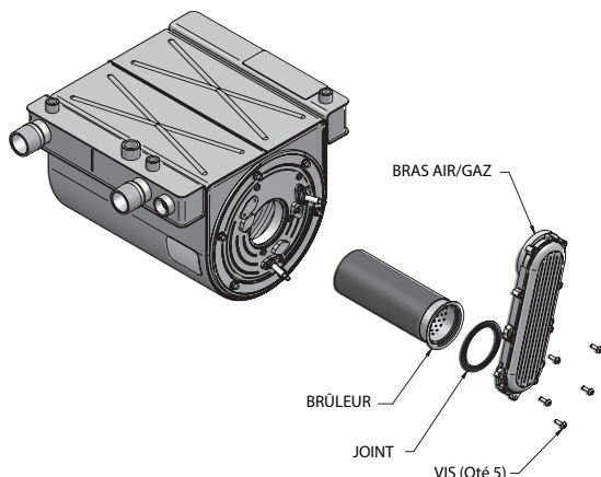
Figure 12-2 Ensemble brûleur
