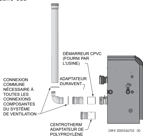
Figure 3-10 Près de la ventilation en polypropylène du chauffe-eau
