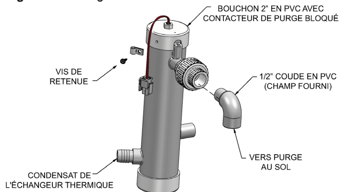
Figure 10-1 Piège à condensat
