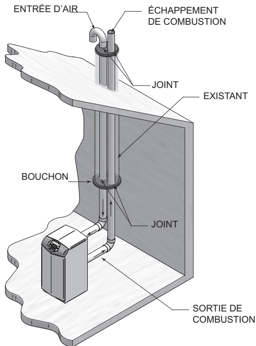
Figure 5-10 Ventilation existante en goutlotte
