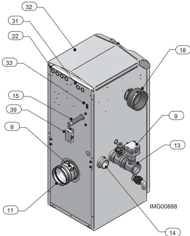
Vue arrière - Modèle 286
