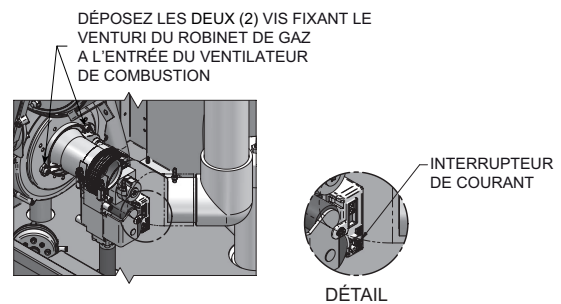
Figure 2-2 Changer de gaz Power Valve & enlèvement Venturi
