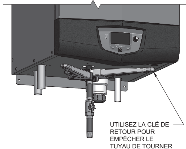
Figure 7-5 Tuyau d'entrée avec clé de retenue
