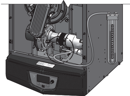
Figure 7-3 Vérification de l'alimentation en gaz d'entrée
