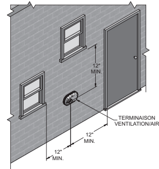
Figure 4-3B Espace alternatif par rapport aux entrées d'air gravitaires avec raccords fournis sur place
