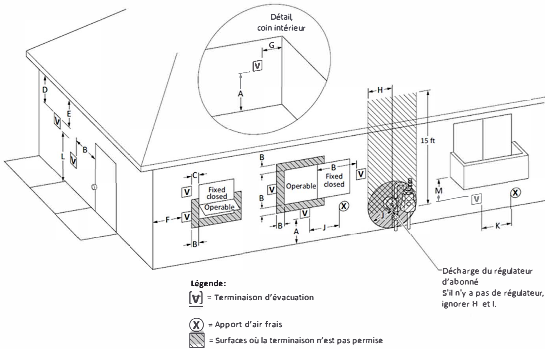
Figure 4-4A Espaces de terminaison de ventilation directe
