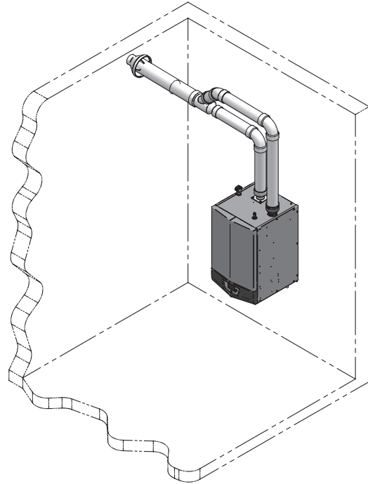
Figure 3-2 Terminaison murale concentrique en PVC/CPVC - Voir page 28 pour d'autres détails
