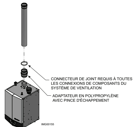
Figure 3-9 Ventilation en Polypropylène à proximité de la chauffe-eau
