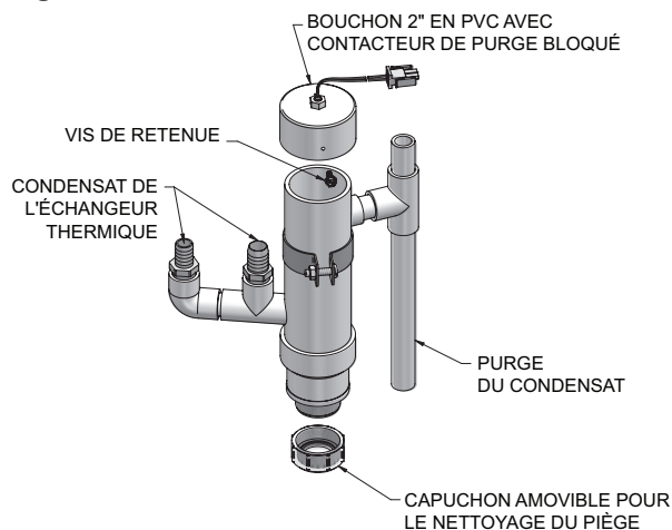
Figure 10-1 PIÈGE À CONDENSAT
