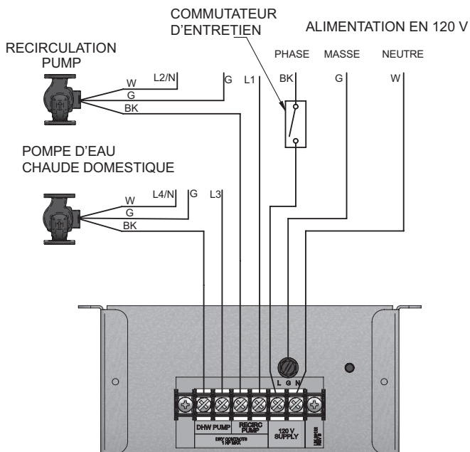
Figure 8-1 Connexions de câblage sur place au secteur
