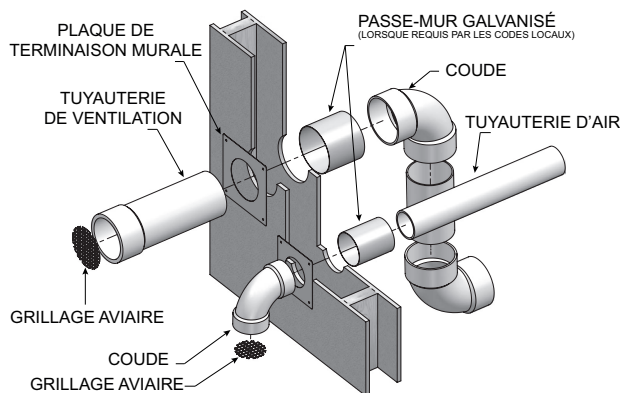
Figure 4-5C Ensemble de terminaison murale classique - PVC/CPVC ou acier inoxydable
