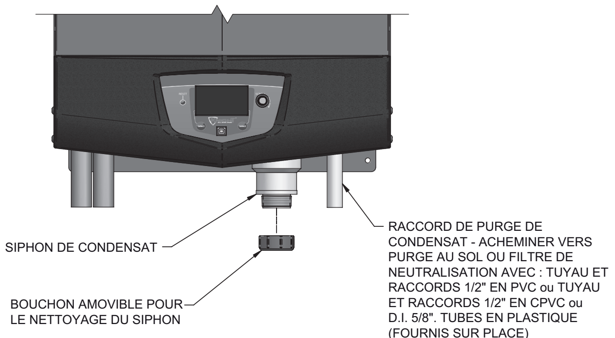
Figure 9-1 Rejet du condensat
