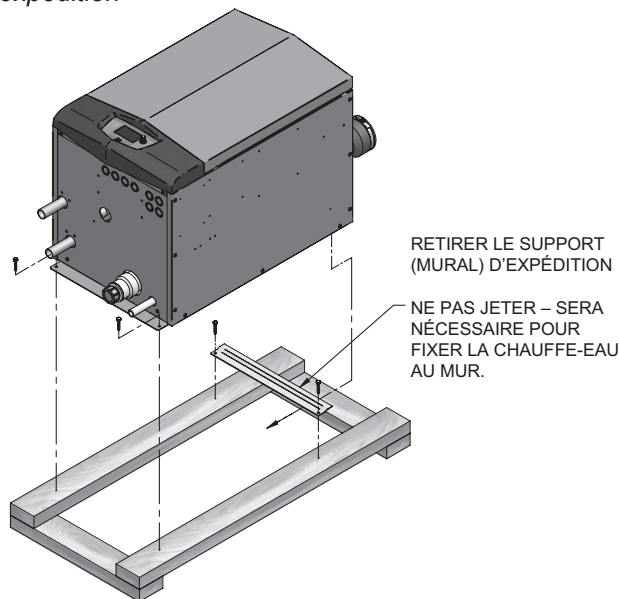
Figure 2-1 chauffe-eau montée sur une palette d'expédition
