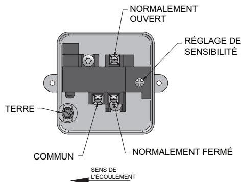
Figure 6-2 Réglage du flussostat
