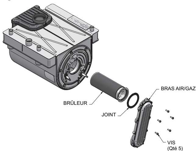
Figure 12-2 Ensemble brûleur
