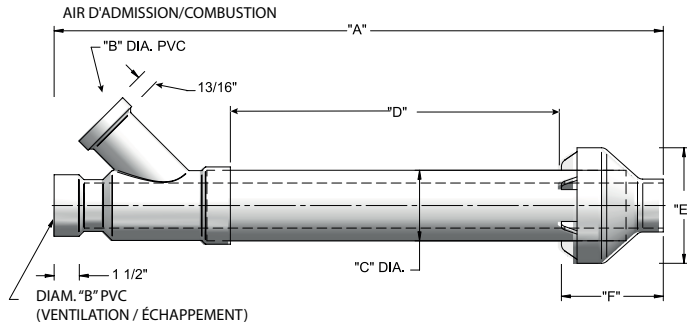
Figure 4-9 Schéma des dimensions de ventilation concentrique
