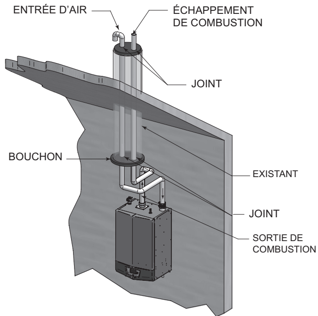
Figure 5-10 Ventilation existante en goutte
