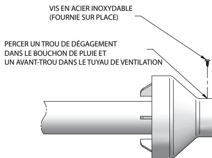
Figure 4-10 Montage alternatif du bouchon de pluie sur le tuyau de ventilation
