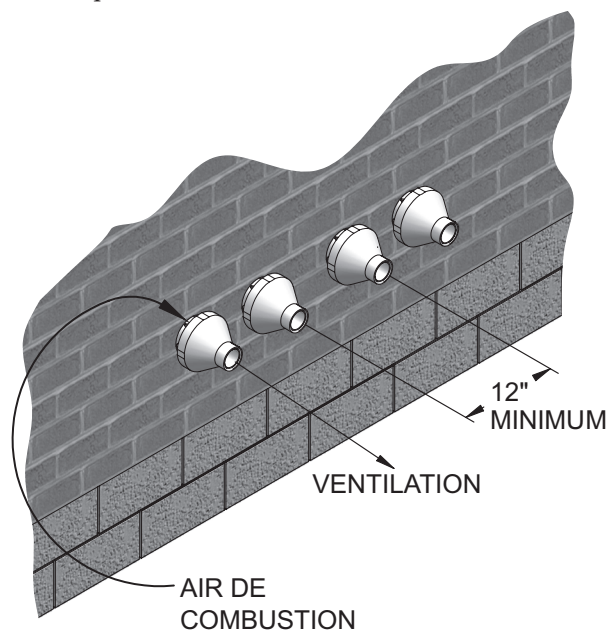
Figure 4-12 Terminaison de ventilation concentrique et d'air de combustion
