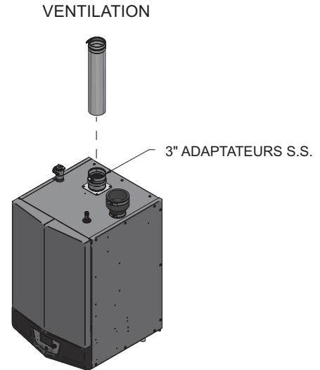
Figure 3-10 Près de la ventilation en acier inoxydable du Chauffe-eau
