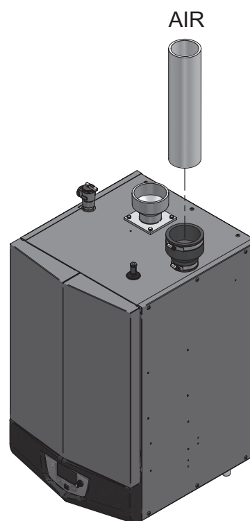
Figure 3-6 À côté de la tuyauterie d'air du chauffe-eau
