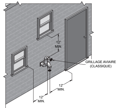
Figure 4-3B Espace alternatif par rapport aux entrées d'air gravitaires avec raccords fournis sur place
