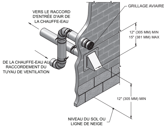
Figure 4-1C Autre terminaison de ventilation en PVC/CPVC/SS - Terminaison murale classique en acier inoxydable air et ventilation avec raccords fournis sur place
