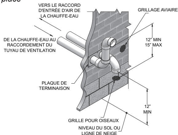
Figure 4-1B Terminaison latérale en PVC/CPVC alternative d'air et de ventilation, avec raccords fournis sur place
