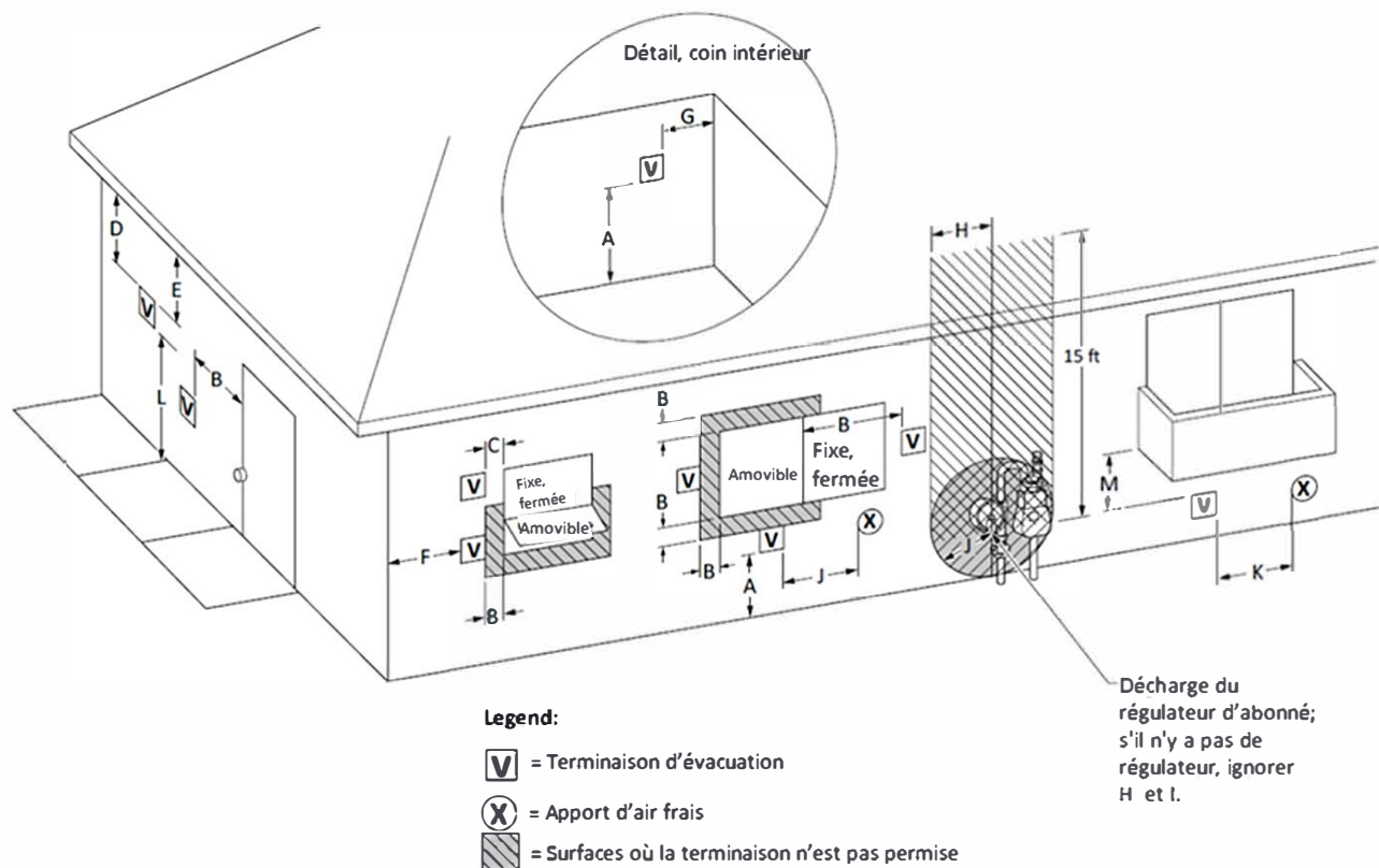
Figure 4-4B Autres que les espaces de terminaison de ventilation directe
