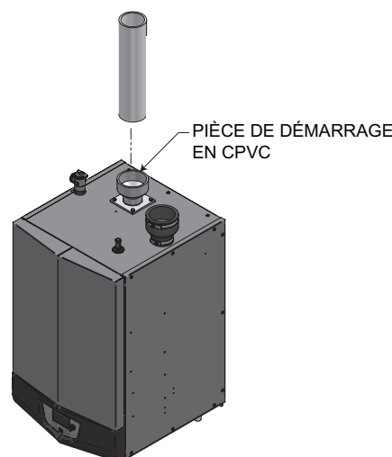
Figure 3-7 Ventilation en PVC/CPVC à proximité de la chauffe-eau
