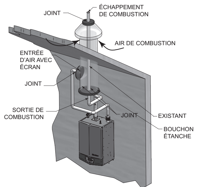
Figure 5-9 Exemple 2 de ventilation concentrique
