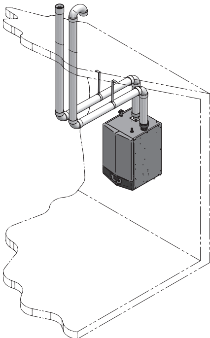
Figure 3-3 Terminaison verticale à deux tuyaux - Voir page 31 pour d'autres détails
