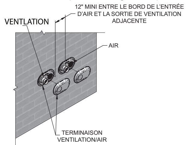
Figure 4-6A Terminaisons pour ventilations multiples (doivent aussi correspondre à la Figure 4-1A)
