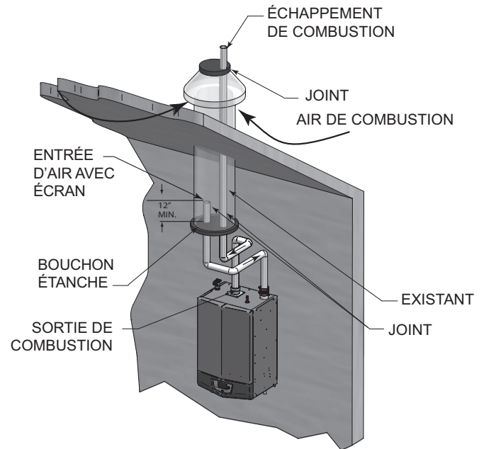
Figure 5-8 Exemple 1 de ventilation concentrique
