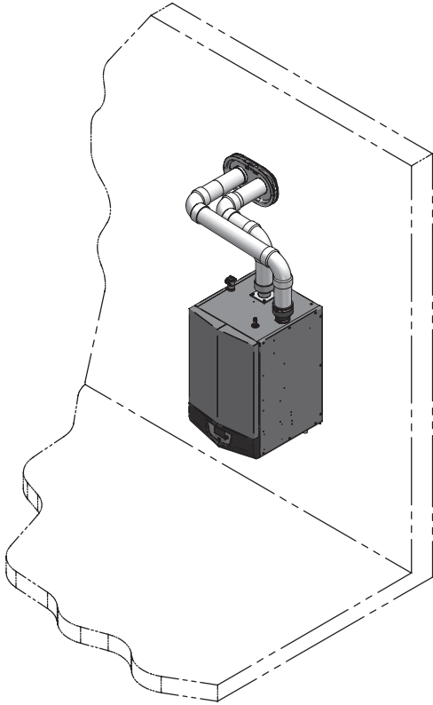
Figure 3-1 Terminaison murale à deux tuyaux - Voir page 21 pour d'autres détails
