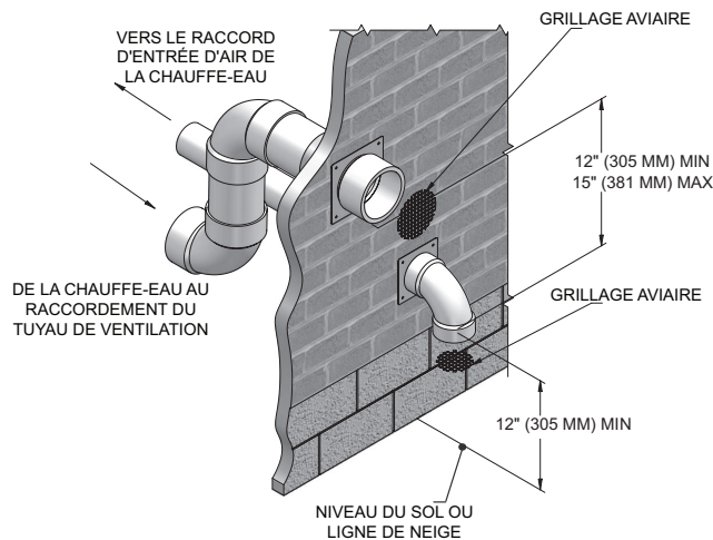
Figure 4-2 Autre terminaison murale en PVC/CPVC/SS/ Polypropylène avec raccords fournis sur place
