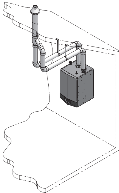
Figure 3-4 Terminaison verticale concentrique en PVC/CPVC - Voir page 33 pour d'autres détails
