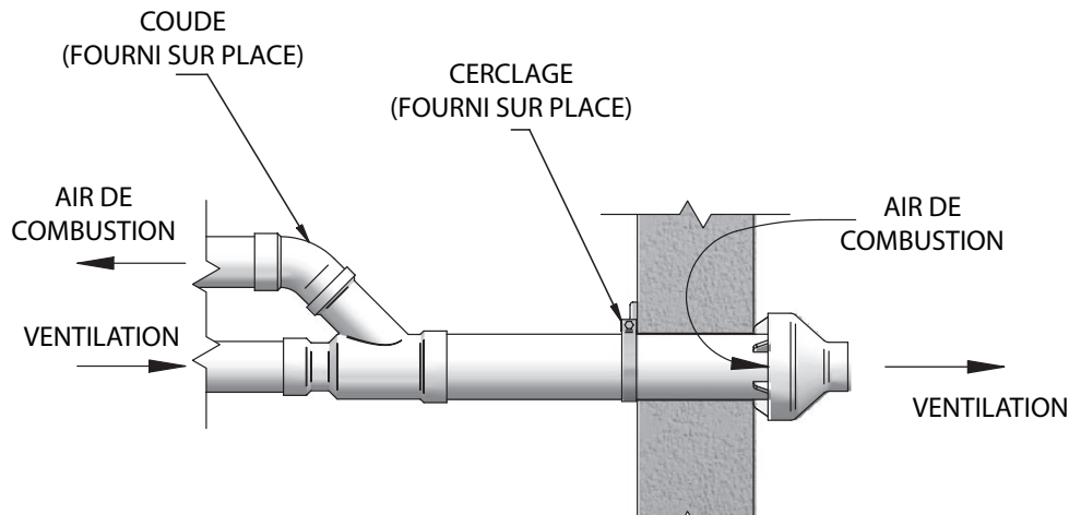
Figure 4-11 Fixation latérale de ventilation concentrique
