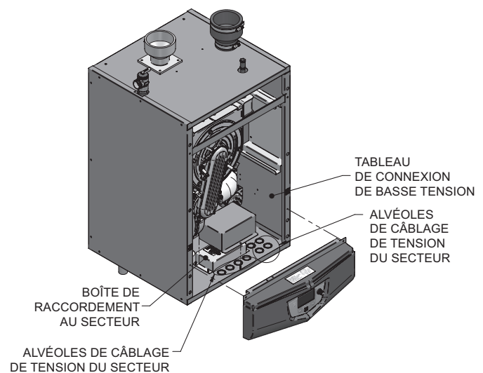
Figure 8-2 Passage des câbles
