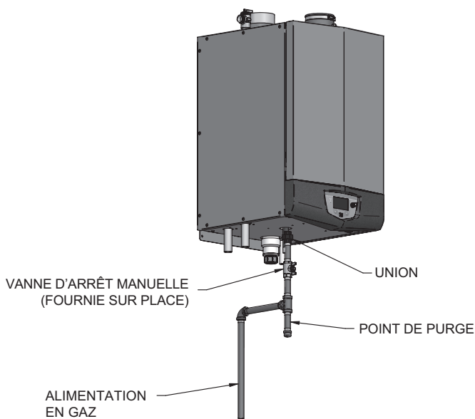
Figure 7-1 Tuyauterie d'alimentation en gaz
