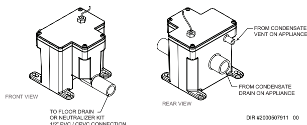
Figure 11-1 Collecteur de condensation
