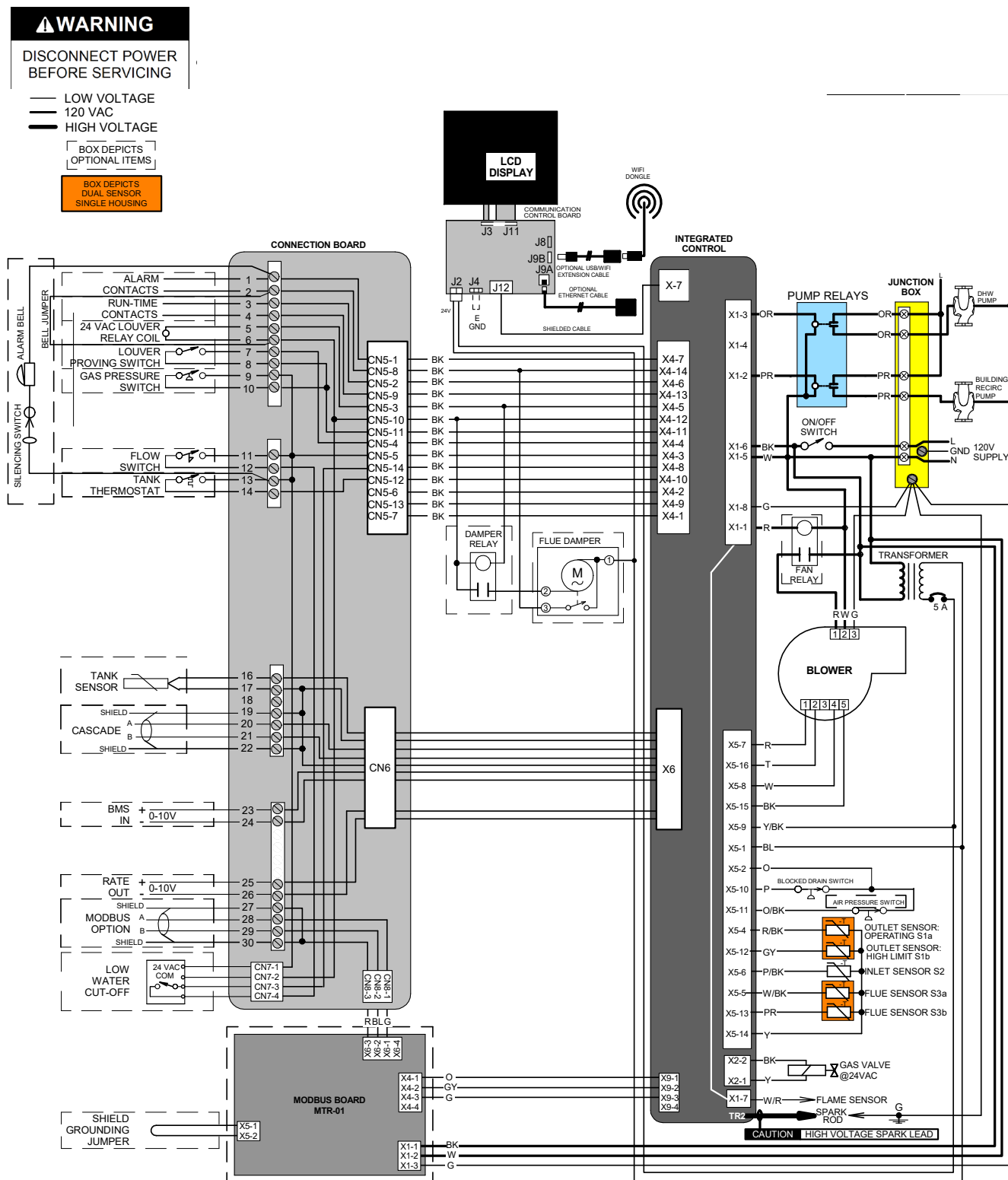
Figure 13-2 Schéma de câblage
