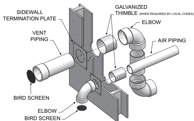
Figure 4-5C Terminaisons murales typiques - PVC/CPVC ou inox
