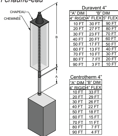
Figure 3-8 Conduit d'évacuation flexible en polypropylène à proximité d'un chauffe-eau
