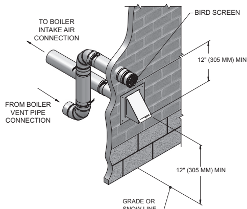
Figure 4-1C Terminaisons d'apport d'air et d'évacuation murales optionnelles en PVC/CPVC/inox (non fournies)
