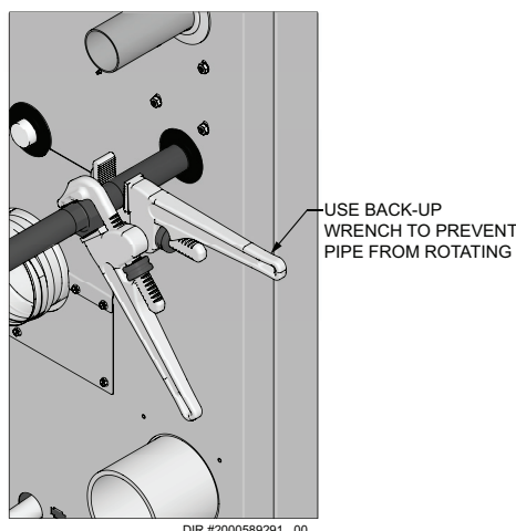
Figure 8-2 Raccord d'entrée de gaz retenu par une clé
