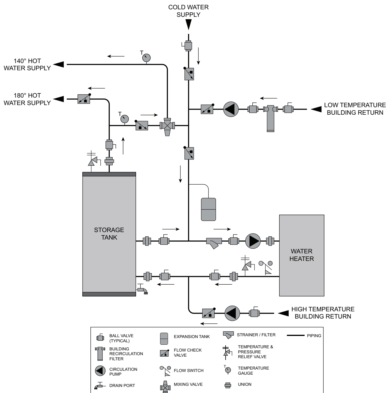
Figure 7-4 Un chauffe-eau, un réservoir (2 températures)
