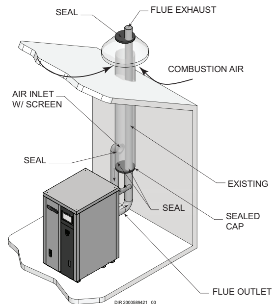
Figure 5-9 Ventilation concentrique, exemple 2
