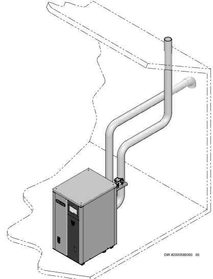
Figure 3-5 Évacuation verticale, apport d'air mural
