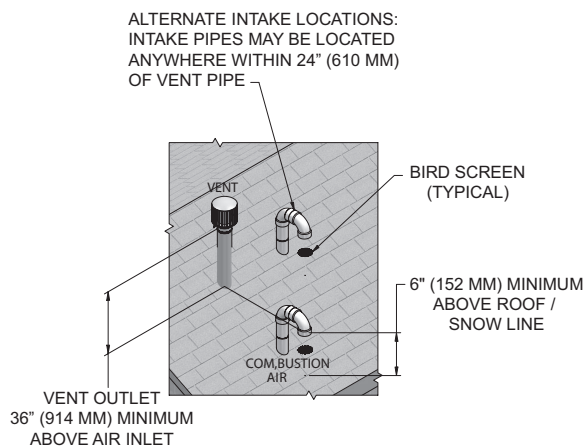
Figure 5-1B Terminaisons verticales d'apport d'air et d'évacuation en acier inoxydable
