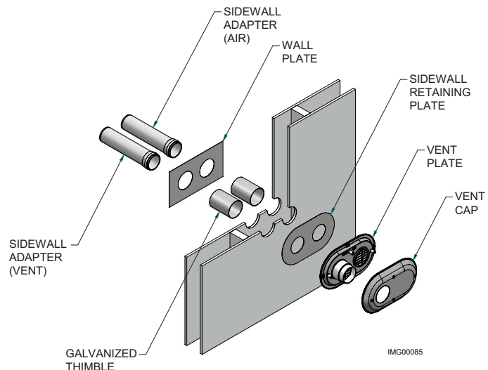
Figure 4-5B Terminaison murale en polypropylène
