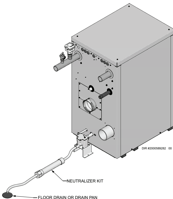
Figure 10-1 Évacuation de la condensation
