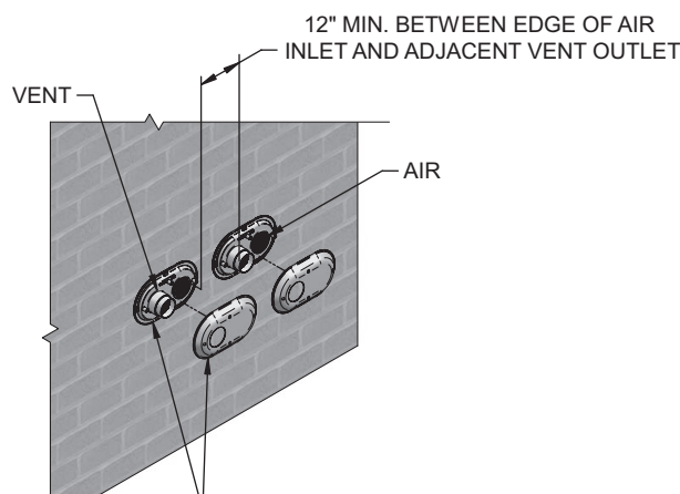
Figure 4-6A Plusieurs terminaisons murales (doit aussi être conforme à Figure 4-1A)
