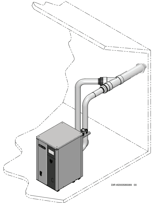
Figure 3-2 Terminaison concentrique murale en PVC/CPVC
