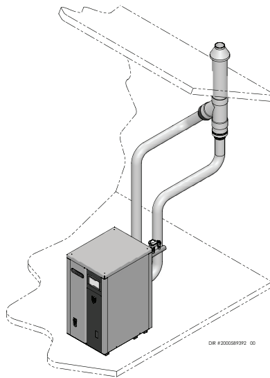
Figure 3-4 Terminaison concentrique verticale en PVC/CPVC
