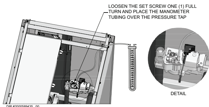
Figure 8-4 Vérification de la pression d'entrée - Modèles 650-1000
