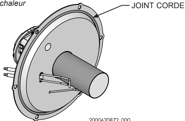
Figure 13-3 Joint torique - Porte de l'échangeur de chaleur
