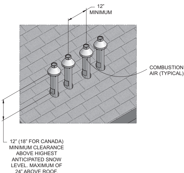
Figure 5-7 Terminaison concentrique, apport d'air et évacuation
