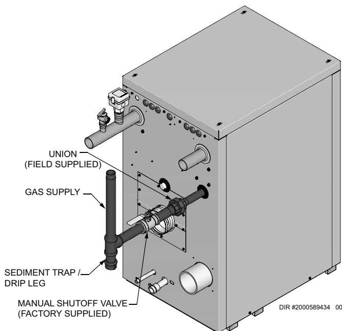
Figure 8-1 Conduites d'alimentation en gaz
