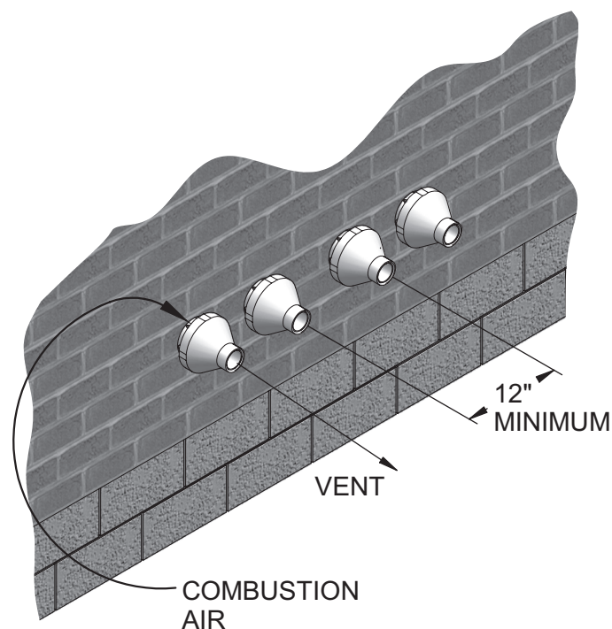
Figure 4-12 Terminaison concentrique, apport d'air et évacuation
