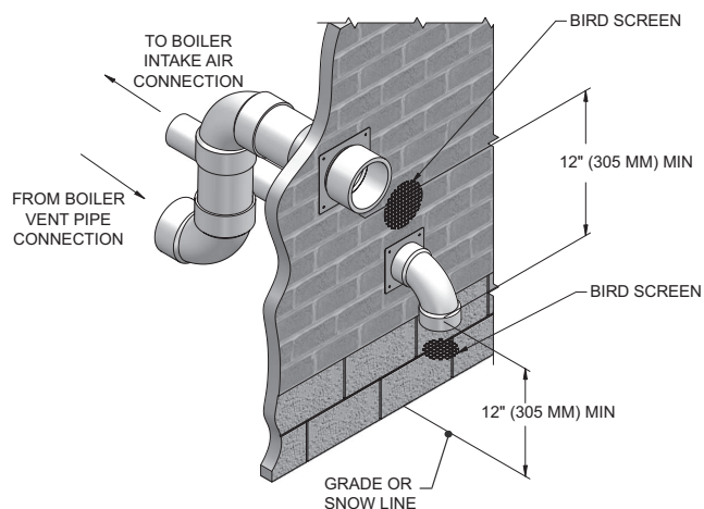
Figure 4-2 Terminaisons murales optionnelles en PVC/CPVC/inox./polypropylène (non fournies)
