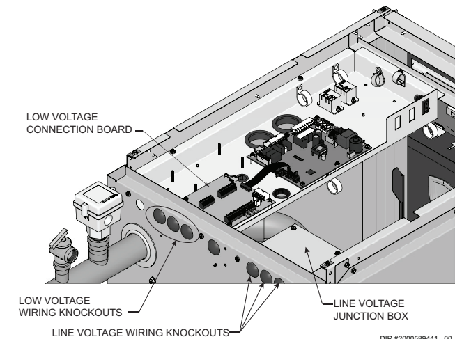
Figure 9-2 Câblage réalisé au chantier
