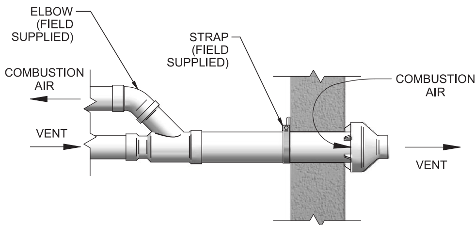
Figure 4-11 Fixation d'une terminaison concentrique murale
