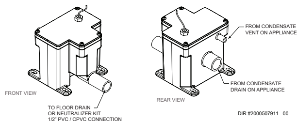
Figure 13 Collecteur de condensation
