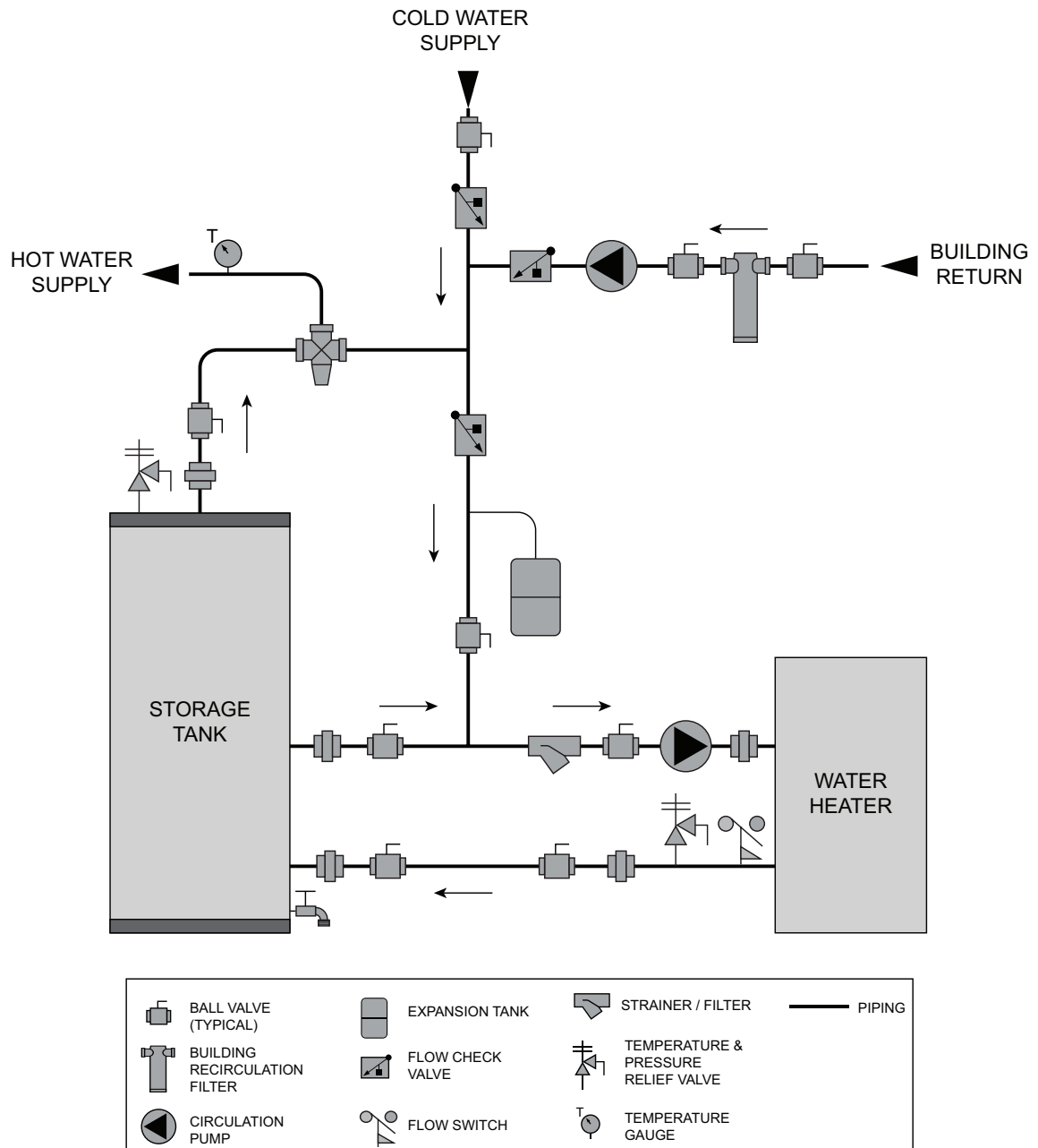
Figure 7-3 Un chauffe-eau, un réservoir
