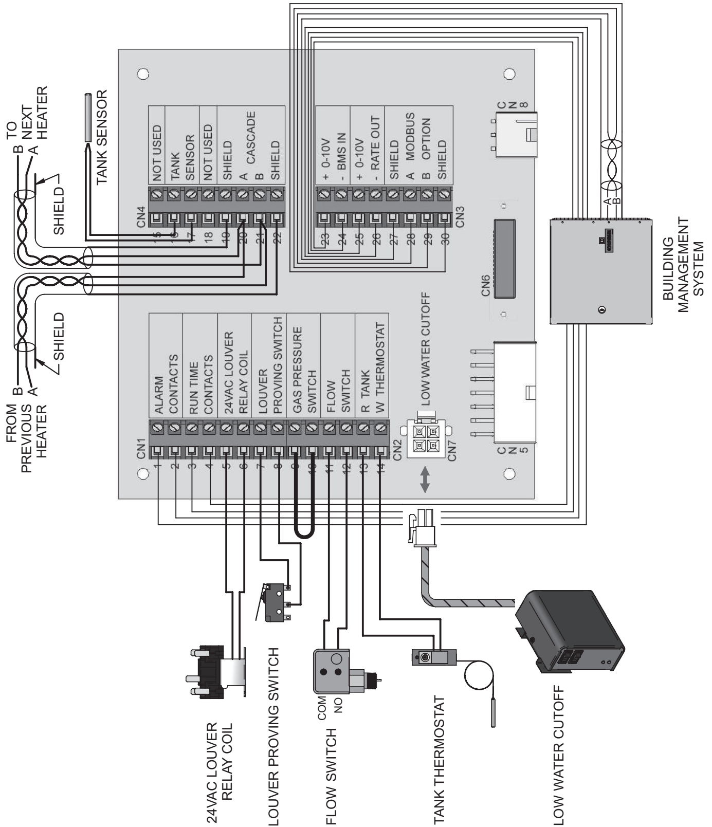
Figure 9-3 Raccords basse tension au chantier
