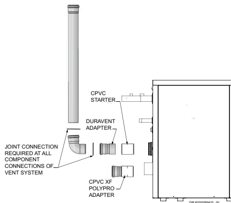
Figure 3-9 Conduit d'évacuation en polypropylène à proximité d'un chauffe-eau
