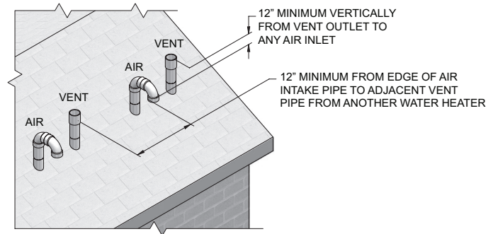
Figure 5-3 Terminaisons verticales optionnelles, plusieurs chauffe-eau
