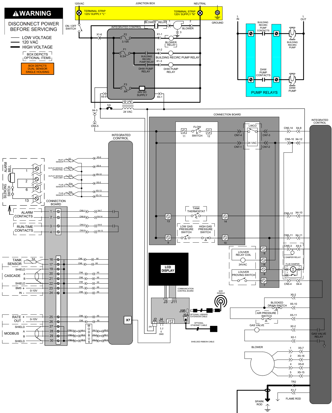
Figure 13-1 Schéma électrique
