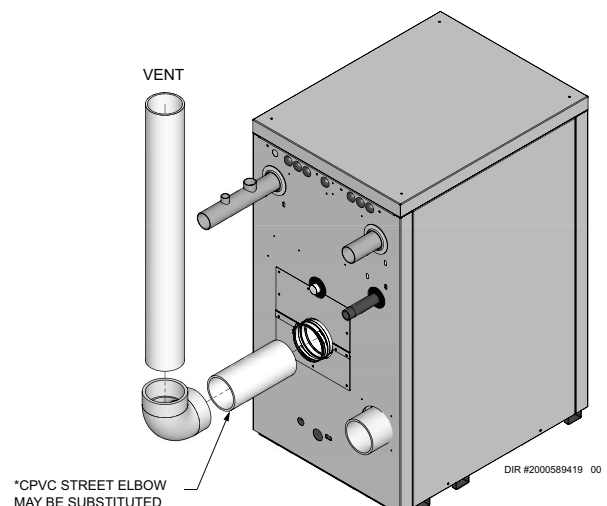
Figure 3-7 Tuyauterie d'évacuation en PVC/CPVC à proximité du chauffe-eau - Modèles 400 - 1000
