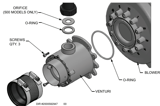
Figure 2-2a Installation d'un orifice au propane - Modèles 400-500
