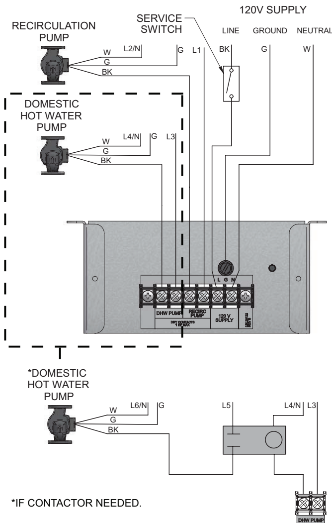
Figure 9-1 Raccords basse tension au chantier - Avec et sans contacteur
