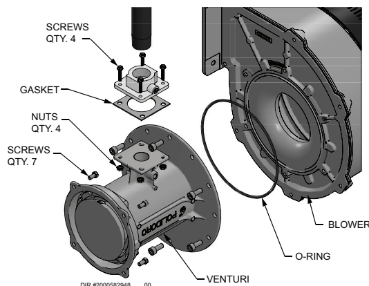
Figure 2-2b Installation d'un orifice au propane - Modèles 650-1000
