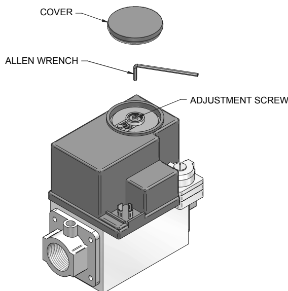
Figure 2-4 Réglage de la vanne du gaz: modèles 400 et 500
