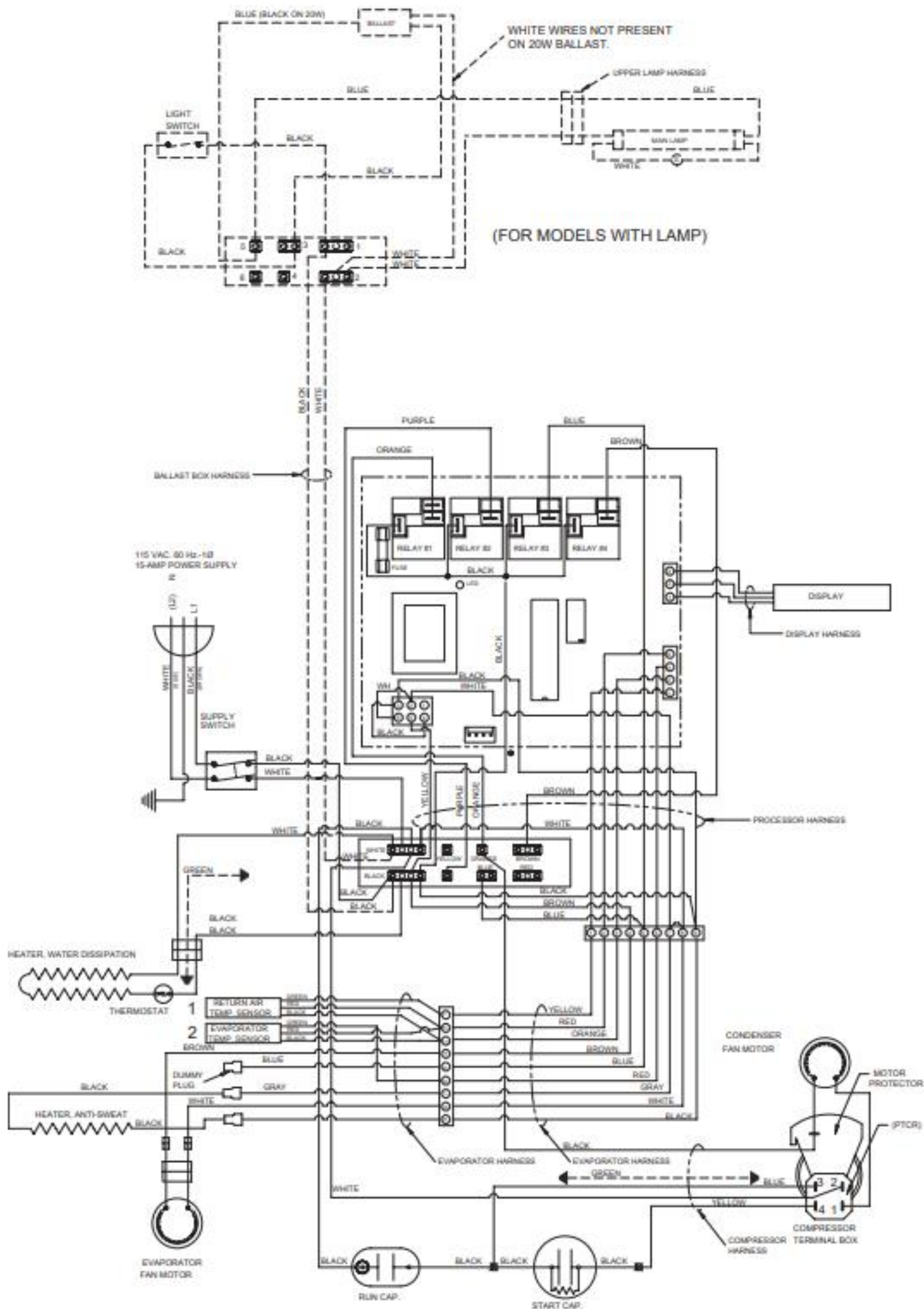
WIRING DIAGRAM-OPEN, MED-TEMP. 00-0219-00
