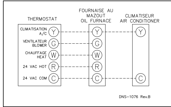
Figure 3: Branchement du thermostat, chauffage et climatisation, unité avec moteur ECM
