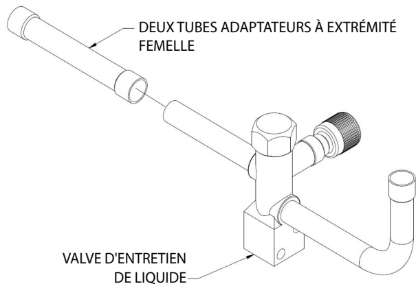
Figure 6 – Valve de service de liquide de climatisation standard A200112
