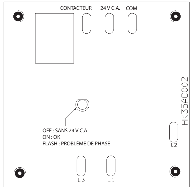
Figure 11 – Commande de moniteur triphasé (s'applique aux appareils triphasés seulement)
