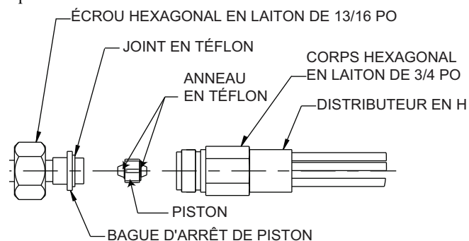
Figure 7 – Installation du piston intérieur A10342
