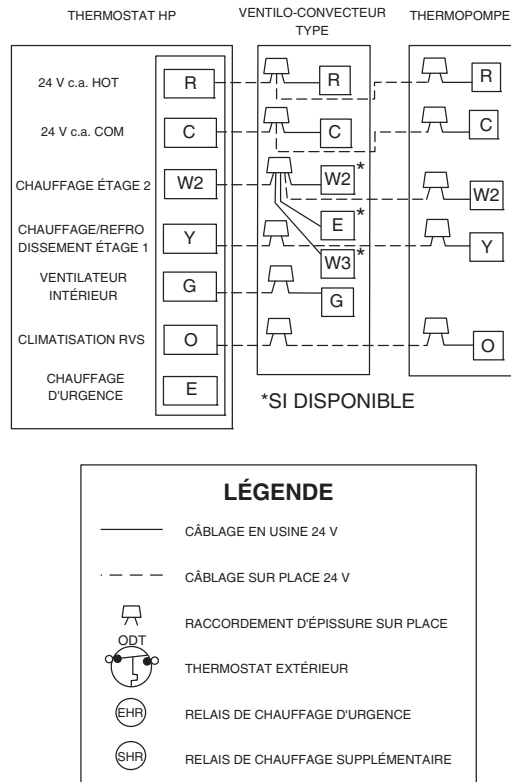
Figure 12 – Schémas de câblage génériques (consultez les instructions d'installation du thermostat pour connaître les combinaisons spécifiques des appareils)
