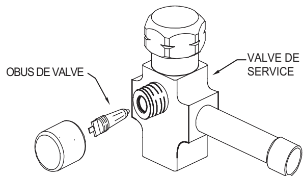
Figure 5 – Valve de service de vapeur
