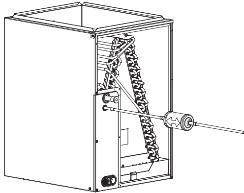
Figure 8 – Déshydrateur-filtre de la conduite de liquide
