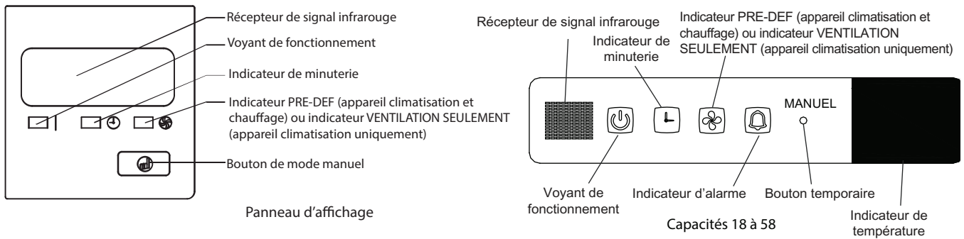
Fig. 3 – Panneau d’affichage du récepteur infrarouge (IR)
