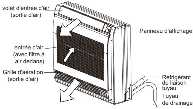
Fig. 1 – Capacité 12K
