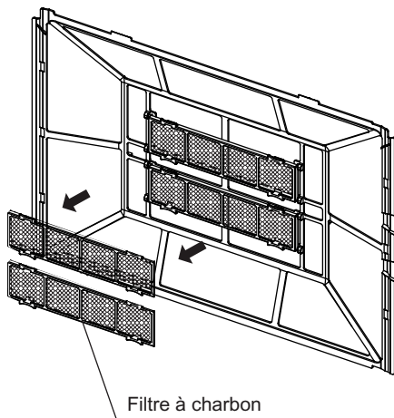
Fig. 31 – Filtre à charbon
