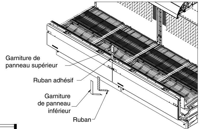
COMPTOIR RÉFRIGÉRÉ 3
