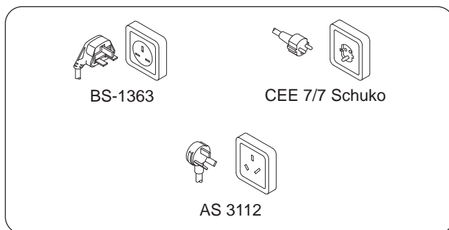
Stekkerconfiguraties
