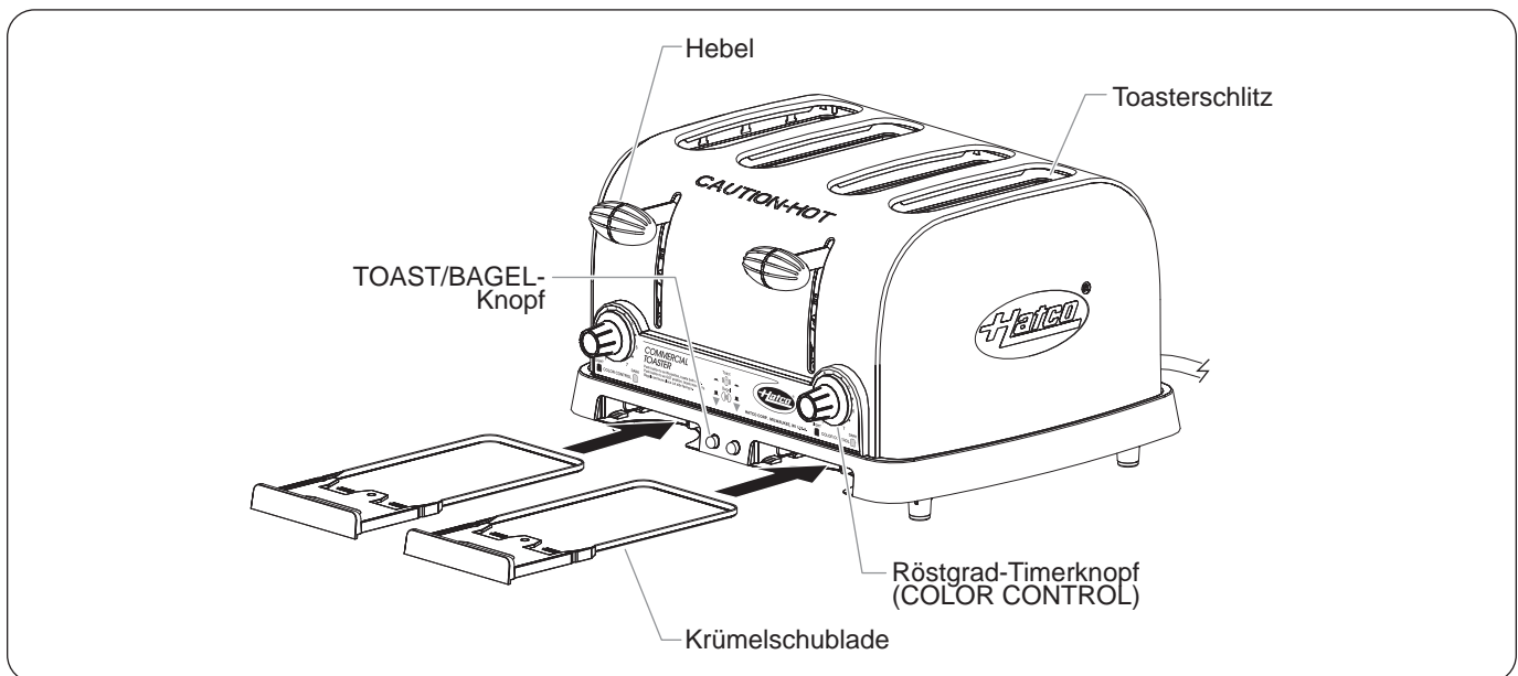
Komponenten
