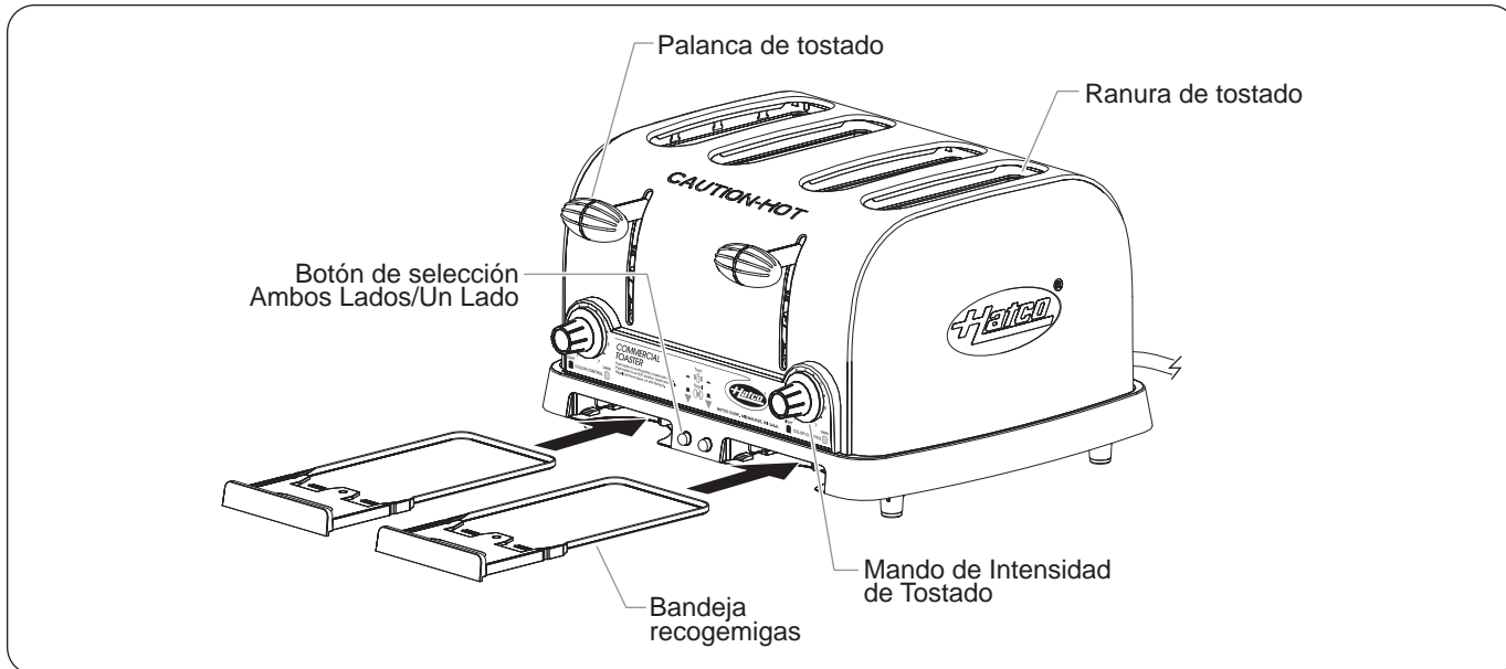
Componentes
