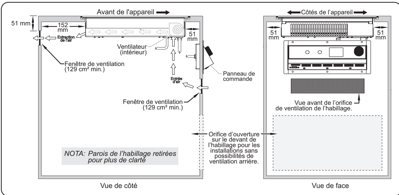
Distances minimales de montage pour les modèles à encastrer
