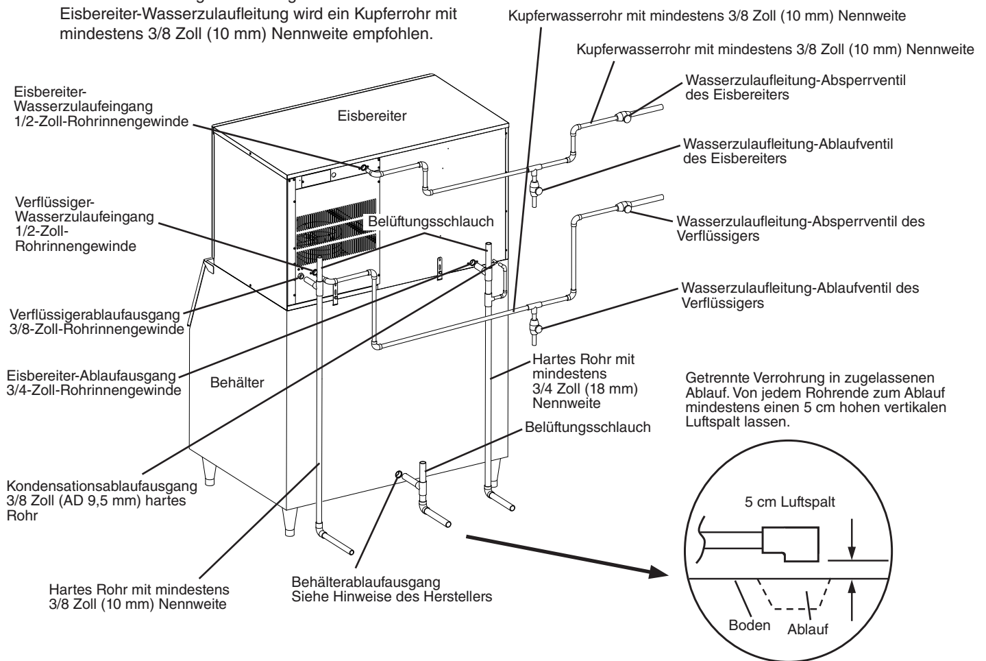
KM-1301SWJ-E Anschluss an ein offenes Ablaufsystem
