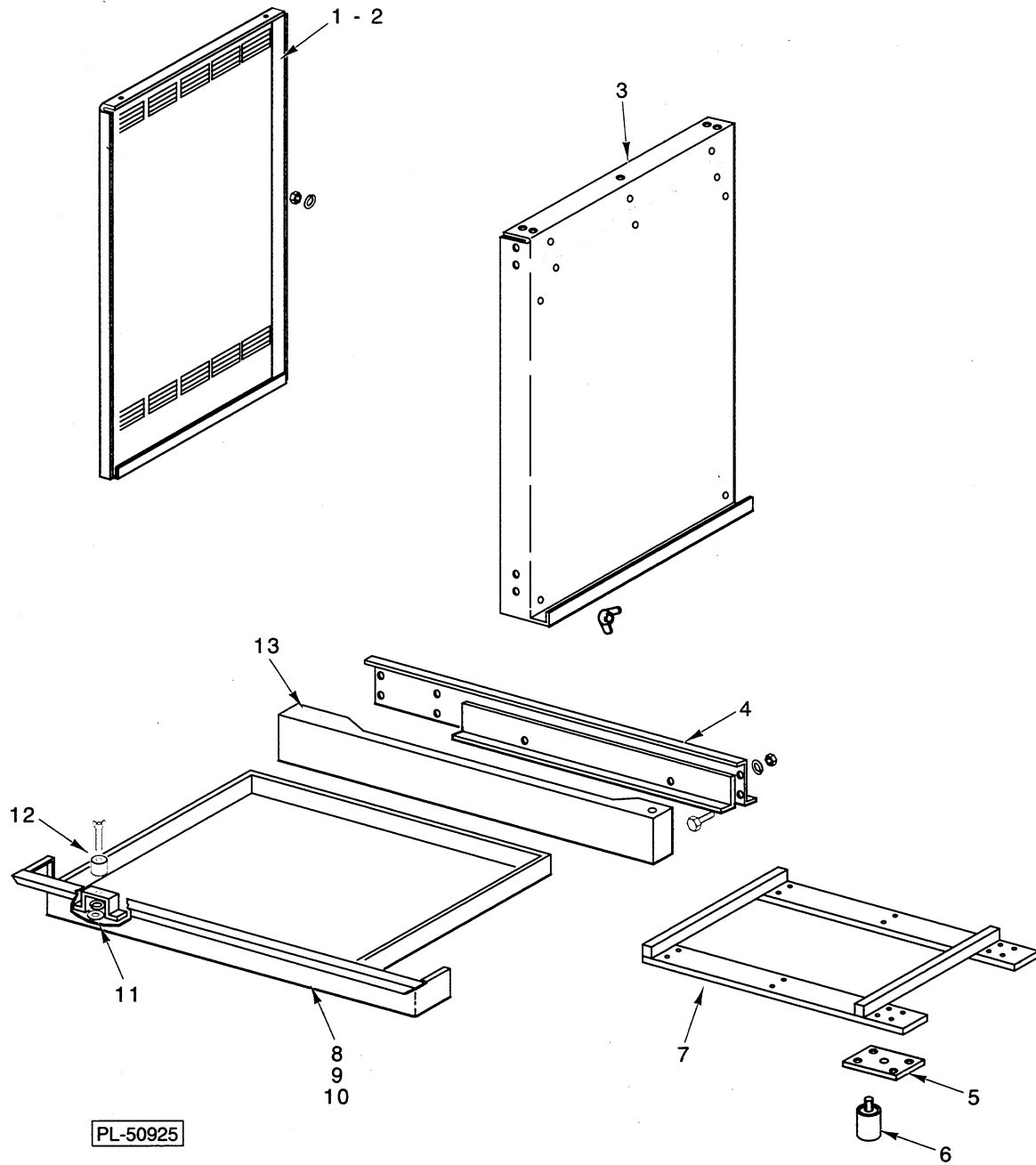
OVEN (L.H. SIDE)
