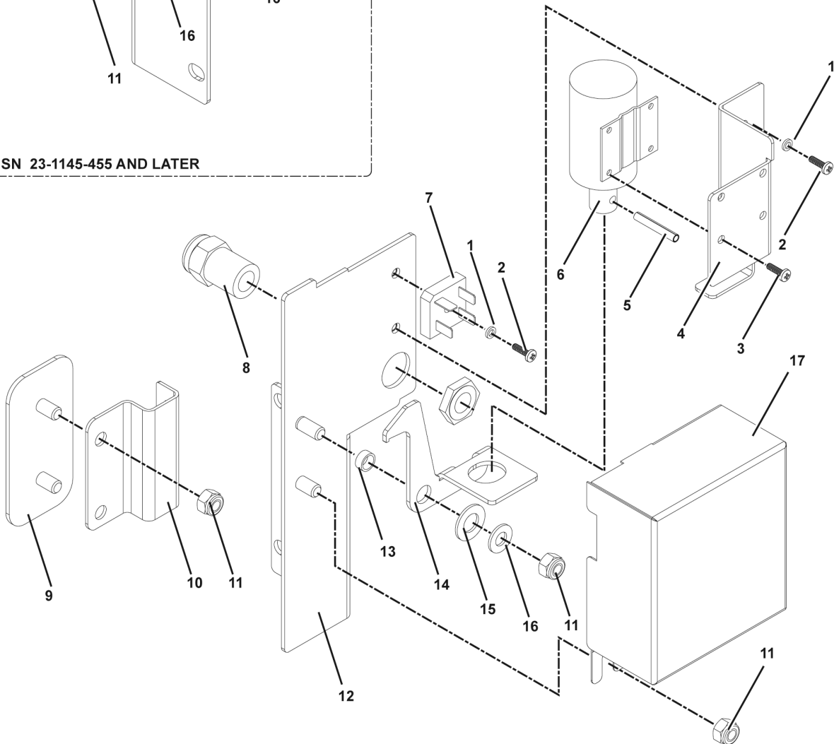
DOOR LOCK (AM15VL)
