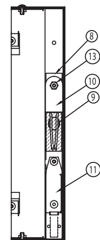
SECTION B-B ÉCHELLE 1:2
