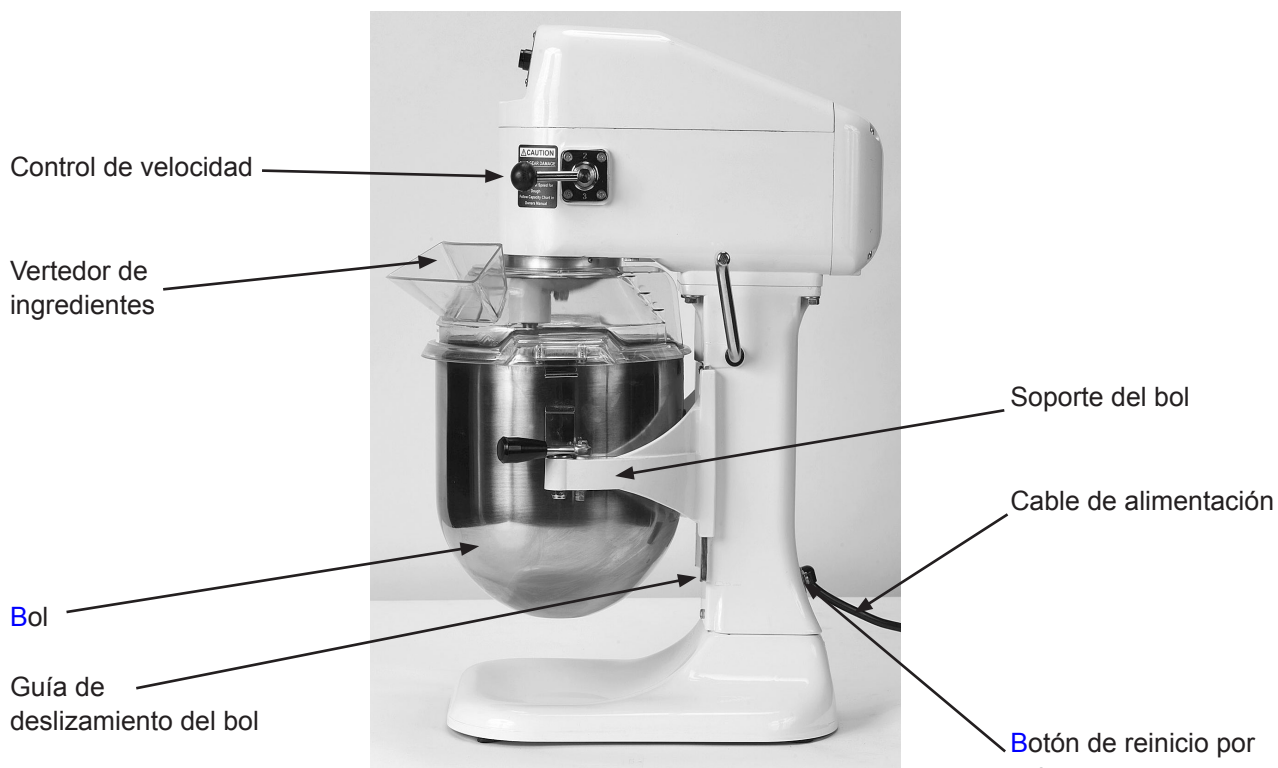
VISTA LATERAL
