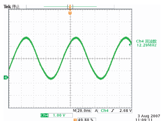
(C) Wave form 3 : CLOCK Waveform (12.288MHz) 波形3: クロック波形 (12.288MHz) X301 (Refer to the SCHEMATIC DIAGRAMS 3/7) (SCHEMATIC DIAGRAMS 3/7を参照)
