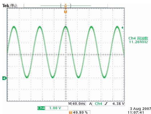
(B) Wave form 2 : CLOCK Waveform (11.2896MHz) 波形2: クロック波形 (11.2896MHz) X302 (Refer to the SCHEMATIC DIAGRAMS 3/7) (SCHEMATIC DIAGRAMS 3/7を参照)
