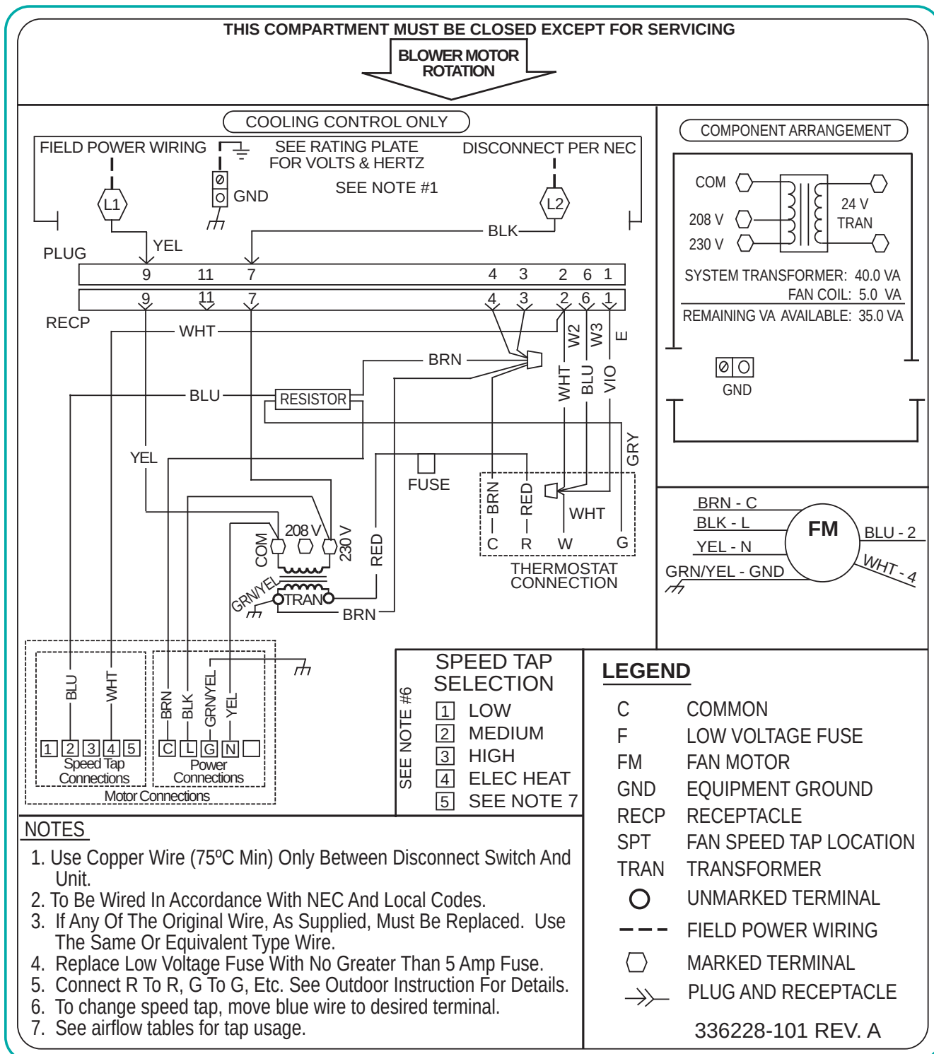
Fig. 18 - 336228-101
