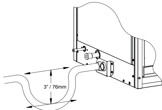
Fig. 6 - Condensate Trap
