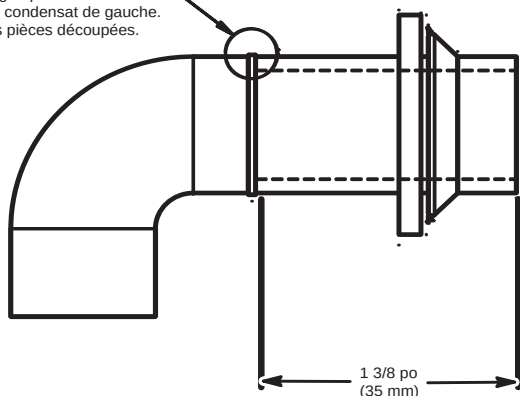
Fig. 16 – Modification du coude d'évacuation en caoutchouc
