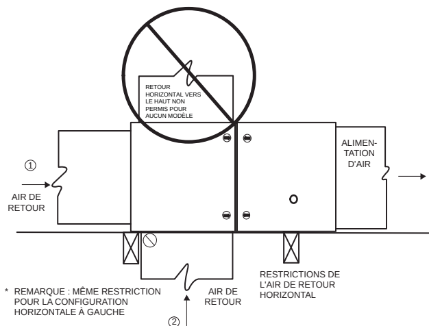
Fig. 28 – Configurations et restrictions des conduits de reprise horizontaux
