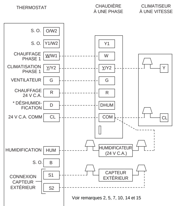
Chaudière à une phase avec climatiser à une phase
