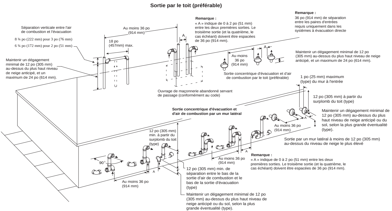
Fig. 52 – Air de combustion et sortie d'évent pour système d'évacuation directe (2 tuyaux)
