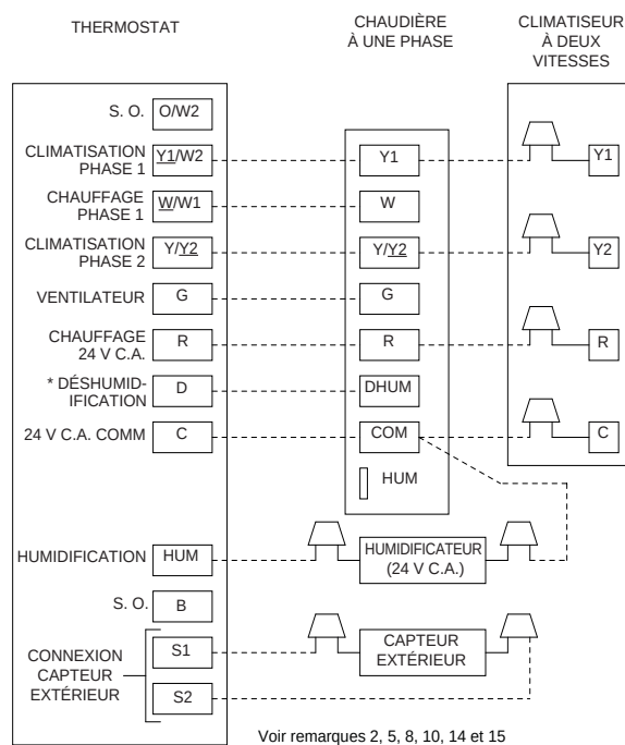
Chaudière à une phase avec climatiser à deux phases
