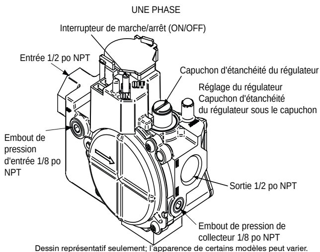
Capacité standard de la valve à gaz sans orifices de pression de tour
