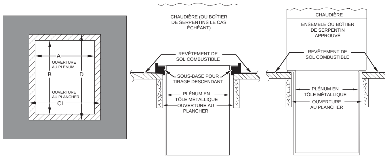
Fig. 20 – Installation sur revêtement de plancher combustible
