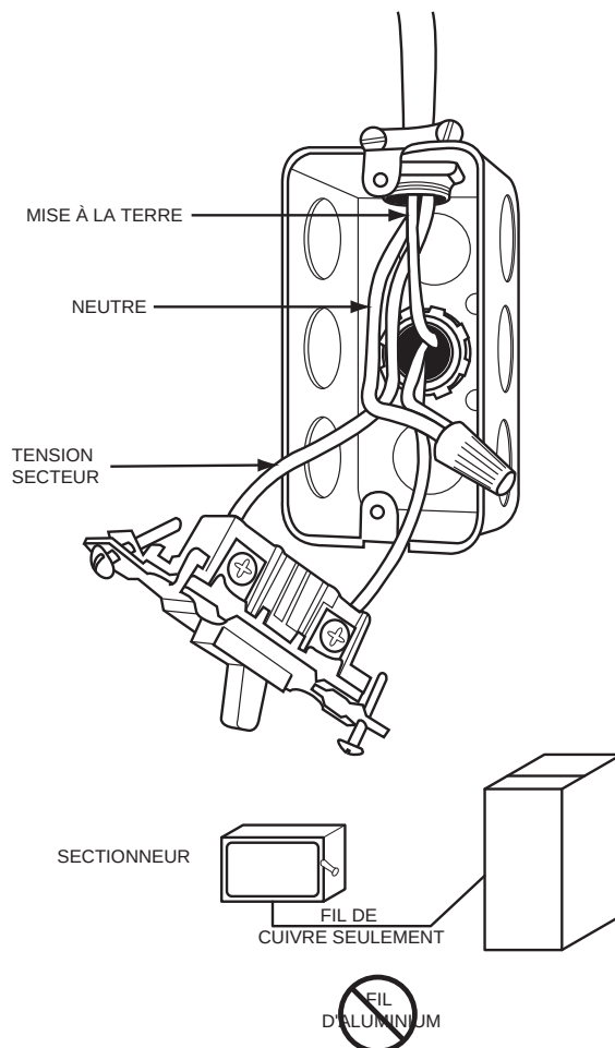
Fig. 35 – Coffret électrique externe fourni sur place sur le caisson de la chaudière
