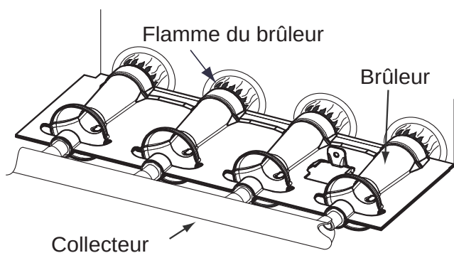
Fig. 66 – Flamme du brûleur
