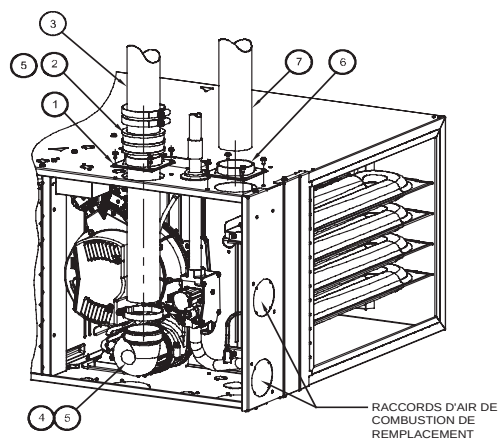
CONFIGURATION HORIZONTALE À DROITE ET VENTILATION VERTICALE
