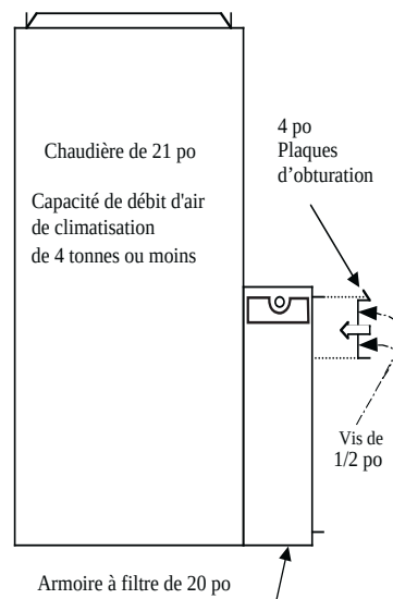
Option d'installation d'armoire à filtre pour capacité de climatisation de 4 tonnes ou moins
