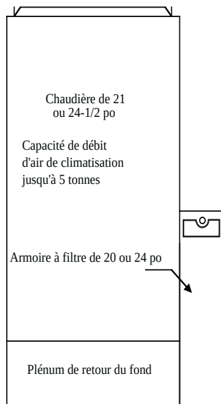
Installation d'armoire à filtre de 20 ou 24 po pour combinaison de retour sur le côté et au fond
