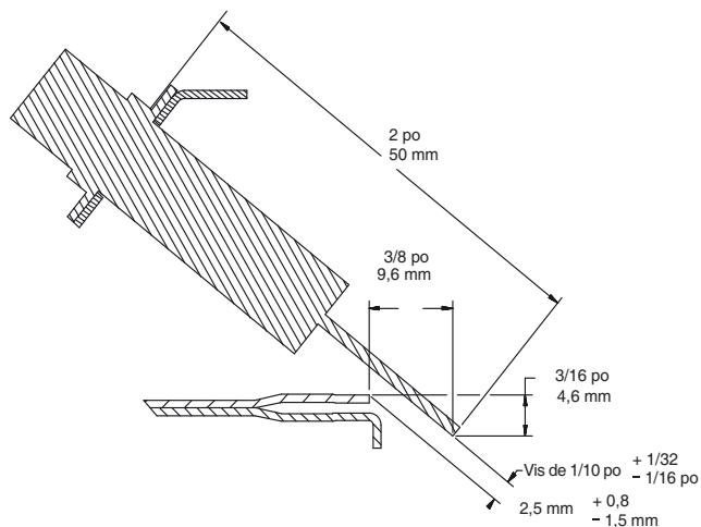
Fig. 63 – Position de l'allumeur— vue de côté
