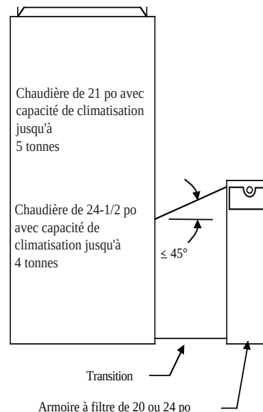
Installation d'armoire à filtre de 20 ou 24 po avec transition en angle
