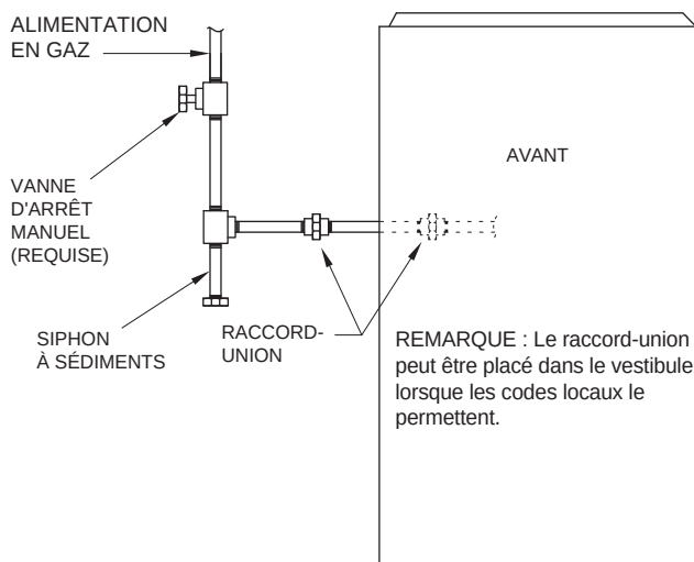
Fig. 33 – Disposition type de la tuyauterie de gaz
