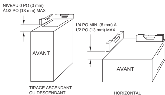
Fig. 25 – Exigences d'inclinaison de la chaudière
