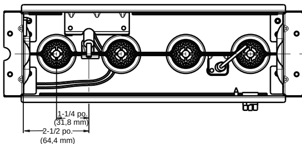
Fig. 57 - Position de l'allumeur - vue de haut
