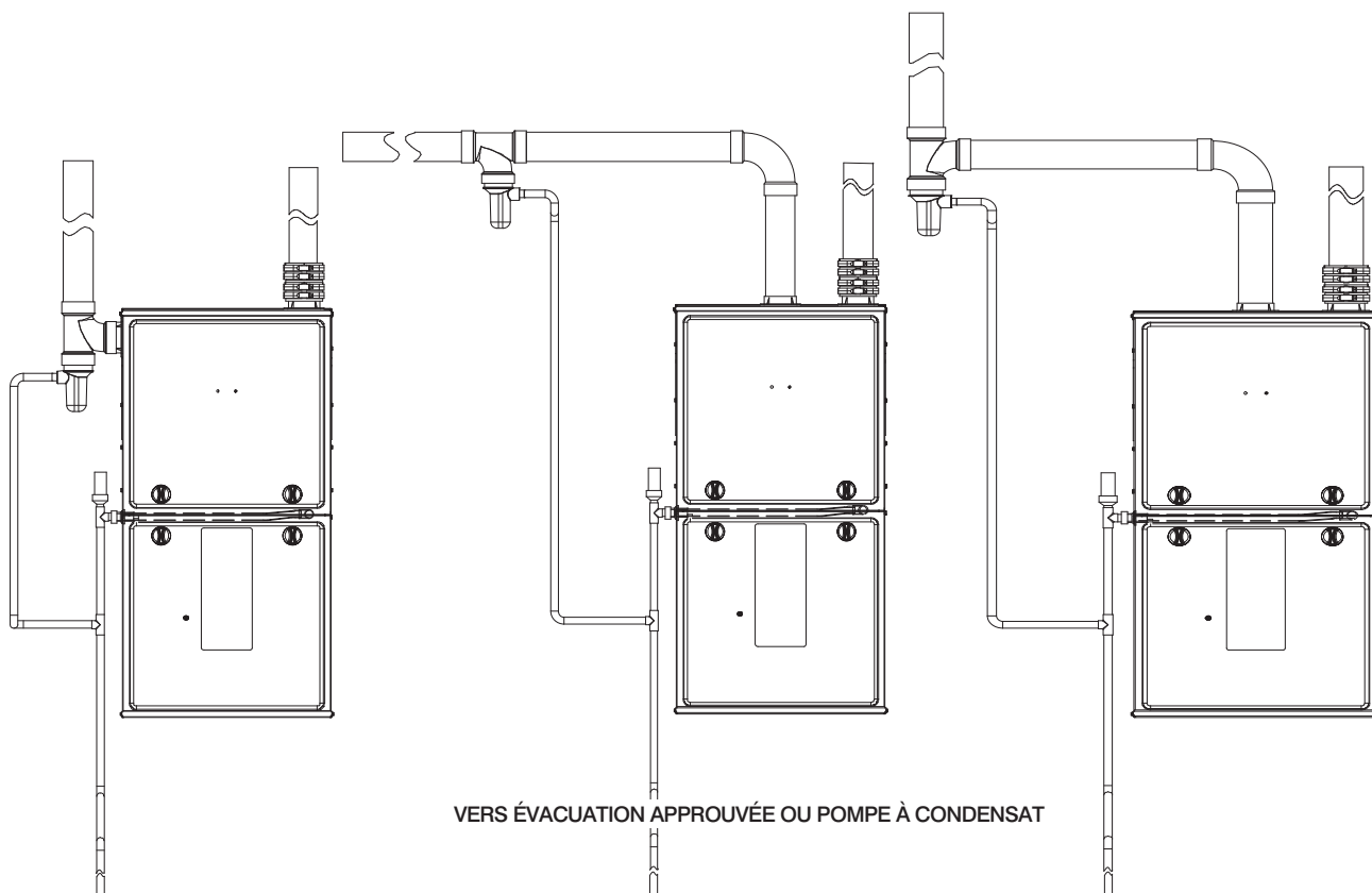
Fig. 51 - Exemple de raccord de tuyau de prise d'air pour les systèmes d'évacuation en polypropylène
