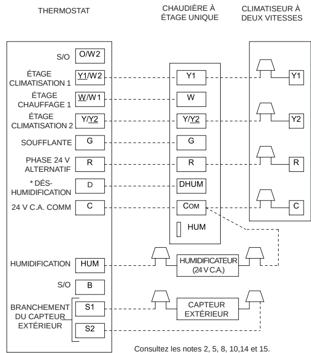
Chaudière à étage unique avec climatiseur à deux vitesses
