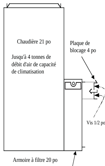
Option installation de l'armoire à filtre pour capacité de climatisation 4 tonnes ou moins
