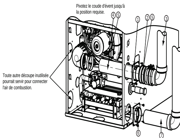
CONFIGURATION TIRAGE DESCENDANT DROITE
