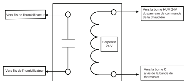
Fig. 33 - Relais d'isolation, fourni sur place, pour humidificateurs avec alimentation interne
