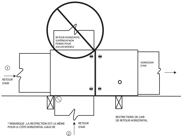
Fig. 26 - Configurations et restrictions d'air de retour, installation horizontale
