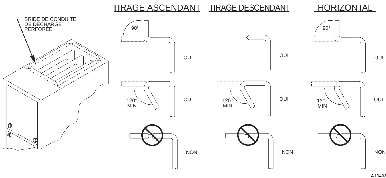
Fig. 20 - Brides d'attache de conduit
