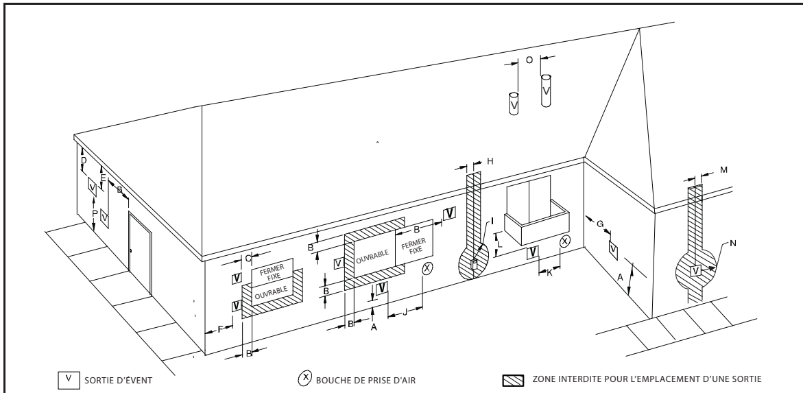
Fig. 45 - Dégagement de sortie à évacuation directe
