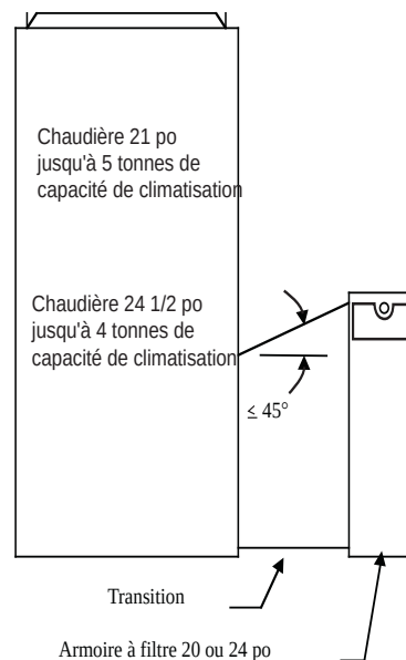
Installation de l'armoire à filtre 20 ou 24 po avec transition coudée
