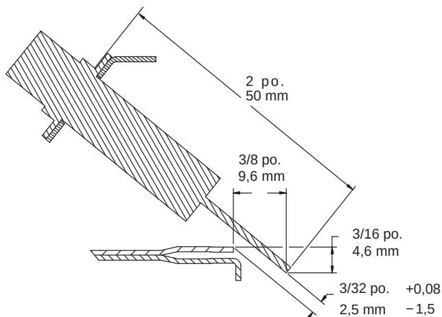
Fig. 58 - Position de l'allumeur - vue de côté
