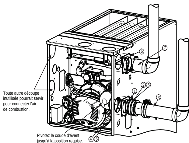
CONFIGURATION À TIRAGE ASCENDANT DROITE
