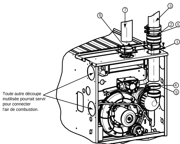
TIRAGE ASCENDANT ÉVACUATION VERTICALE
