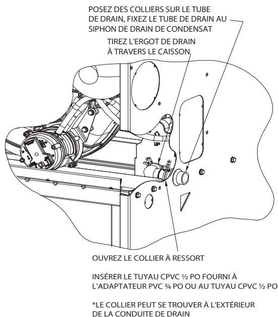
INSTALLATION DU DRAIN DU CÔTÉ DROIT
