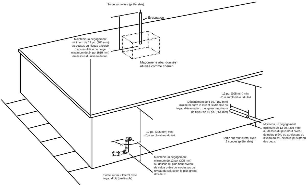
Fig. 47 – Sortie d'évent de tuyau d'air de combustion et d'évacuation pour système à évacuation directe (2 tuyaux)
