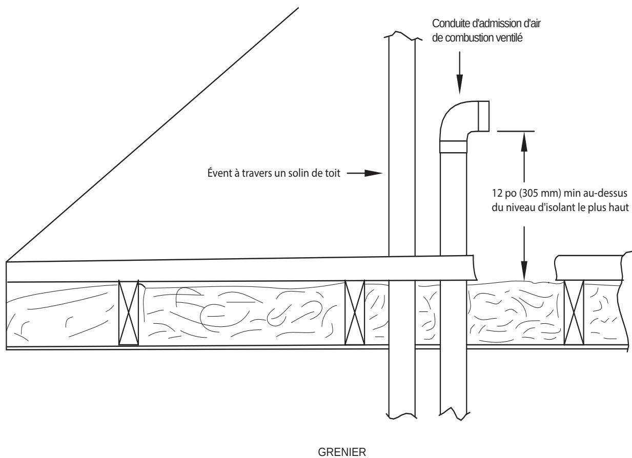
Fig. 50 - Sorties d'évent pour air de combustion ventilé
