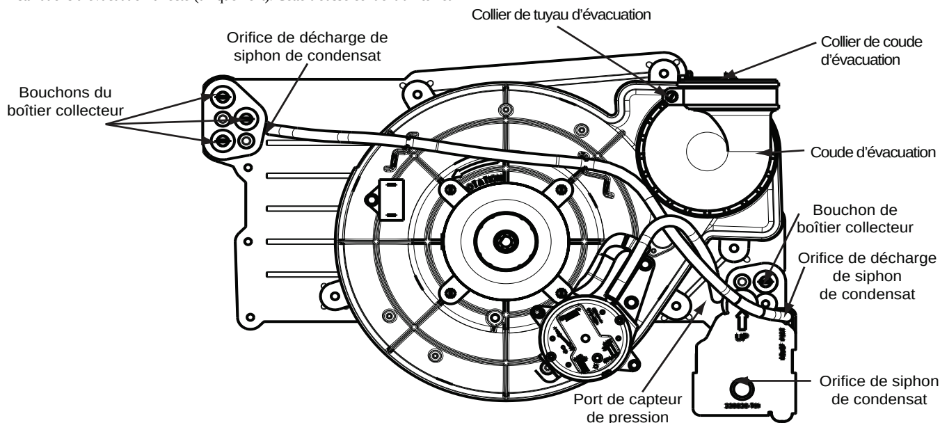
CONFIGURATION DU SIPHON POUR TIRAGE VERTICAL
