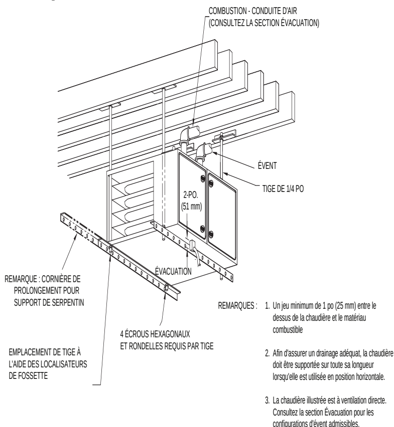
Fig. 28 - Installation de chaudière suspendue
