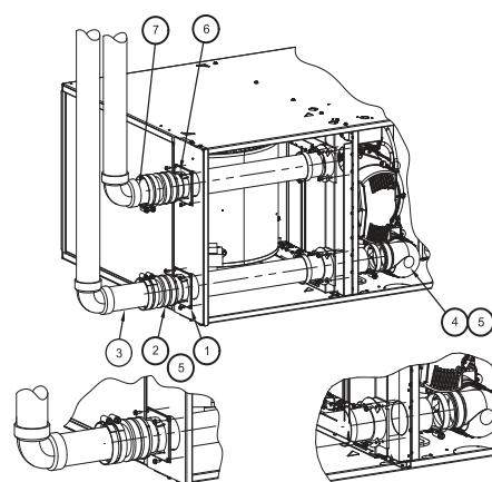
CONFIGURATION HORIZONTAL DROITE À ÉVACUATION VERTICALE
