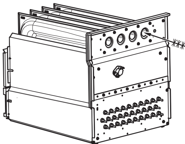
Fig. 60 - Nettoyage de la cellule de l'échangeur thermique
