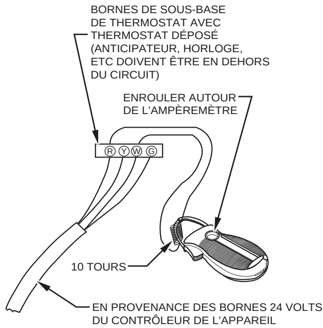
Fig. 55 - Mesure de l'appel de courant avec un ampèremètre
