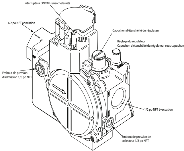
Fig. 53 - Vanne de gaz
