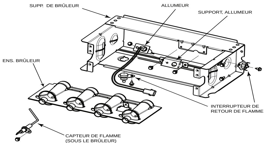
Fig. 63 - Ensemble du brûleur
