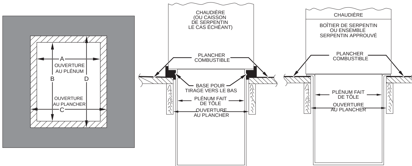
Fig. 19 - Installation sur plancher combustible
