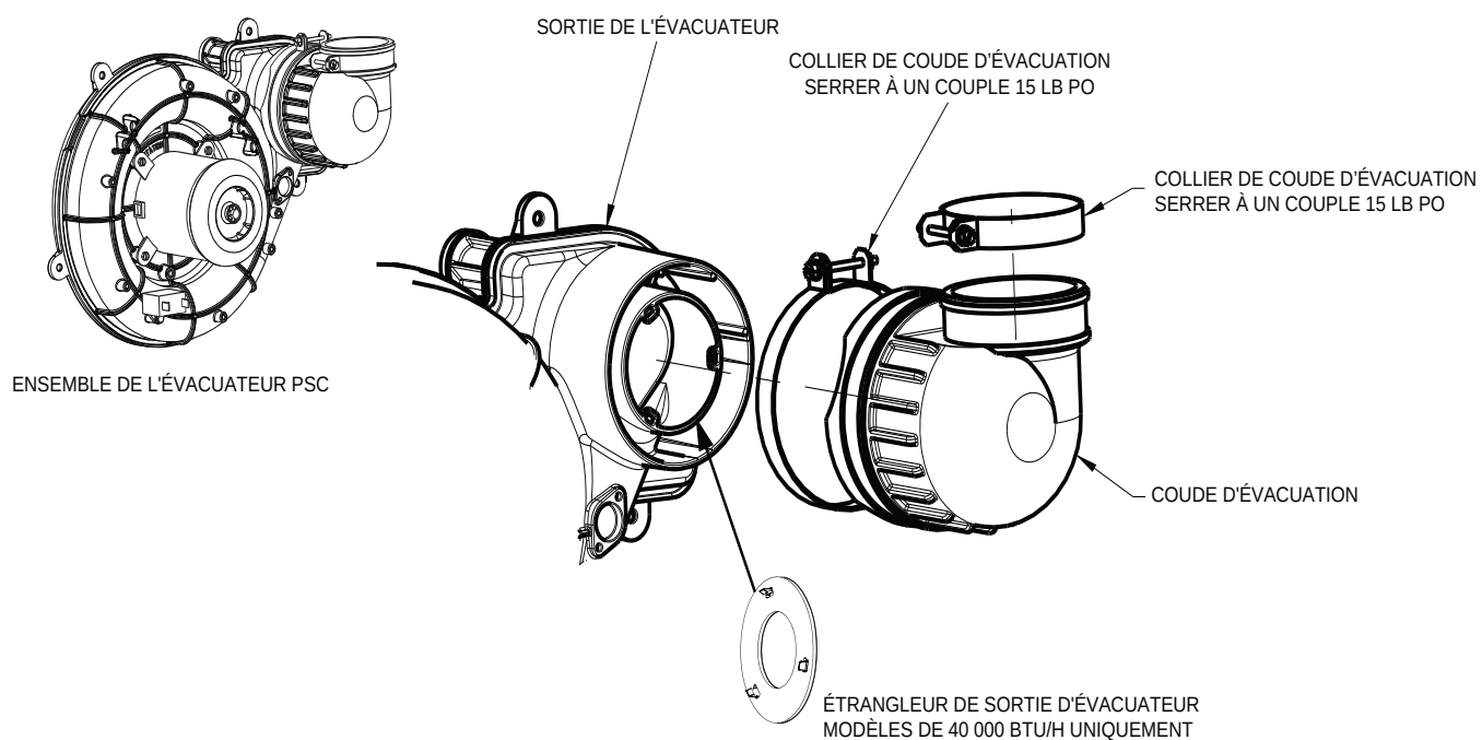
Fig. 38 - Coude d'évacuation de l'évacuateur
