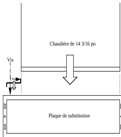
Chaudière 14 3/16 po avec plaques de substitution, décalées à droite
