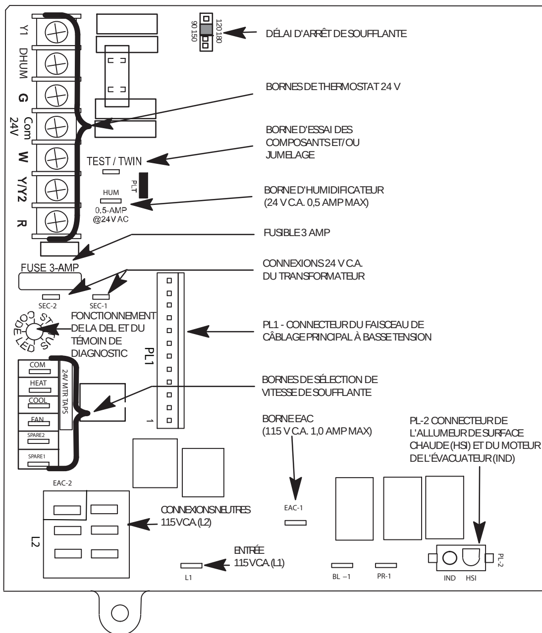
Fig. 35 - Exemple de contrôleur de chaudière à étage unique
