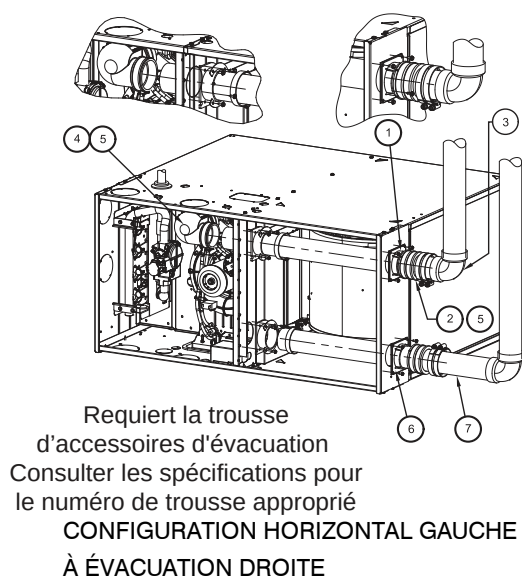
Fig. 41 - Horizontale gauche (l'apparence peut varier) Voir « remarques pour options d'évacuation »
