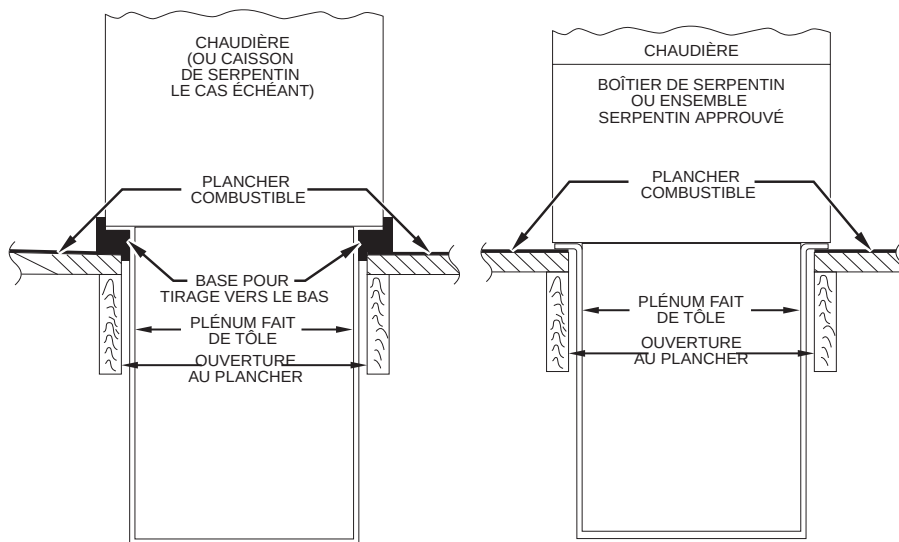
Fig. 19 - Installation sur revêtement de plancher combustible
