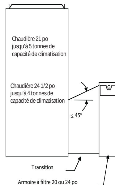
Installation de l'armoire à filtre 20 ou 24 po avec transition coudée
