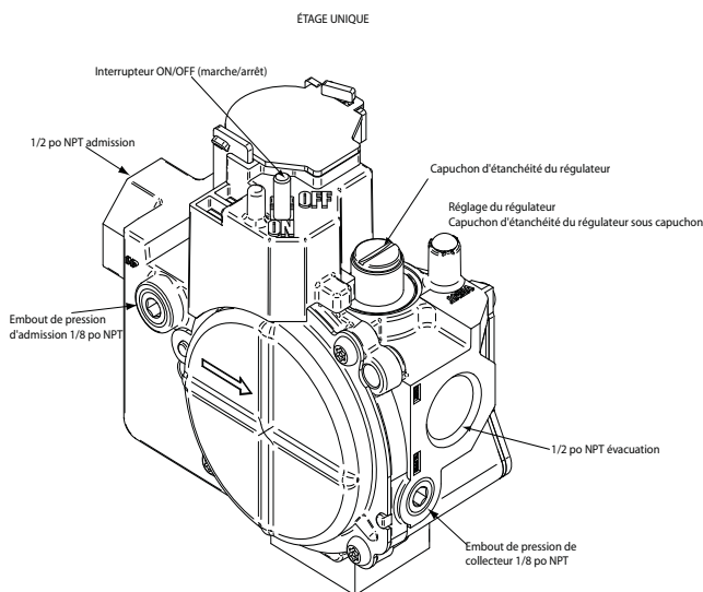
Fig. 51 – Soupape de gaz
