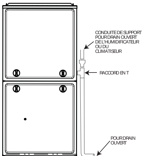
Fig. 13 - Exemple de fixation au drain sur le terrain
