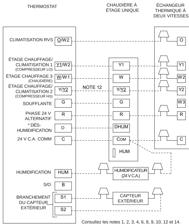
Chaudière à étage unique avec échangeur thermique à deux vitesses
