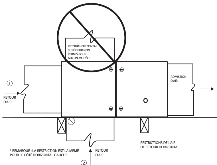
Fig. 26 - Configurations et restrictions de l'air de retour horizontal
