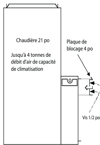
Option installation de l'armoire à filtre pour capacité de climatisation 4 tonnes ou moins
