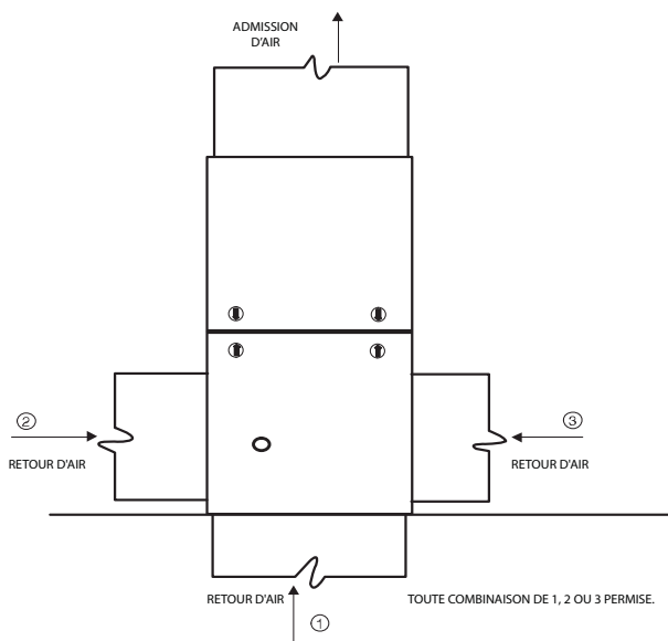
Fig. 24 - Configurations et restrictions de l'air de retour ascendant
