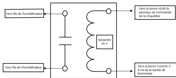
Fig. 33 - Relais d'isolation pour humidificateurs, fourni sur le site, avec bloc d'alimentation interne
