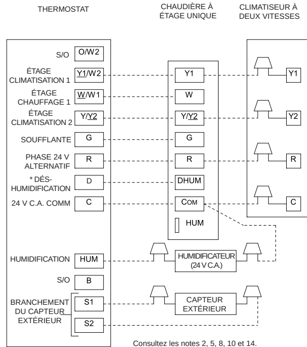
Chaudière à étage unique avec climatiseur à deux vitesses
