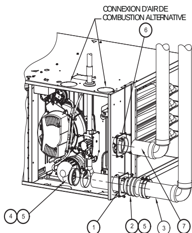
HORizontALE DROITE- CONFIGURATION À ÉVACUATION À DROITE
