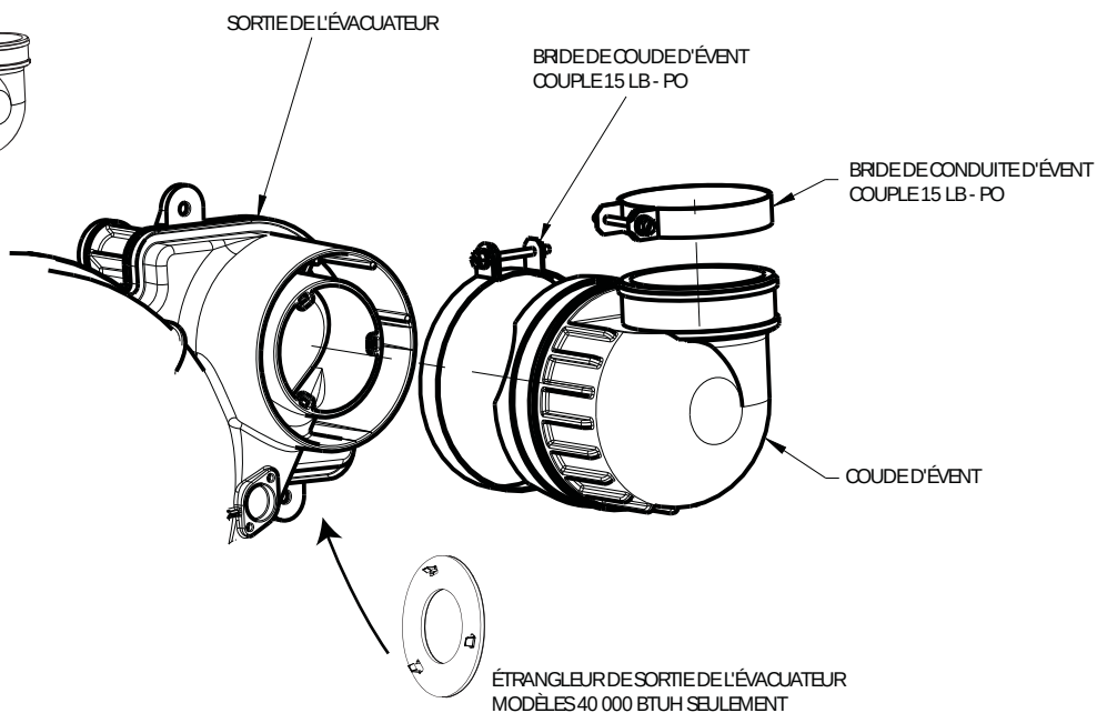
Fig. 38 - Coude d'évent d'évacuateur
