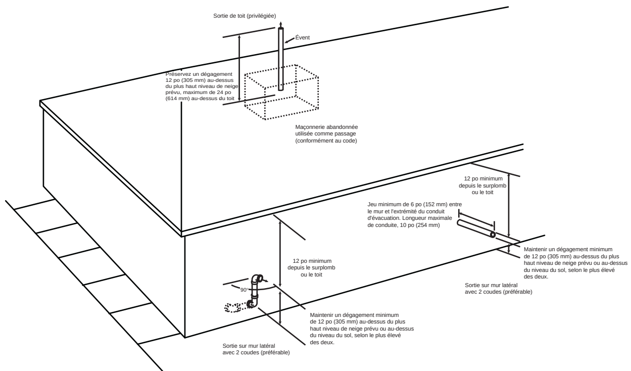
Fig. 48 - Sortie d'évent pour système d'évacuation non directe et d'air de combustion
