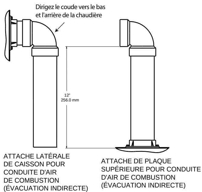
Fig. 44 - Fixation de la conduite d'air de combustion
