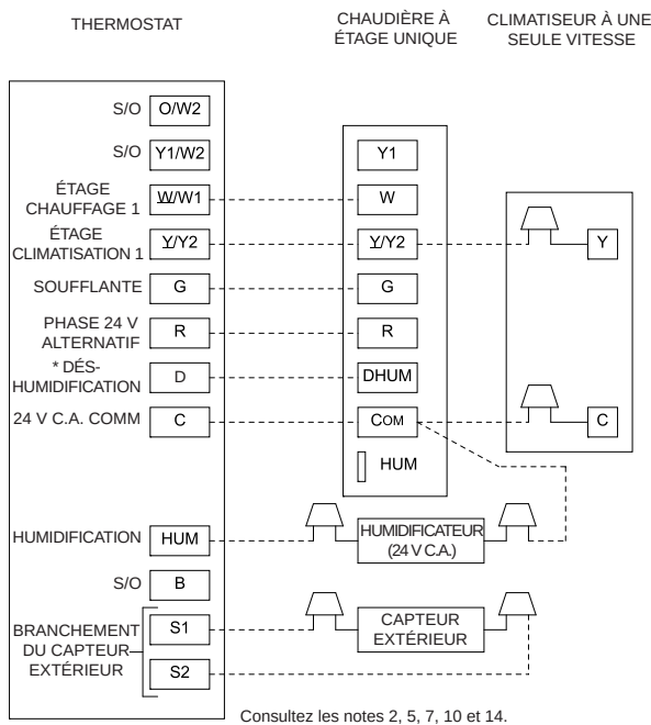
Chaudière à étage unique avec climatiseur à une seule vitesse
