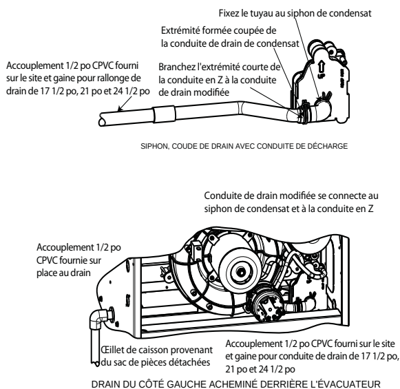
Fig. 16 - Connexion et acheminement du siphon de drain
