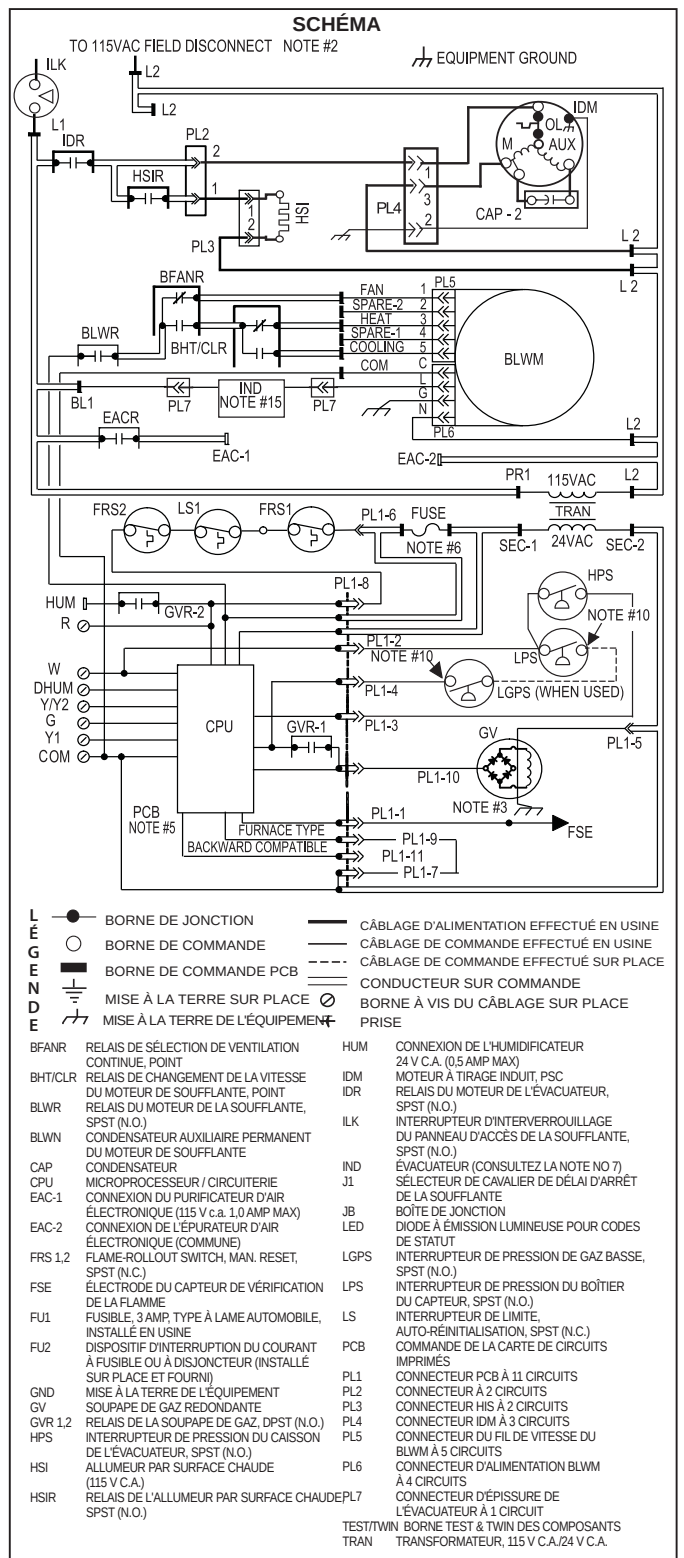
Fig. 63 - Schéma de câblage
