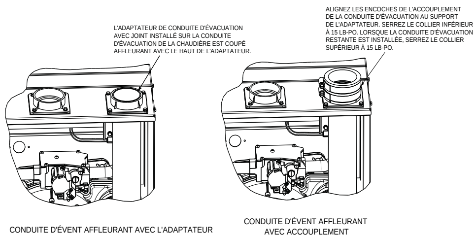
Fig. 43 - Conduite d'évent affleurant avec l'adaptateur
