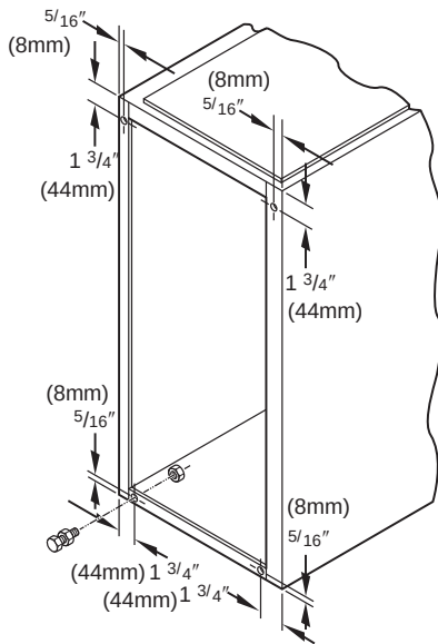
Fig. 21 - Pattes de mise à niveau
