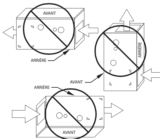
Fig. 4 - Installations prohibées
