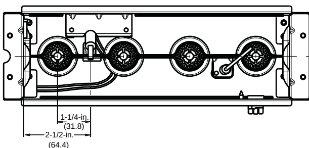
Fig. 55 - Position de l'allumeur - vue du haut
