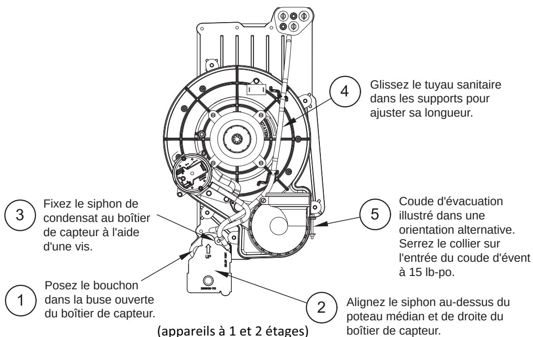
Fig. 10 - Configuration de siphon horizontal à droite
