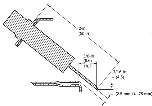
Fig. 56 - Position de l'allumeur - vue latérale
