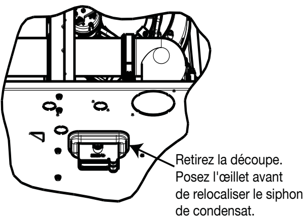
Fig. 16 - Connexion et acheminement du siphon de drain
