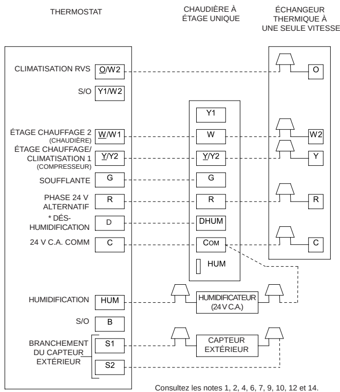
Chaudière à étage unique avec échangeur thermique à une seule vitesse
