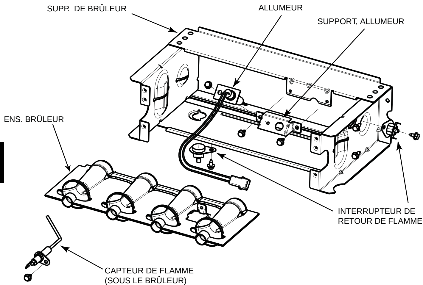
Fig. 61 - Ensemble du brûleur
