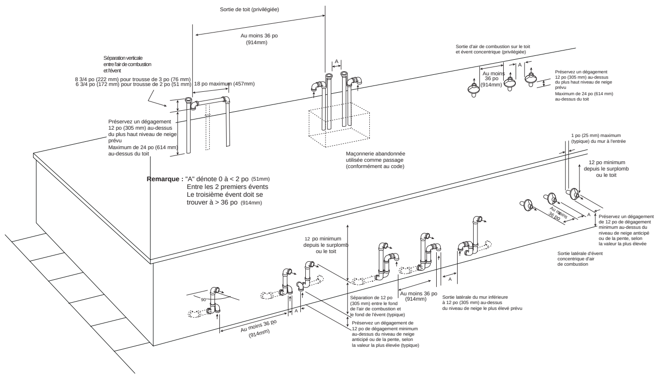
Fig. 47 - Air de combustion et sortie d'évent pour système d'évacuation directe (2 tuyaux)
