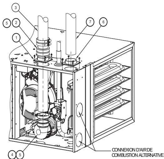
HORizontALE DROITE- CONFIGURATION À ÉVACUATION VERTICALE
