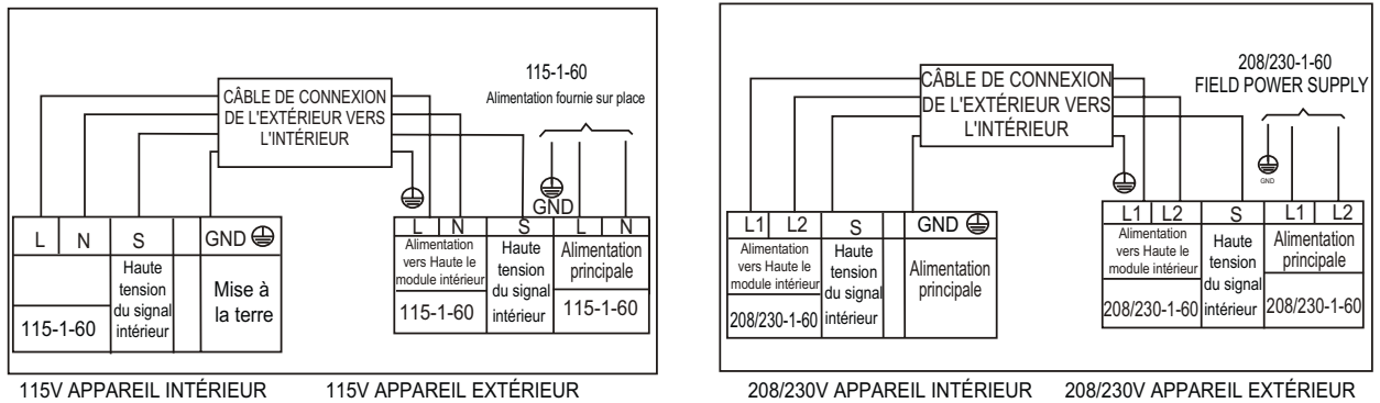
Fig. 12 — Schémas de raccordement
