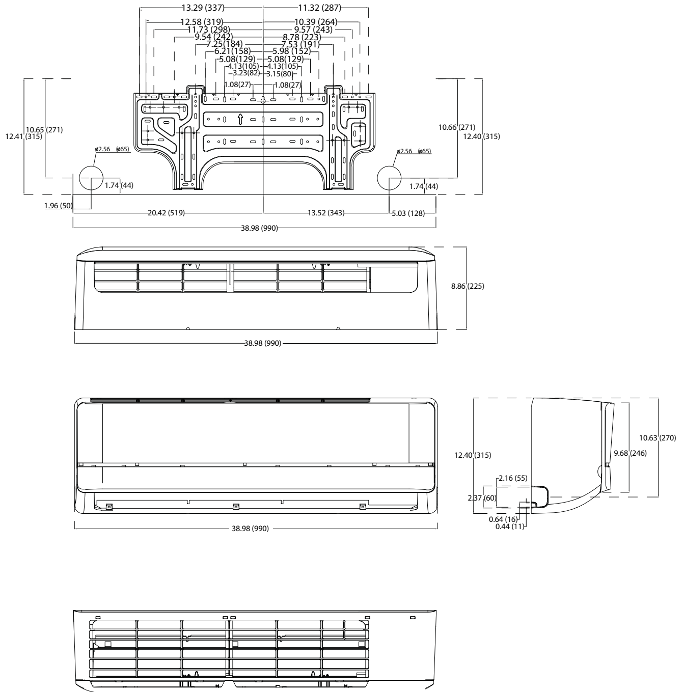
Fig. 6 — Capacité 18K
