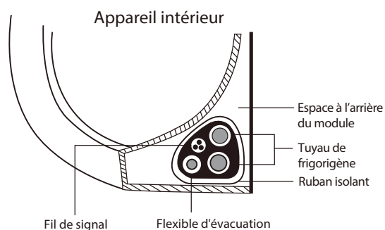
Fig. 21 — Regroupement du flexible d'évacuation, de la tuyauterie de frigorigène et du câble de signal
