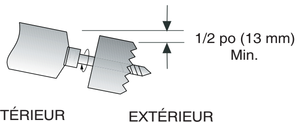
Fig. 10 — Perçage des trous
