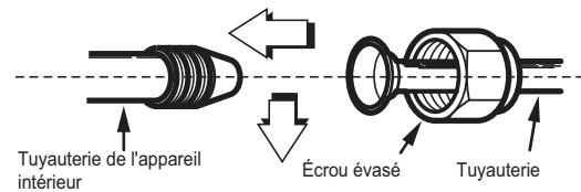
Fig. 18 — Alignez le centre du tuyau
