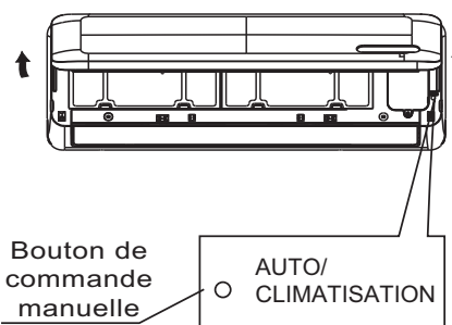
Fig. 22 — Essai de fonctionnement
