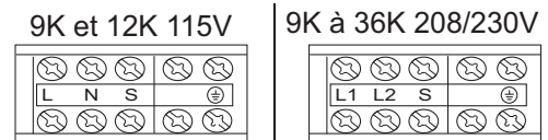
Fig. 14 — Commande et câblage électrique du module intérieur
