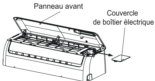
Fig. 13 — Emplacement du bloc à bornes
