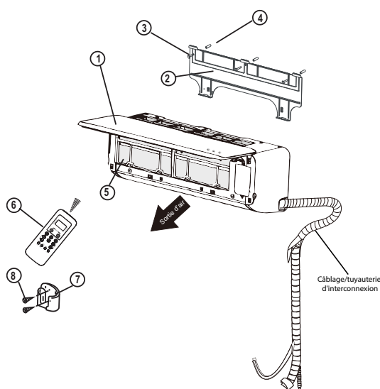
Fig. 3 — Liste de Pièces
