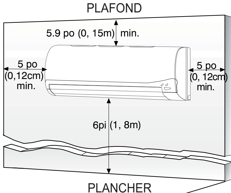
Fig. 8 — Dégagement du module intérieur
