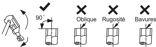
Fig. 16 — Tronçonner
