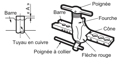
Fig. 17 — Espacement des écrous évasés
