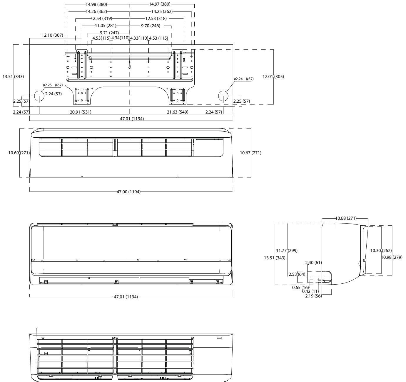
Fig. 7 — Capacités 24K, 30K et 36K
