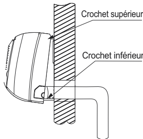
Fig. 15 — Installation du module intérieur
