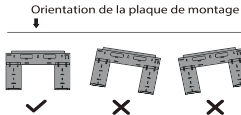
Fig. 9 — Orientation de la plaque de montage
