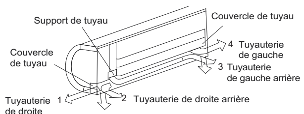
Fig. 11 — Emplacements des tuyauteries
