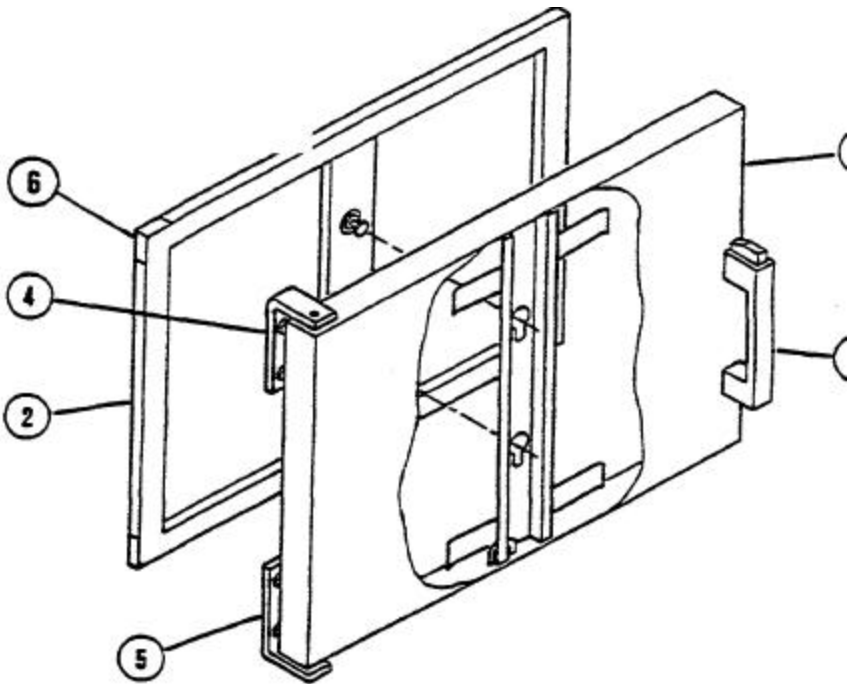
Fig. 27 DOOR ASSEMBLY
