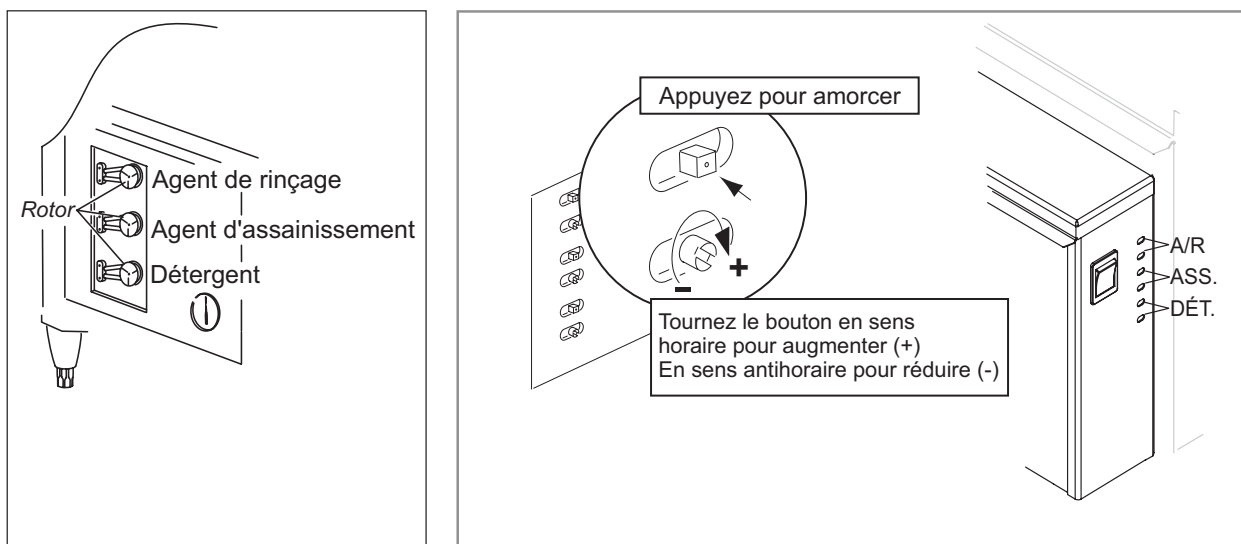
Commandes d'amorçage et de concentration des injecteurs de produits chimiques
